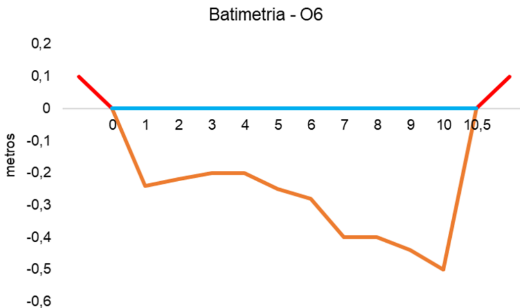
Figura V.2.3-26. Desenho esquemático da batimetria da estação O6 - Rio Sapucaia.
