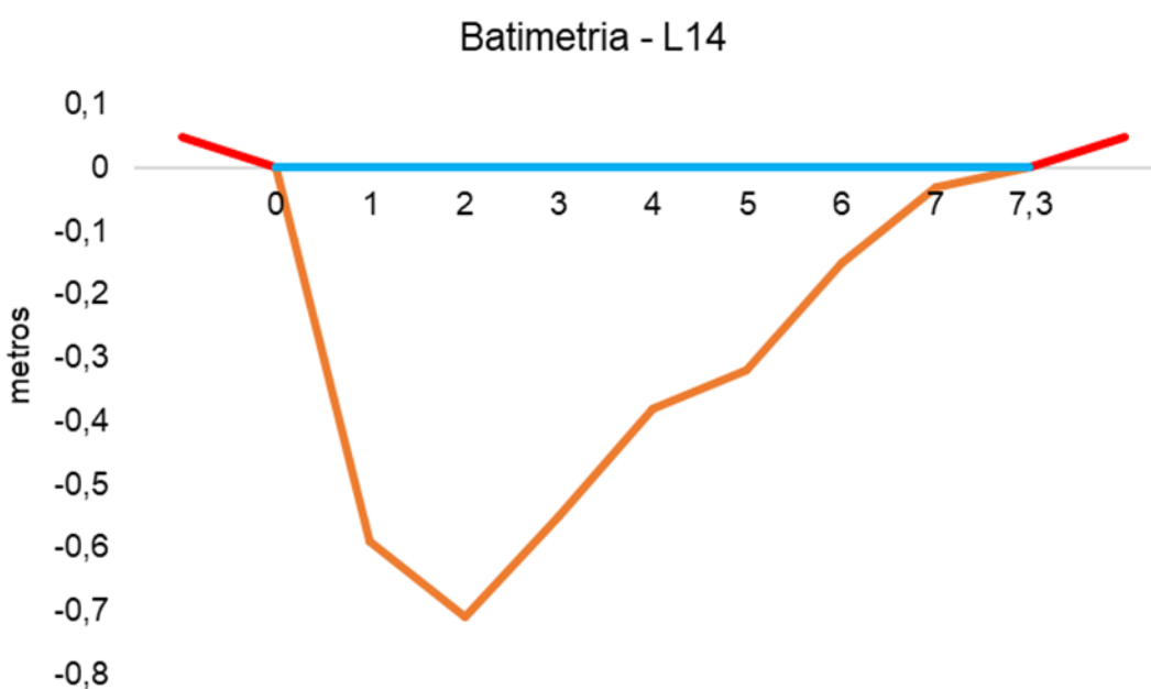
Figura V.2.3-15. Desenho esquemático da batimetria da estação L14 - Rio Duas Barras.
