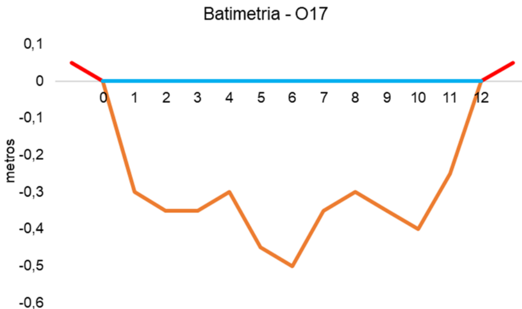
Figura V.2.3-36. Desenho esquemático da batimetria da estação O17 - Rio Sarapuí.
