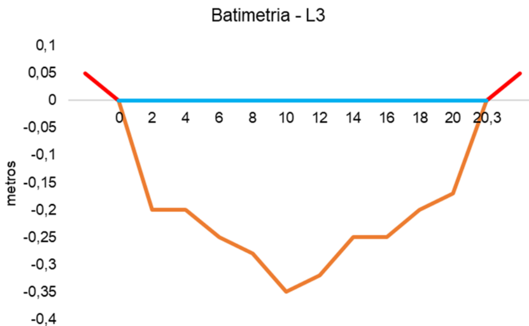
Figura V.2.3-7. Desenho esquemático da batimetria da estação L3 - Rio Macacu.
