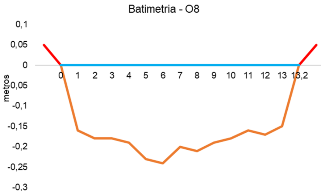
Figura V.2.3-28. Desenho esquemático da batimetria da estação O8 - Rio Tinguá.
