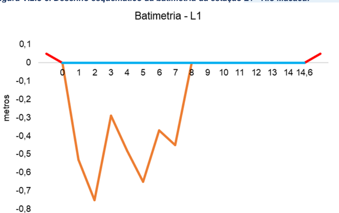
Figura V.2.3-5. Desenho esquemático da batimetria da estação L1 - Rio Macacu.
