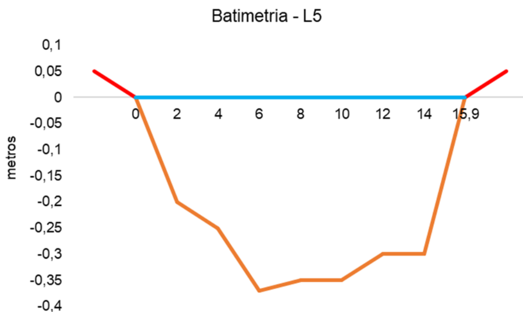
Figura V.2.3-9. Desenho esquemático da batimetria da estação L5 - Rio Macacu.
