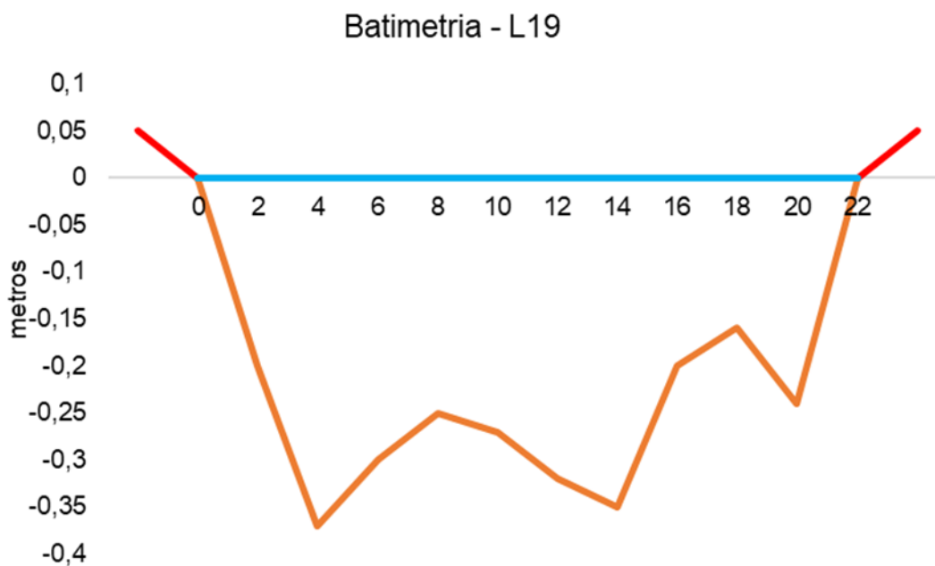
Figura V.2.3-19. Desenho esquemático da batimetria da estação L19 - Rio Guapiaçu.
