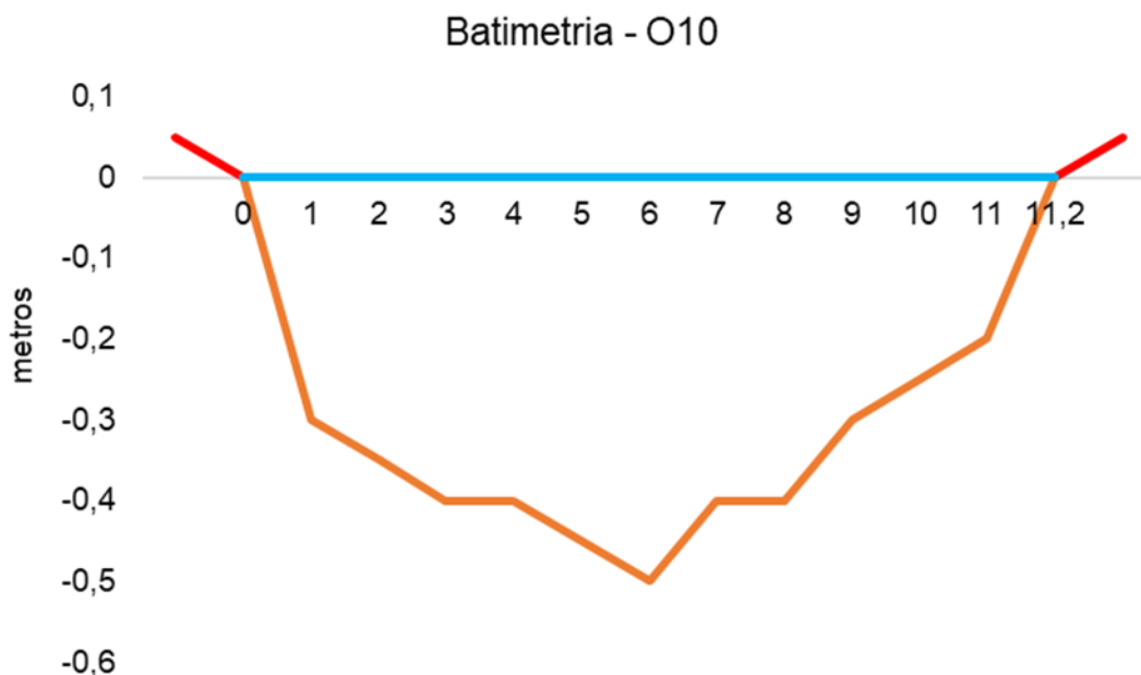
Figura V.2.3-30. Desenho esquemático da batimetria da estação O10 - Rio Iguaçu.
