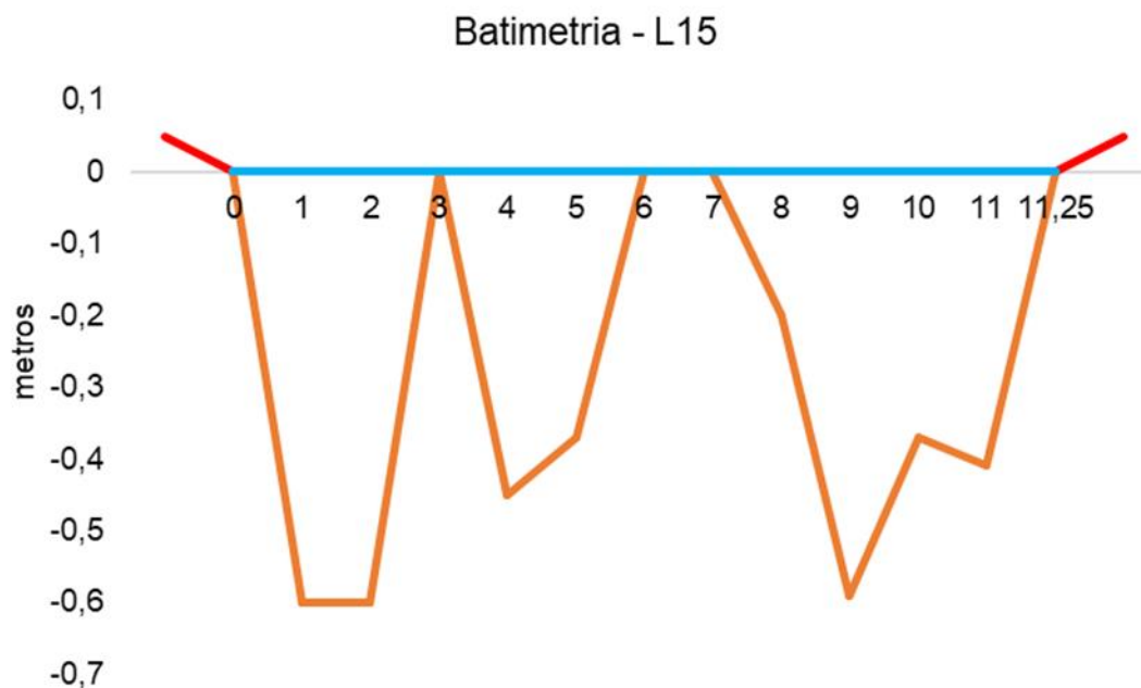
Figura V.2.3-16. Desenho esquemático da batimetria da estação L15 - Rio Guapiaçu.
