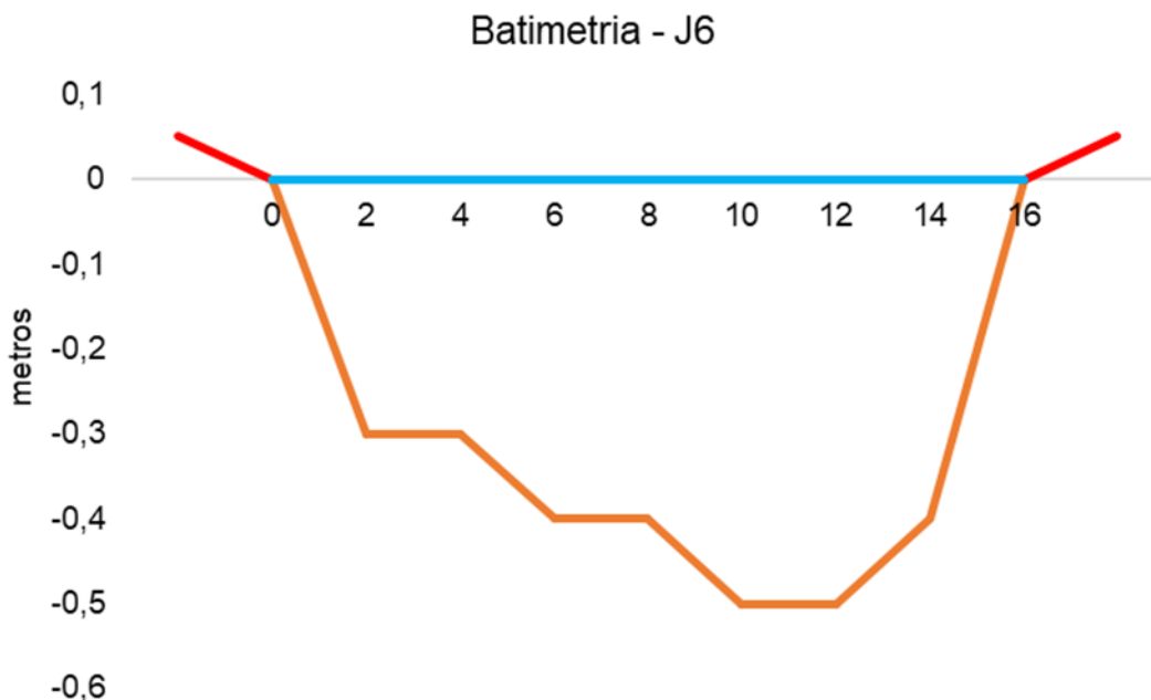
Figura V.2.3-2. Desenho esquemático da batimetria da estação J6 - Canal de Sernambetiba.
