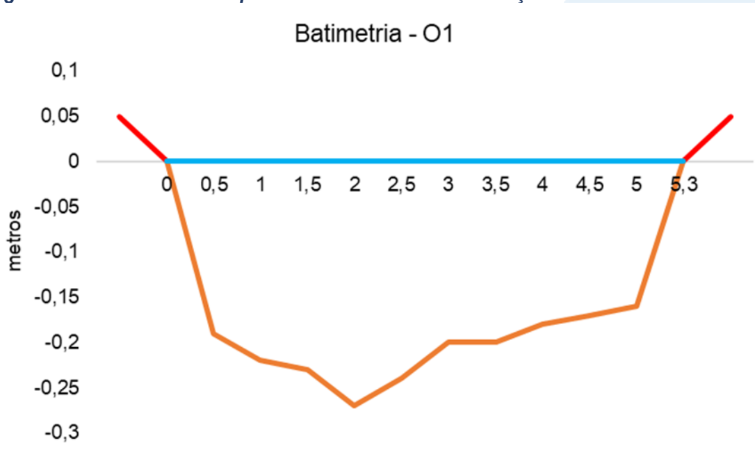
Figura V.2.3-23. Desenho esquemático da batimetria da estação O1 - Rio Saracuruna.
