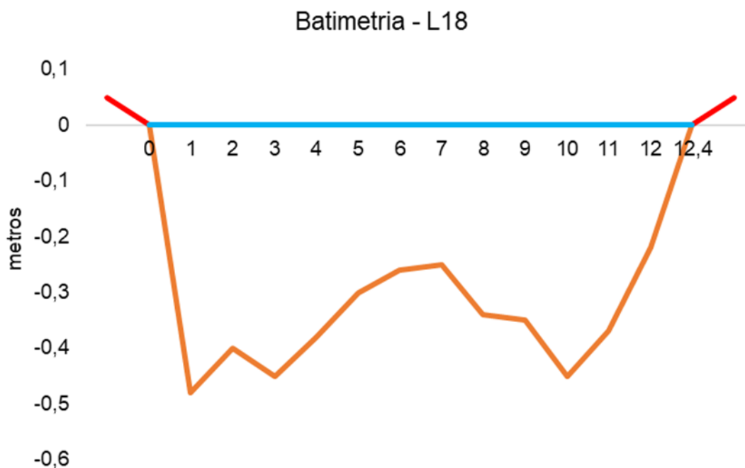
Figura V.2.3-18. Desenho esquemático da batimetria da estação L18 - Rio Guapiaçu.
