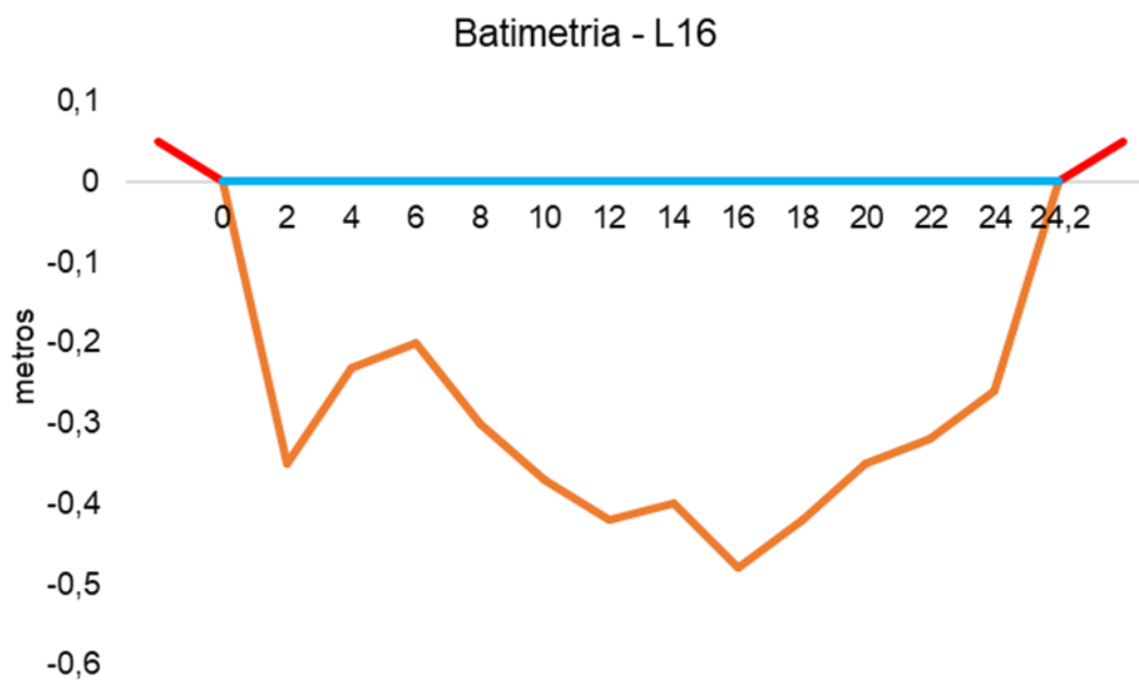
Figura V.2.3-17. Desenho esquemático da batimetria da estação L16 - Rio Guapiaçu.
