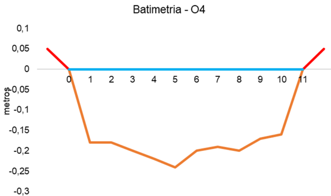
Figura V.2.3-25. Desenho esquemático da batimetria da estação O4 - Rio Sapucaia.
