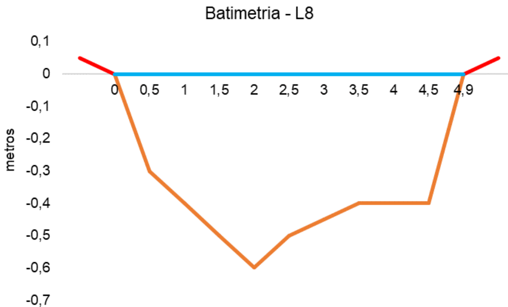
Figura V.2.3-13. Desenho esquemático da batimetria da estação L8 - Papucainha.
