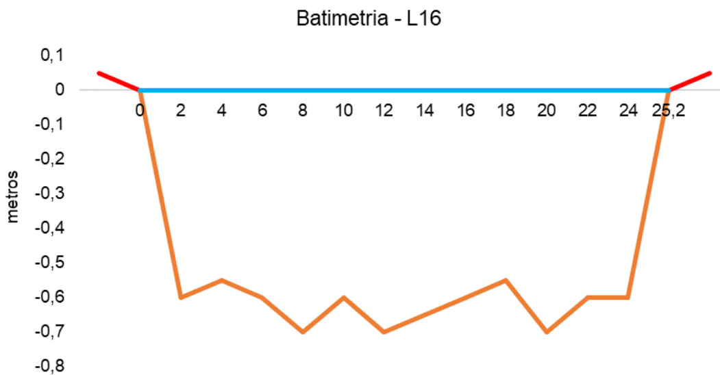
Figura V.2.3-19. Desenho esquemático da batimetria da estação L16 - Rio Guapiaçu.
