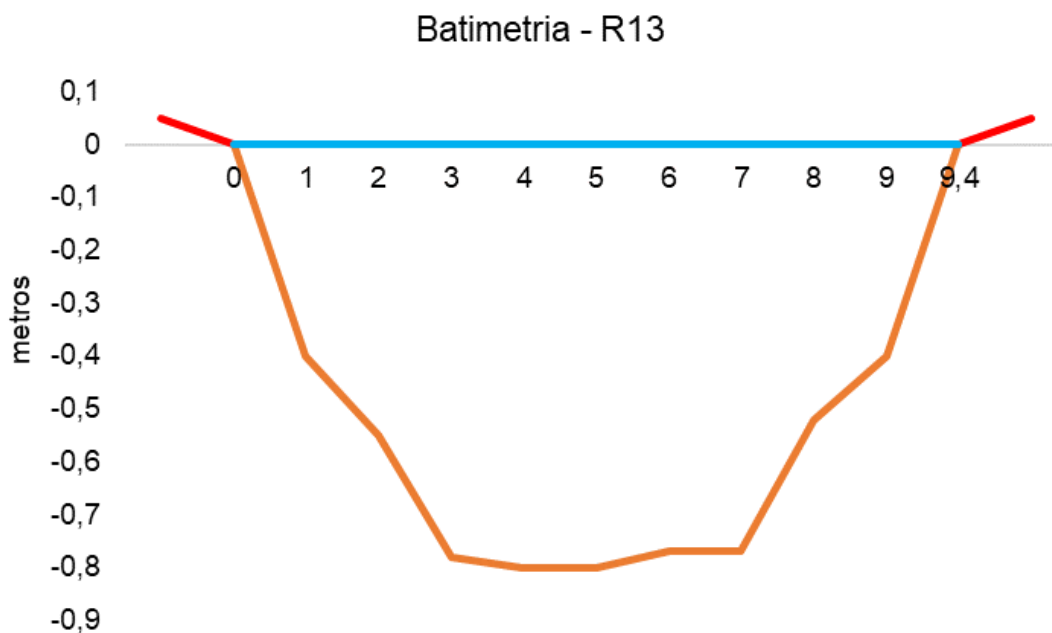
Figura V.2.3-6. Desenho esquemático da batimetria da estação R13 - Rio Rainha.
