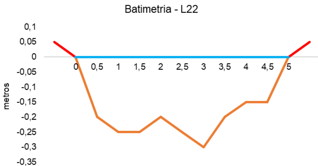
Figura V.2.3-23. Desenho esquemático da batimetria da estação L22 - Afluente do Rio Caceribu.
