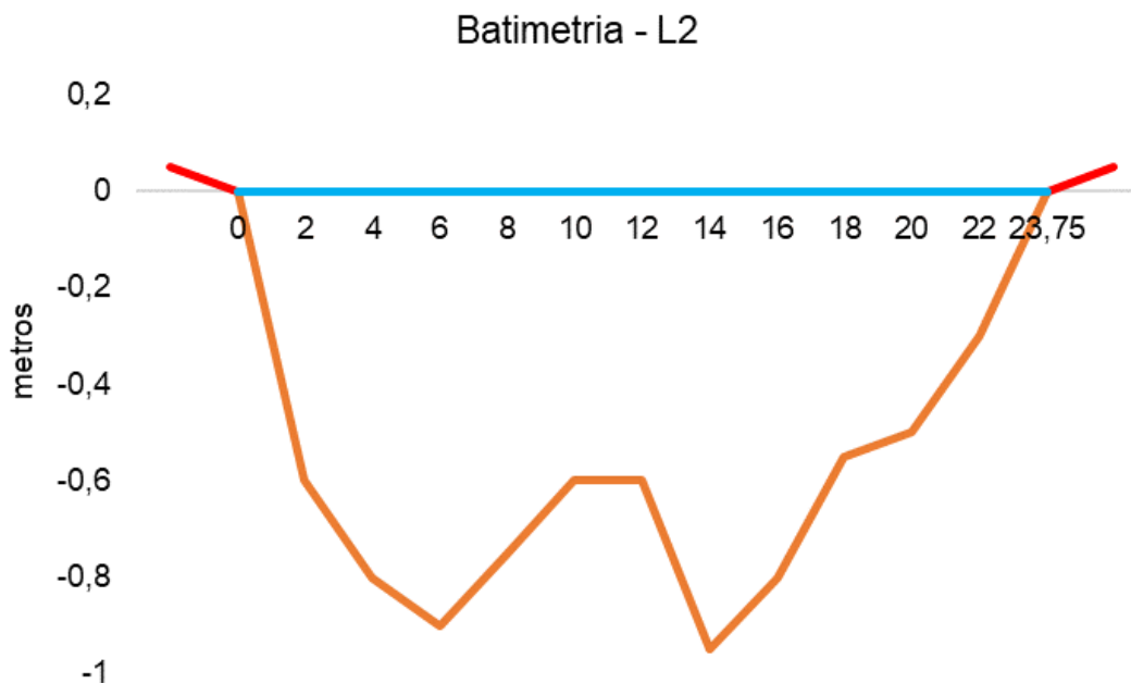
Figura V.2.3-8. Desenho esquemático da batimetria da estação L2 - Rio Macacu.
