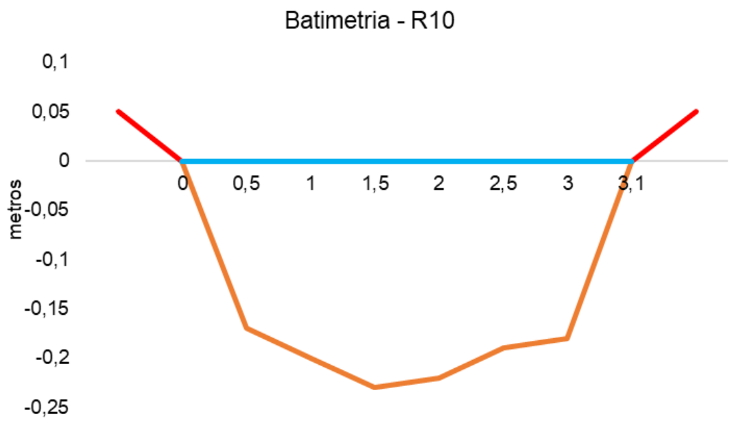
Figura V.2.3-5. Desenho esquemático da batimetria da estação R10 - Rio Rainha.
