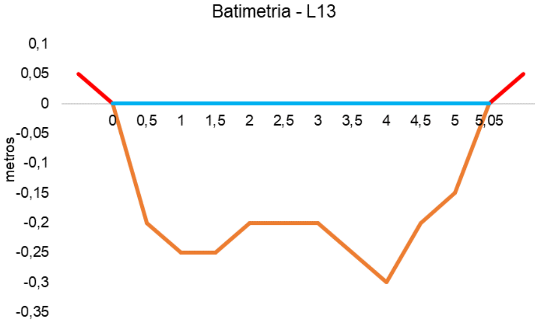
Figura V.2.3-16. Desenho esquemático da batimetria da estação L13 - Rio Itaperi.
