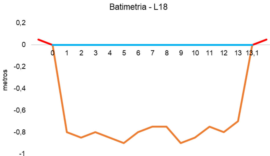
Figura V.2.3-20. Desenho esquemático da batimetria da estação L18 - Rio Guapiaçu.
