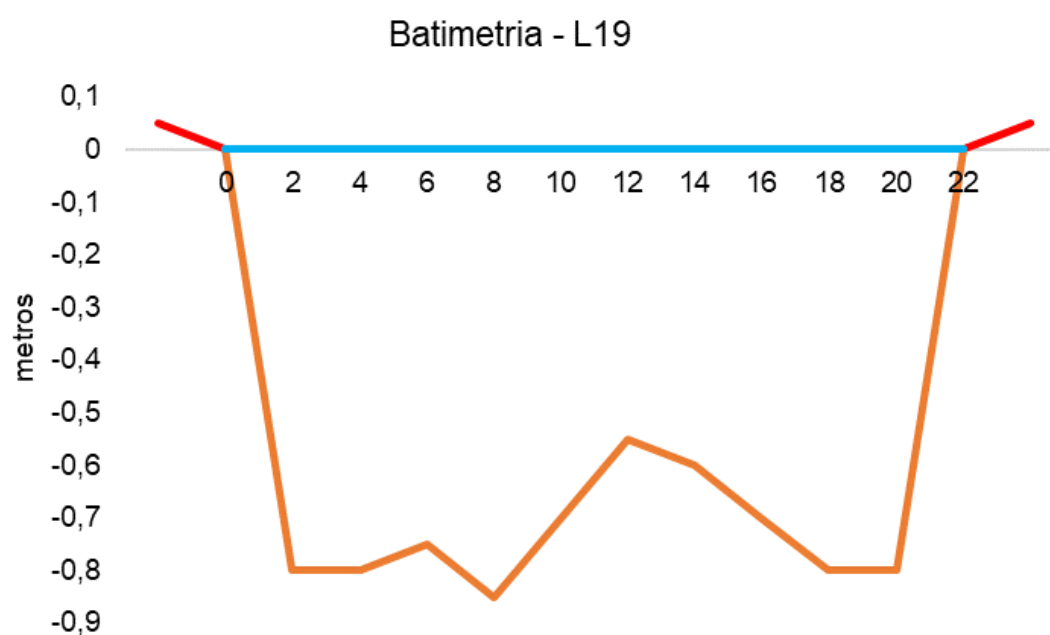
Figura V.2.3-21. Desenho esquemático da batimetria da estação L19 - Rio Guapiaçu.
