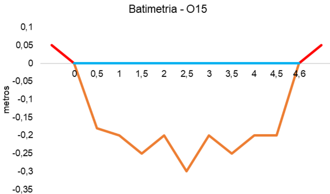
Figura V.2.3-37. Desenho esquemático da batimetria da estação O15 - Rio Sarapuí.
