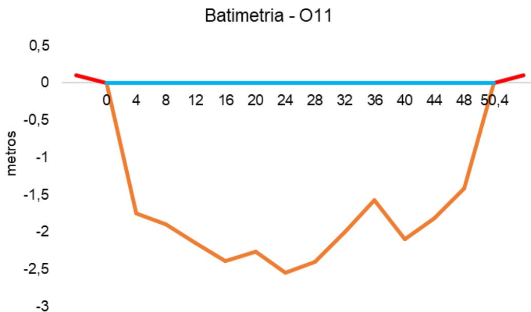
Figura V.2.3-33. Desenho esquemático da batimetria da estação O11 - Rio Iguaçu.
