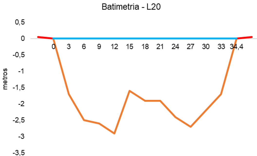
Figura V.2.3-22. Desenho esquemático da batimetria da estação L20 - Rio Guapiaçu.
