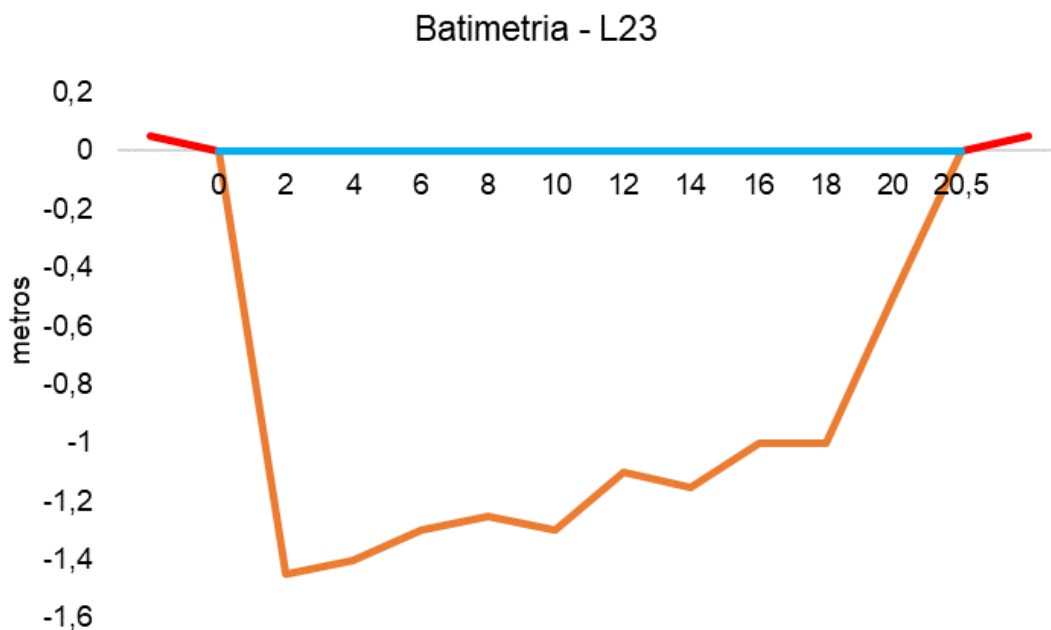
Figura V.2.3-24. Desenho esquemático da batimetria da estação L22 - Afluente do Rio Caceribu.
