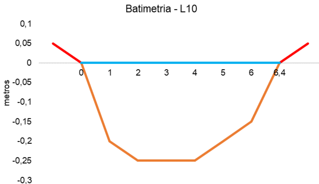
Figura V.2.3-14. Desenho esquemático da batimetria da estação L10 - Rio Rabelo.
