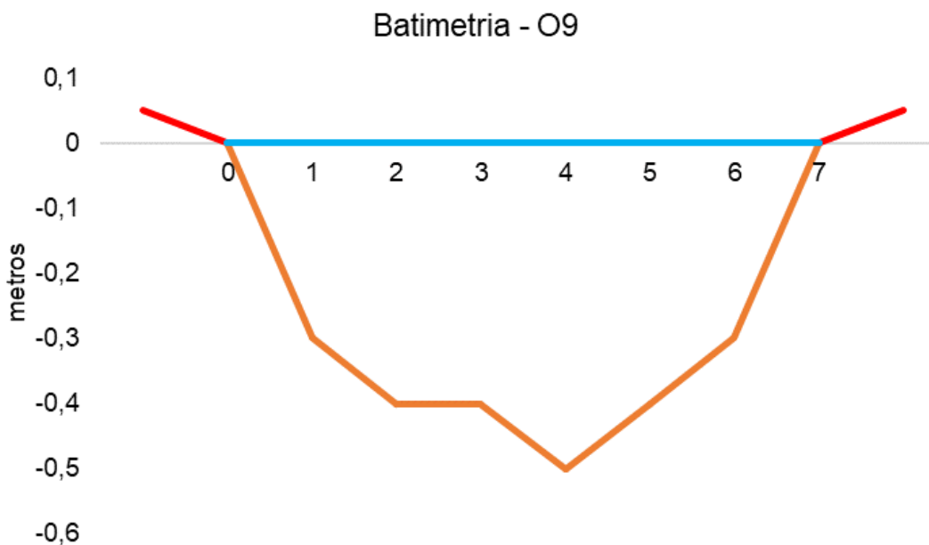
Figura V.2.3-31. Desenho esquemático da batimetria da estação O9 - Rio Iguaçu.
