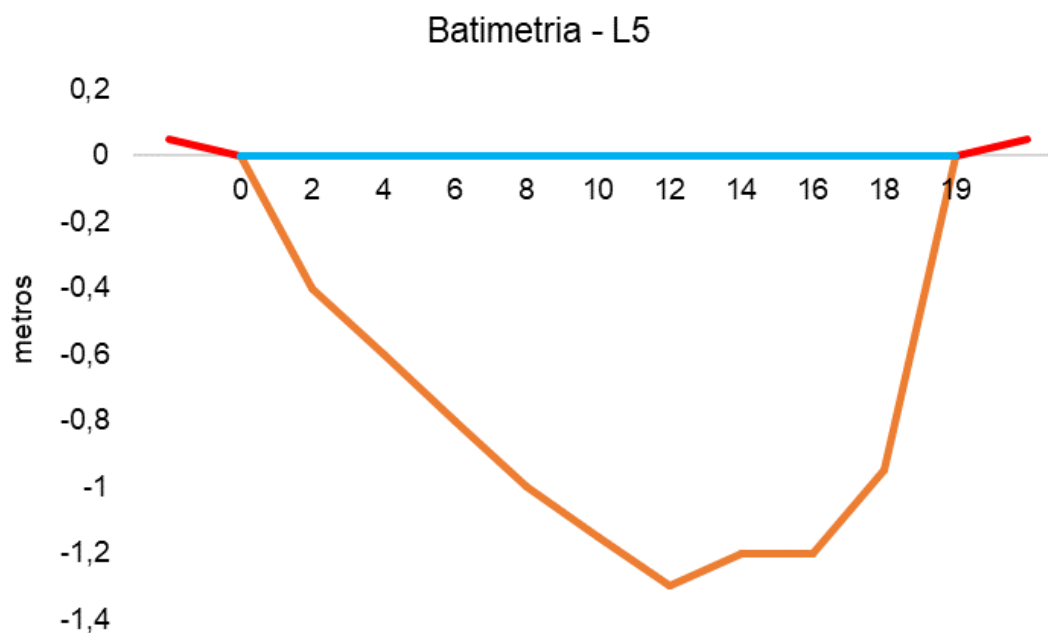
Figura V.2.3-11. Desenho esquemático da batimetria da estação L5 - Rio Macacu.
