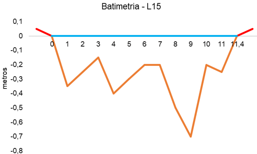
Figura V.2.3-18. Desenho esquemático da batimetria da estação L15 - Rio Guapiaçu.
