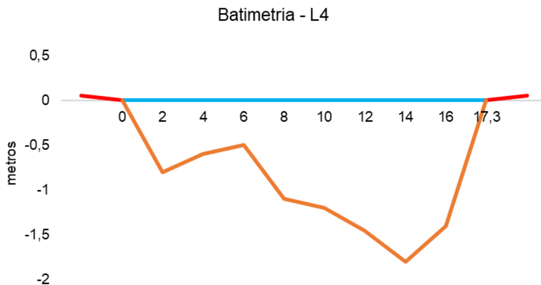
Figura V.2.3-10. Desenho esquemático da batimetria da estação L4 - Rio Macacu.
