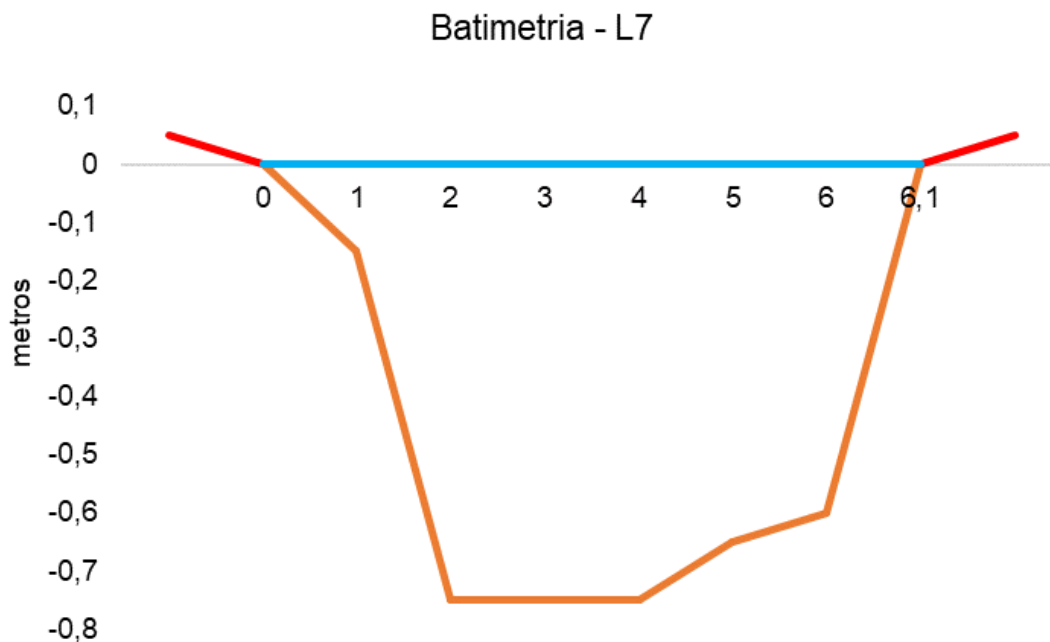
Figura V.2.3-12. Desenho esquemático da batimetria da estação L7 - Rio Cassiano.
