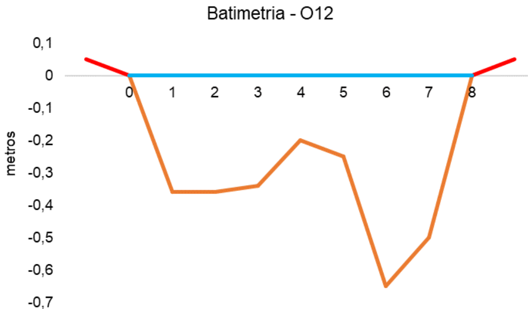
Figura V.2.3-34. Desenho esquemático da batimetria da estação O12 - Rio Botas.
