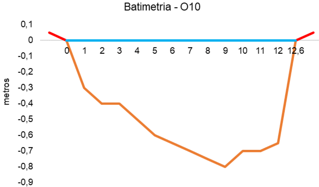
Figura V.2.3-32. Desenho esquemático da batimetria da estação O10 - Rio Iguaçu.
