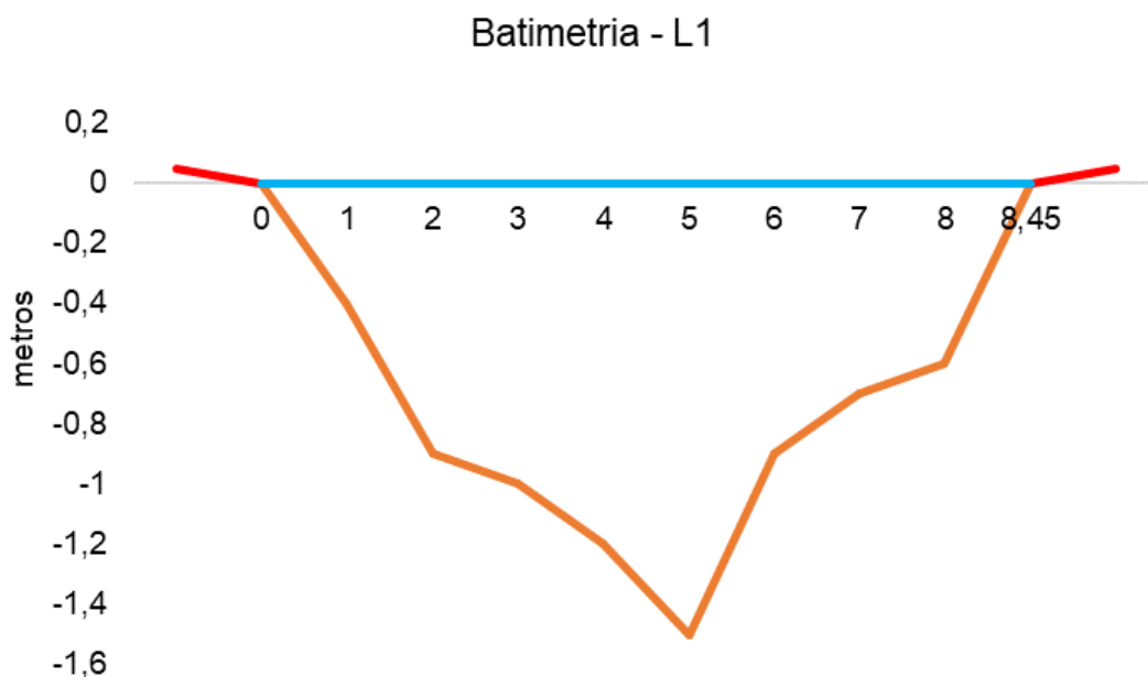
Figura V.2.3-7. Desenho esquemático da batimetria da estação L1 - Rio Macacu.
