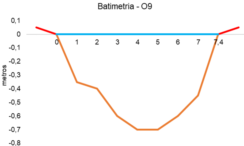
Figura V.2.3-31. Desenho esquemático da batimetria da estação O9 - Rio Iguçu.
