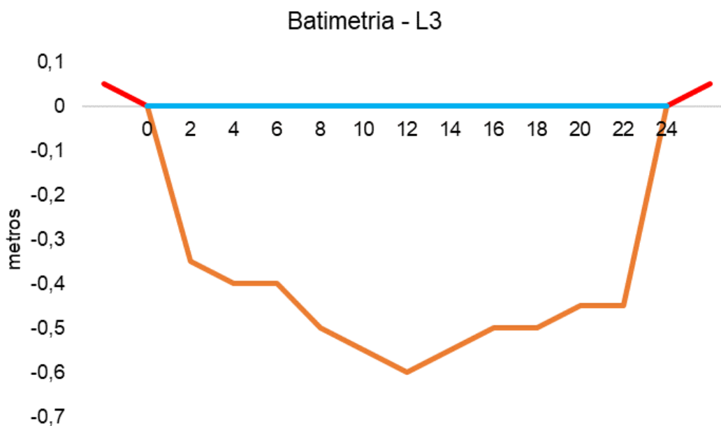
Figura V.2.3-9. Desenho esquemático da batimetria da estação L3 - Rio Macacu.
