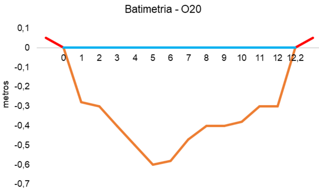
Figura V.2.3-39. Desenho esquemático da batimetria da estação O20 - Rio Acari.
