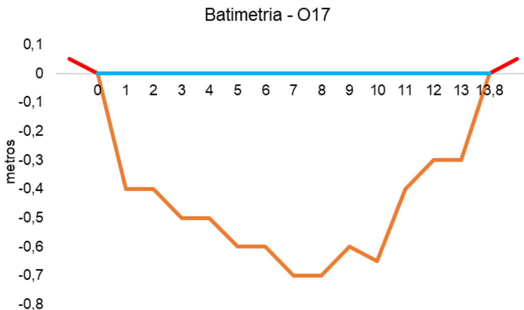
Figura V.2.3-38. Desenho esquemático da batimetria da estação O17 - Rio Sarapuí.
