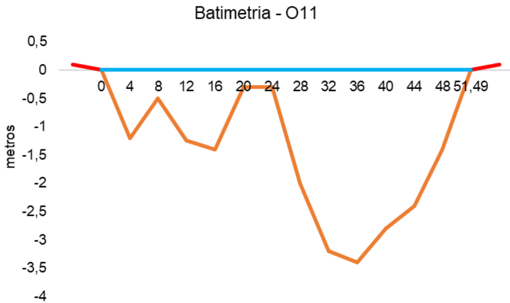
Figura V.2.3-33. Desenho esquemático da batimetria da estação O11 - Rio Iguaçu.
