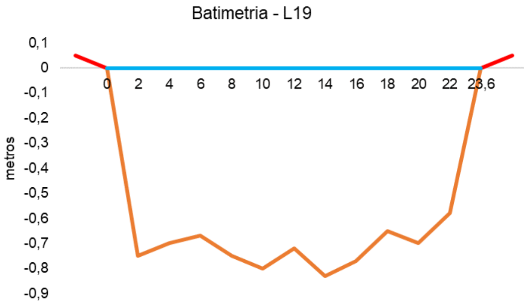
Figura V.2.3-21. Desenho esquemático da batimetria da estação L19 - Rio Guapiaçu.
