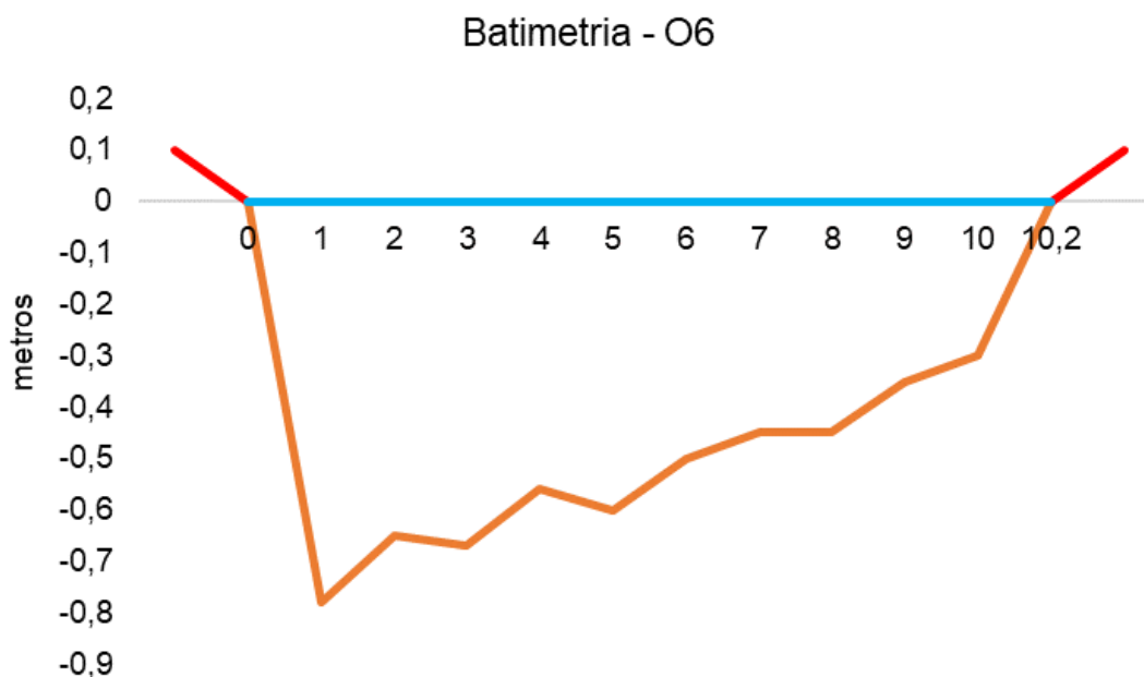
Figura V.2.3-27. Desenho esquemático da batimetria da estação O6 - Rio Sapucaia.
