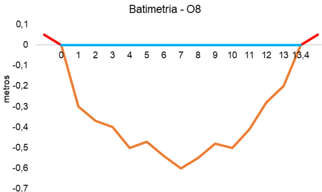
Figura V.2.3-29. Desenho esquemático da batimetria da estação O8 - Rio Tinguá.
