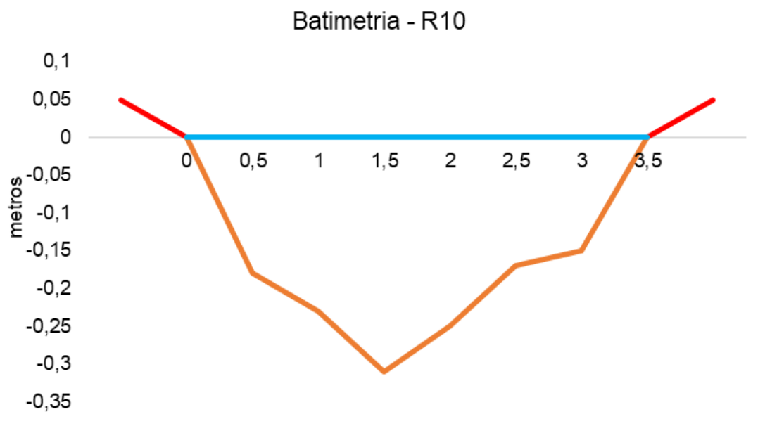
Figura V.2.3-4. Desenho esquemático da batimetria da estação R10 - Rio Rainha.
