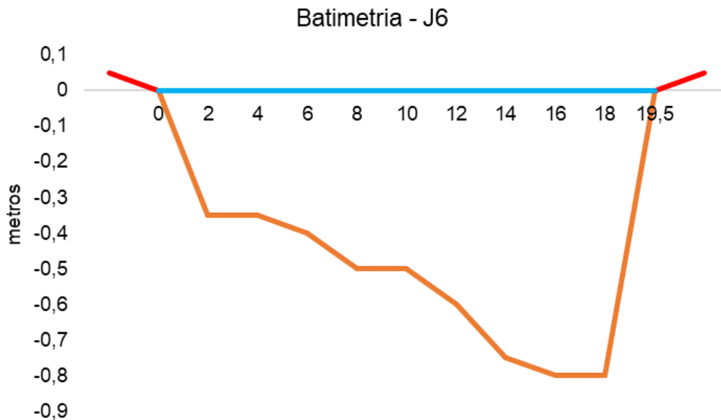
Figura V.2.3-2. Desenho esquemático da batimetria da estação J6 - Canal de Sernambetiba.
