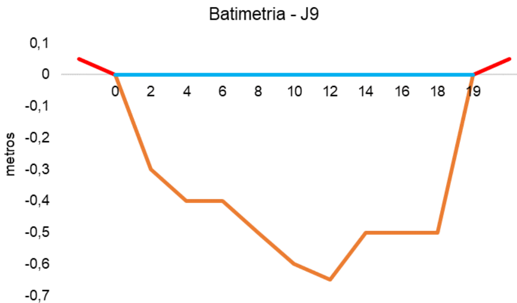
Figura V.2.3-3. Desenho esquemático da batimetria da estação J9 - Canal das Taxas.
