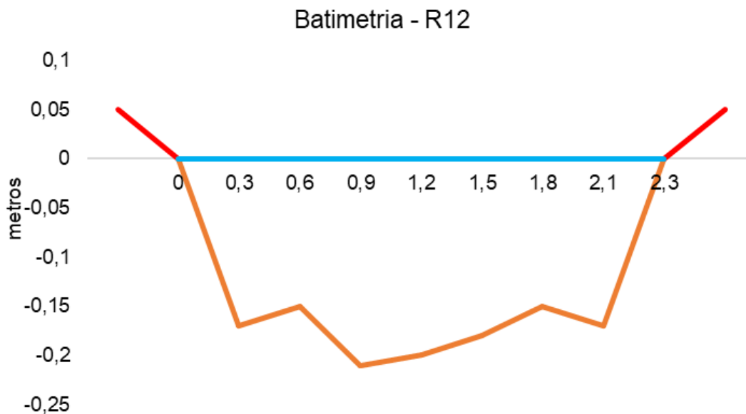
Figura V.2.3-5. Desenho esquemático da batimetria da estação R12 - Rio Rainha.
