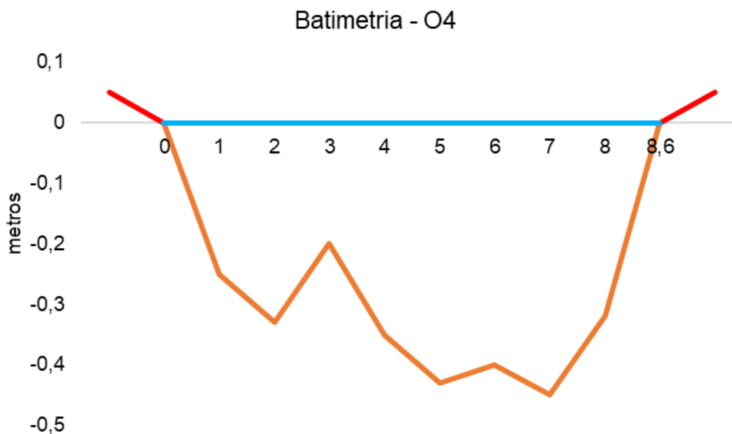
Figura V.2.3-26. Desenho esquemático da batimetria da estação O4 - Rio Sapucaia.
