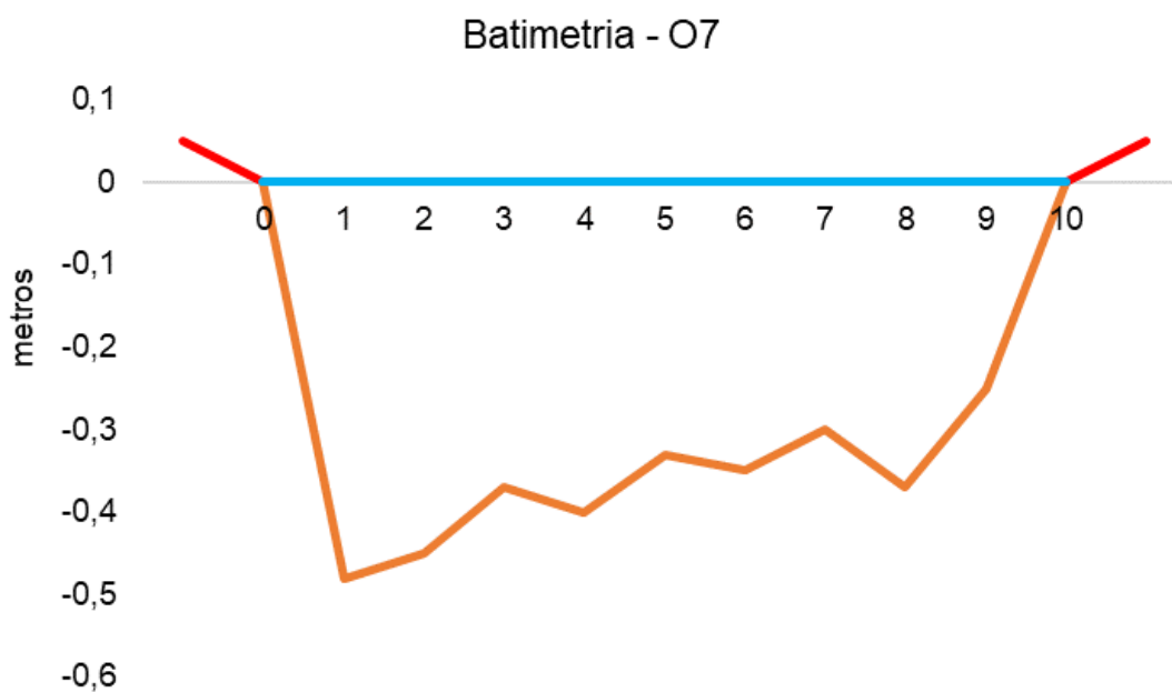
Figura V.2.3-28. Desenho esquemático da batimetria da estação O7 - Rio Tinguá.
