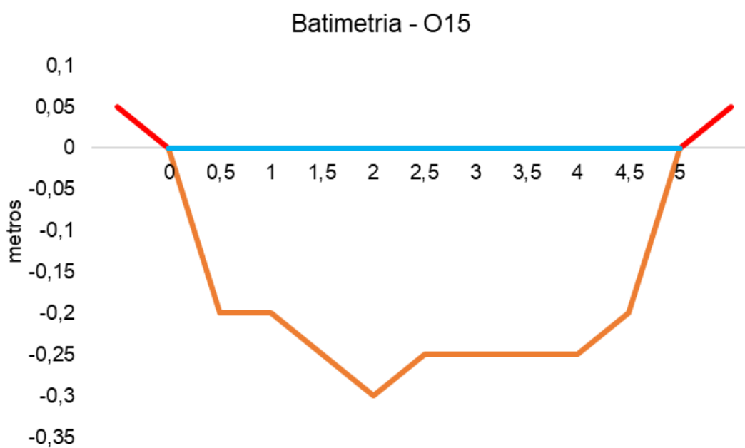
Figura V.2.3-36. Desenho esquemático da batimetria da estação O15 - Rio Sarapuí.
