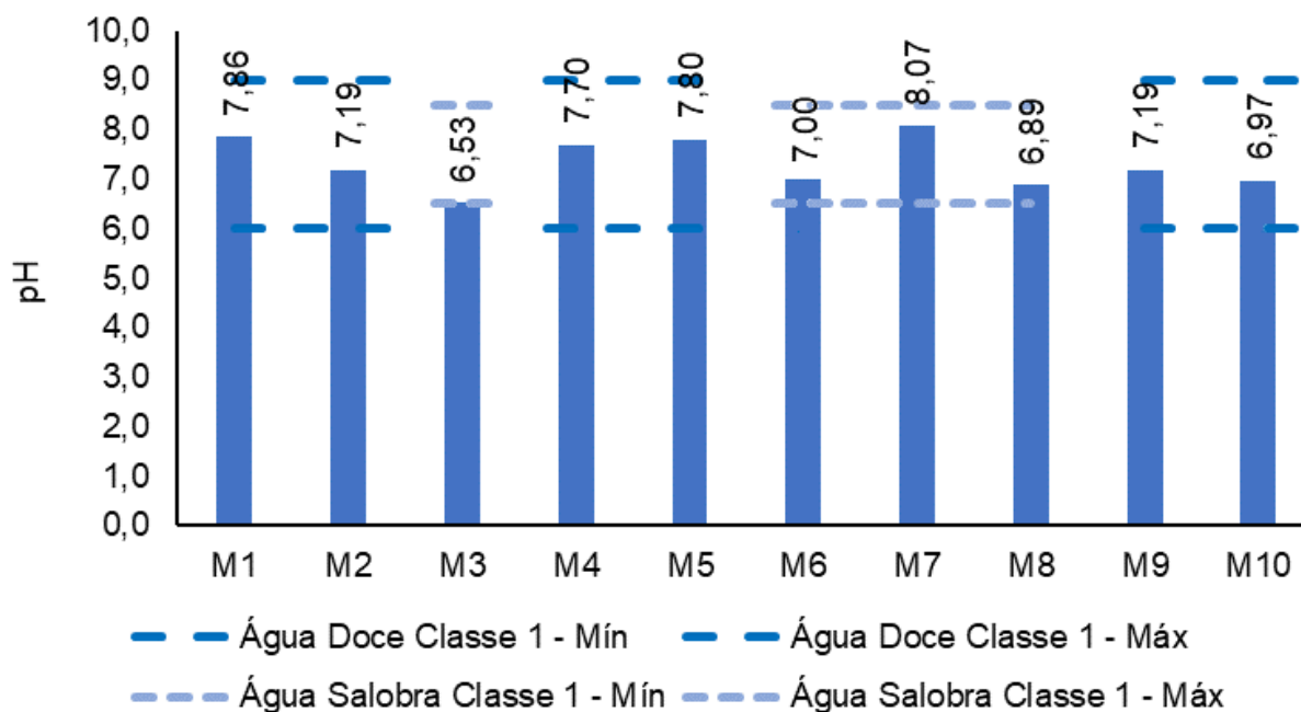
Figura V.2.1-6. Distribuição de pH na Sub-bacia do Sistema Lagunar de Maricá durante a campanha de novembro de 2023.
