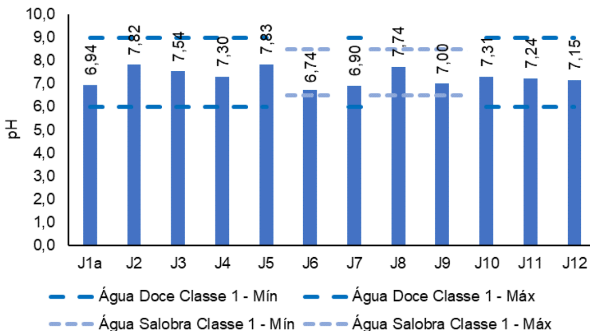
Figura V.2.1-18. Distribuição de pH na Sub-bacia do Sistema Lagunar de Jacarepaguá durante a campanha de novembro de 2023.
