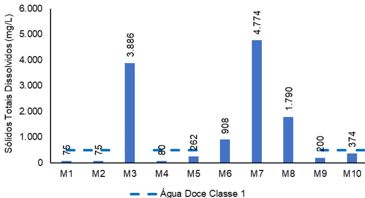
Figura V.2.1-11. Distribuição de STD na Sub-bacia do Sistema Lagunar de Maricá durante a campanha de novembro de 2023.
