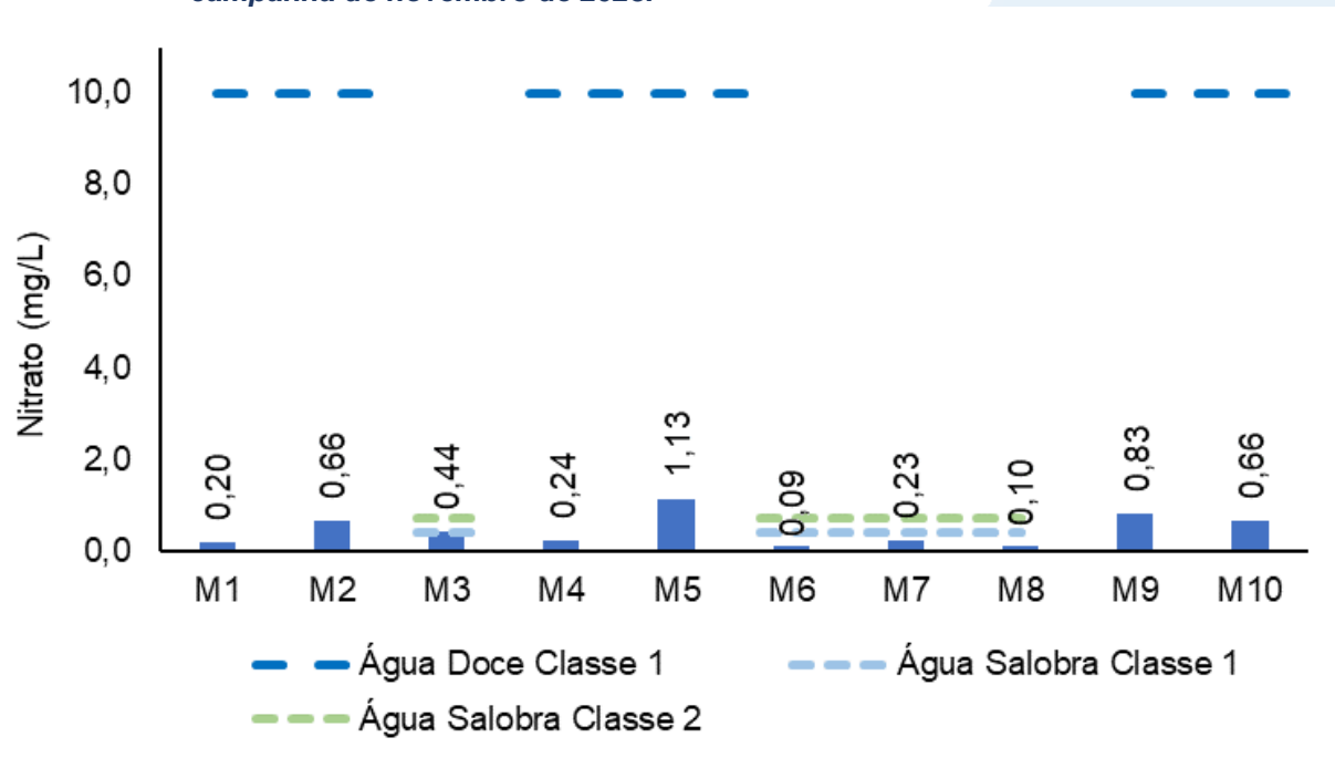
Figura V.2.1-9. Distribuição de nitrato na Sub-bacia do Sistema Lagunar de Maricá durante a campanha de novembro de 2023.
