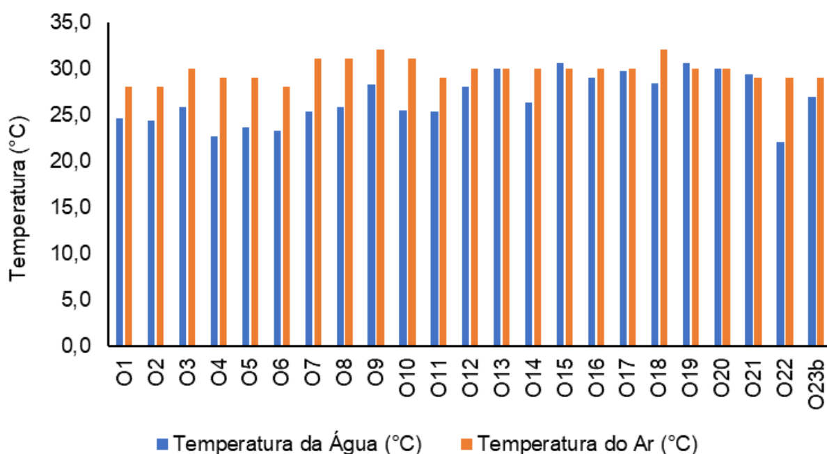
Figura V.2.1-62. Distribuição de temperatura do ar e da água na Sub-bacia Oeste durante a campanha de novembro de 2023.
