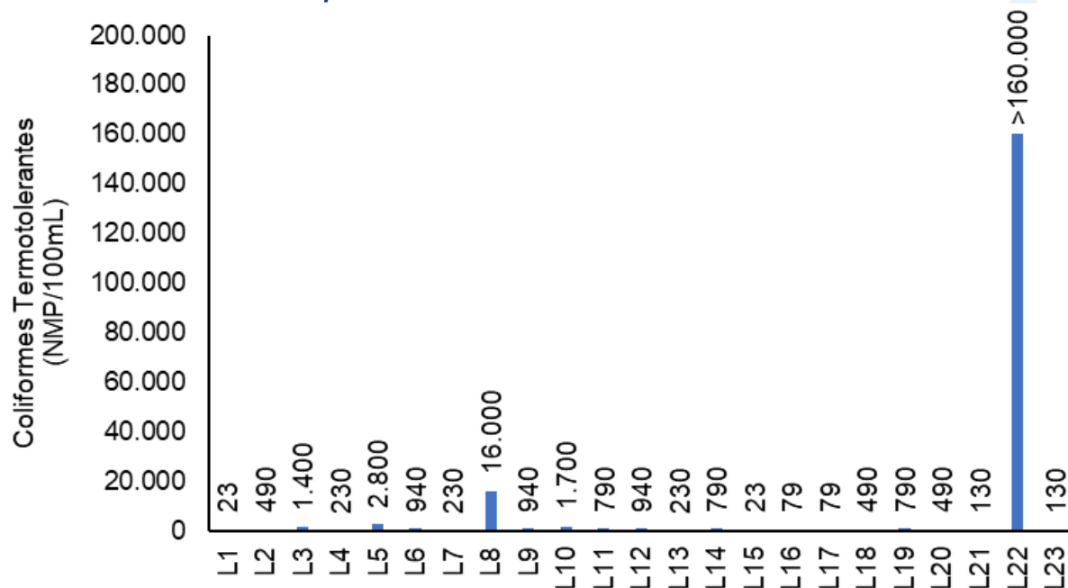
Figura V.2.1-60. Distribuição de coliformes termotolerantes na região Leste da Baía de Guanabara durante a campanha de novembro de 2023.
