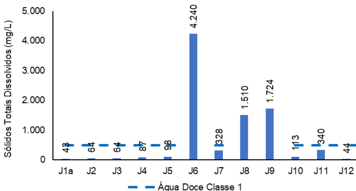
Figura V.2.1-23. Distribuição de STD na Sub-bacia do Sistema Lagunar de Jacarepaguá durante a campanha de novembro de 2023.
