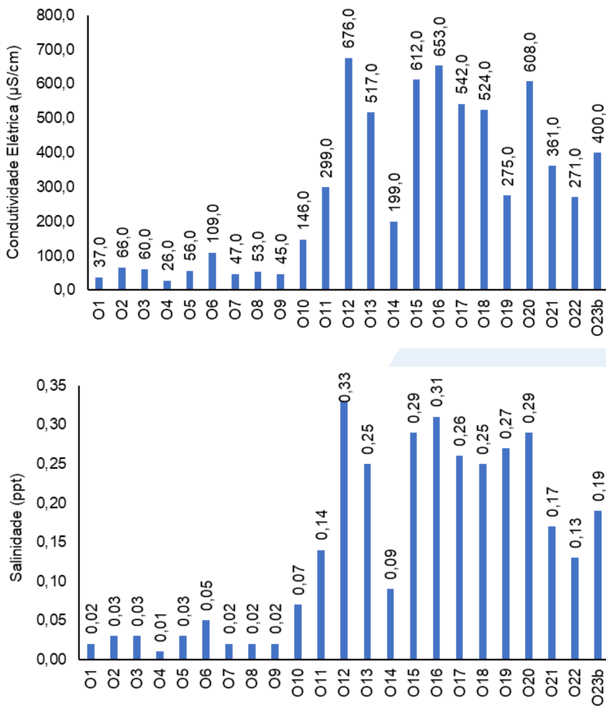
Figura V.2.1-61. Distribuição de condutividade e salinidade na Sub-bacia Oeste durante a campanha de novembro de 2023.
