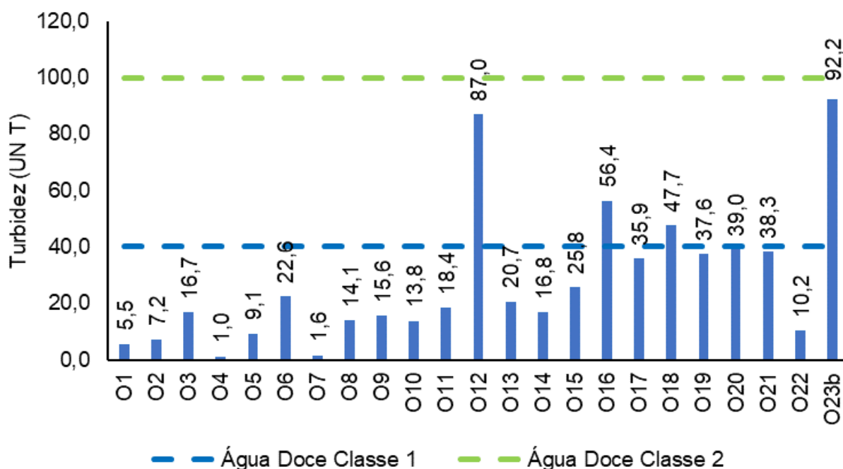
Figura V.2.1-67. Distribuição de turbidez na Sub-bacia Oeste durante a campanha de novembro de 2023.
