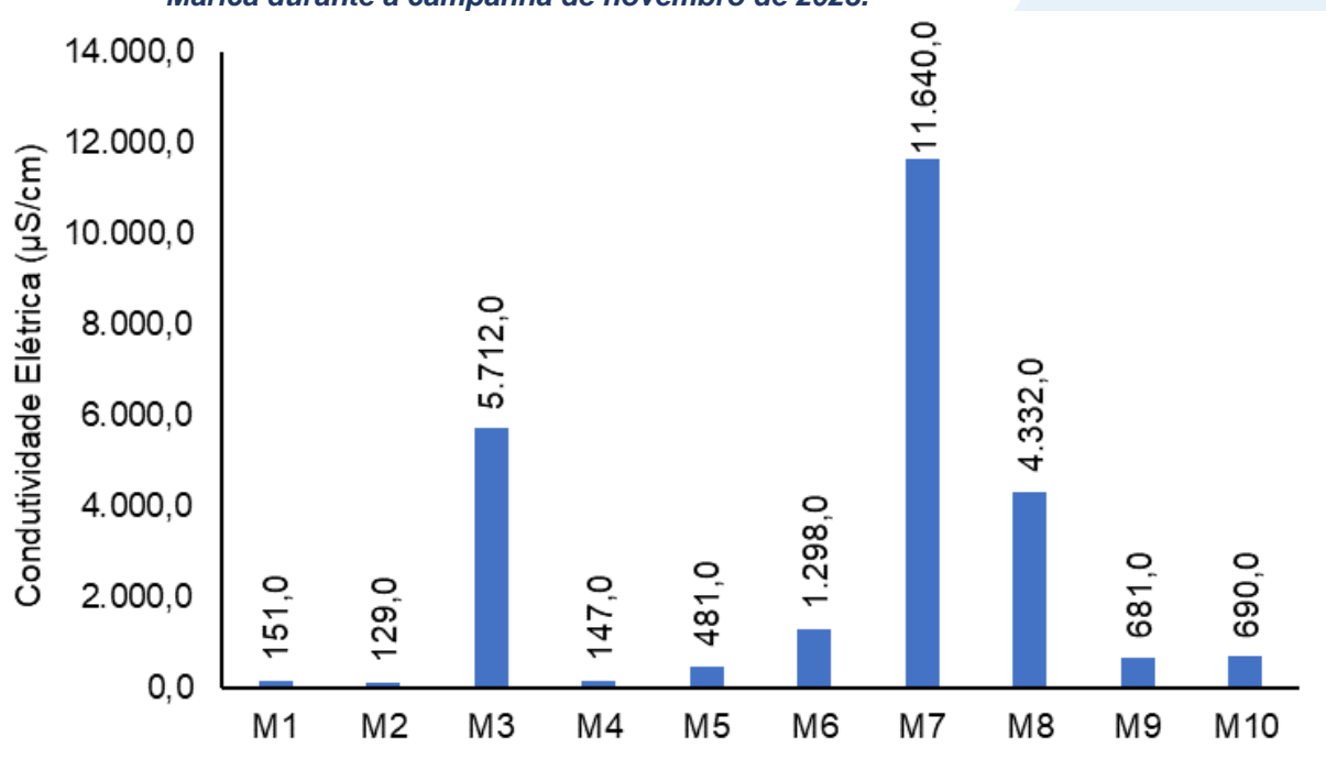
Figura V.2.1-1. Distribuição de condutividade e salinidade na Sub-bacia do Sistema Lagunar de Maricá durante a campanha de novembro de 2023.
