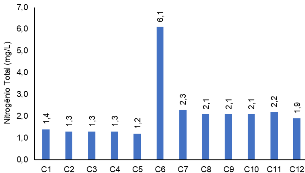
Figura V.2.1-46. Distribuição de nitrogênio total na Sub-bacia do Sistema Lagunar Itaipu-Piratininga durante a campanha de novembro de 2023.
