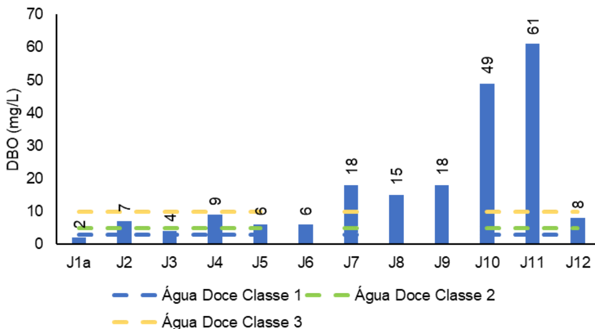
Figura V.2.1-16. Distribuição de DBO na Sub-bacia do Sistema Lagunar de Jacarepaguá durante a campanha de novembro de 2023.
