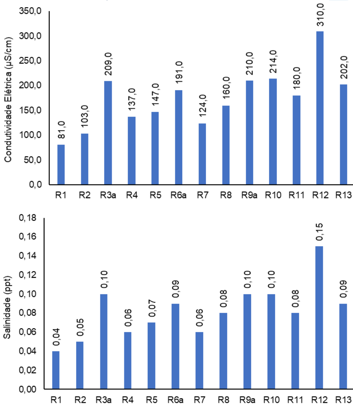
Figura V.2.1-25. Distribuição de condutividade e salinidade na Bacia da Lagoa Rodrigo de Freitas durante a campanha de novembro de 2023.
