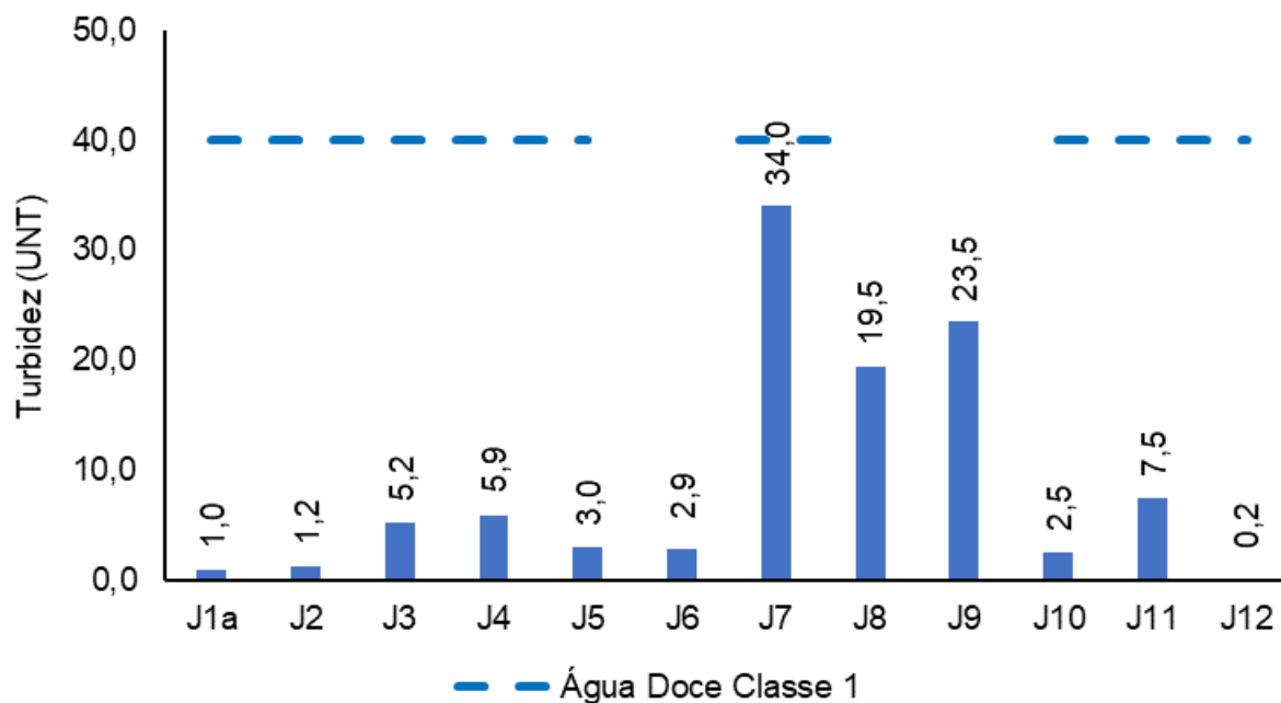
Figura V.2.1-19. Distribuição de turbidez na Sub-bacia do Sistema Lagunar de Jacarepaguá durante a campanha de novembro de 2023.
