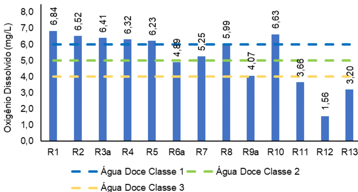
Figura V.2.1-27. Distribuição de oxigênio dissolvido na Bacia da Lagoa Rodrigo de Freitas durante a campanha de novembro de 2023.
