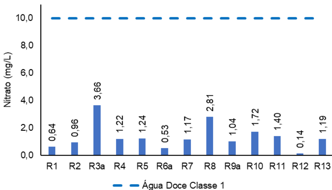
Figura V.2.1-33. Distribuição de nitrato na Bacia da Lagoa Rodrigo de Freitas durante a campanha de novembro de 2023.
