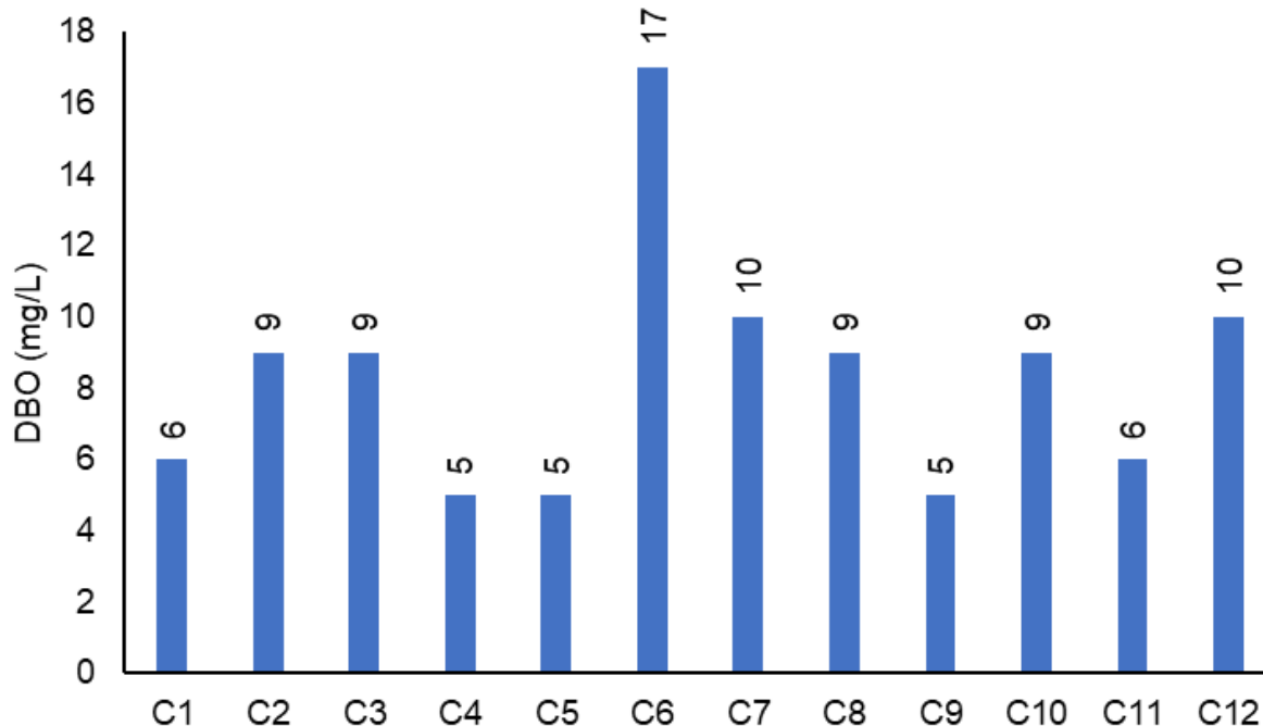
Figura V.2.1-40. Distribuição de DBO na Sub-bacia do Sistema Lagunar Itaipu-Piratininga durante a campanha de novembro de 2023.
