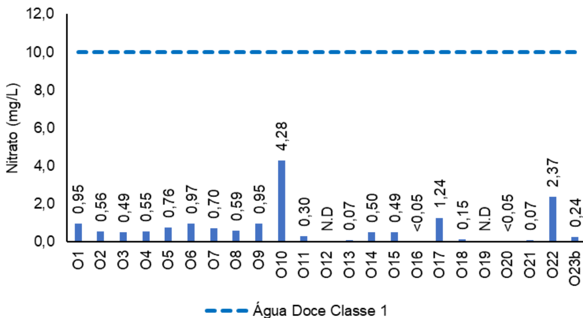
Figura V.2.1-69. Distribuição de nitrato na Sub-bacia Oeste durante a campanha de novembro de 2023.
