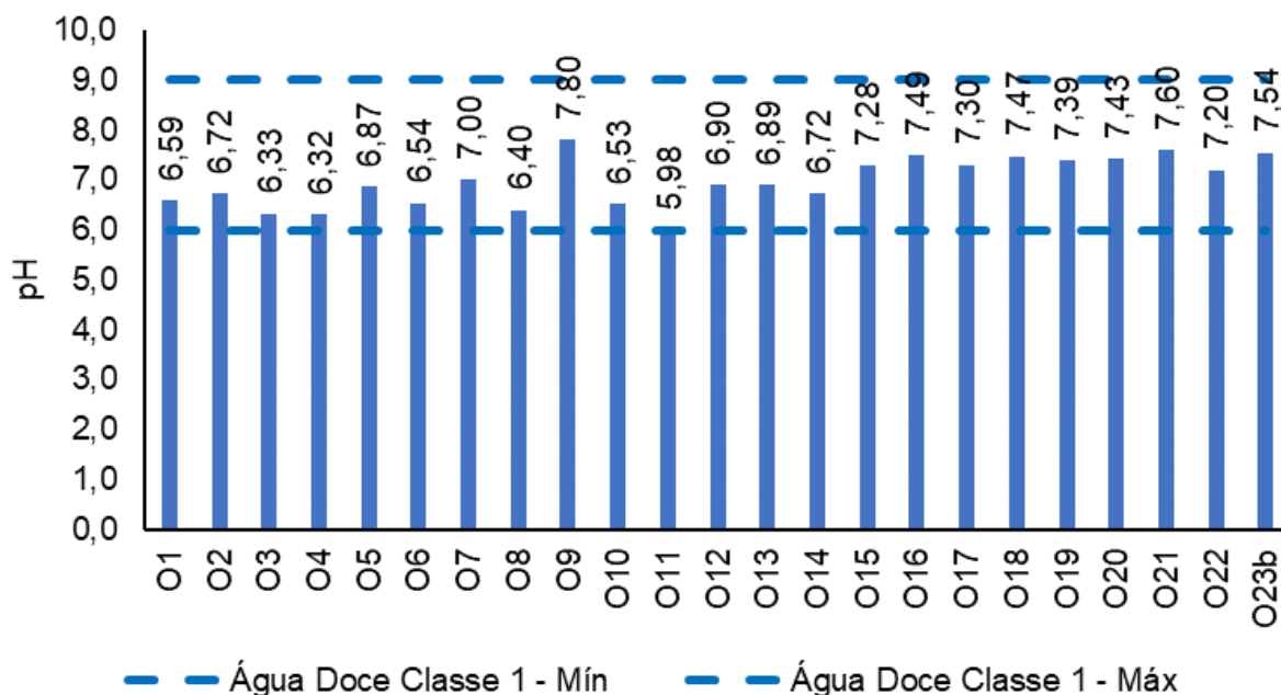
Figura V.2.1-66. Distribuição de pH na Sub-bacia Oeste durante a campanha de novembro de 2023.
