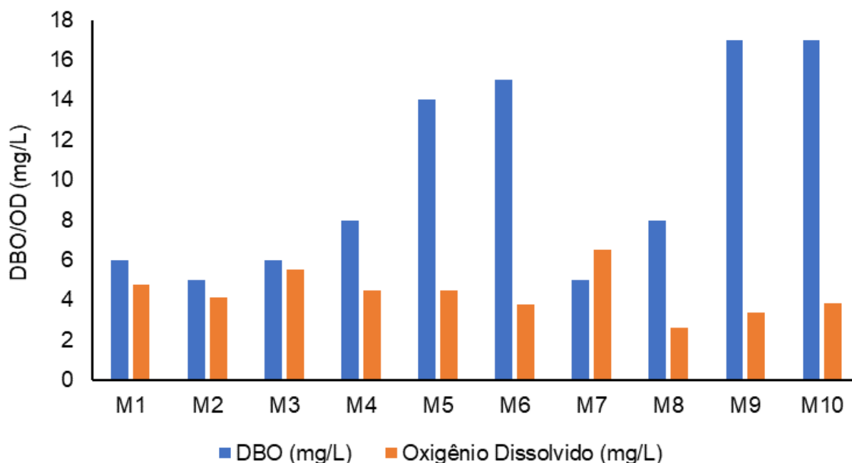
Figura V.2.1-5. Comparativo entre disponibilidade de oxigênio dissolvido e DBO na Sub-bacia do Sistema Lagunar de Maricá durante a campanha de novembro de 2023.
