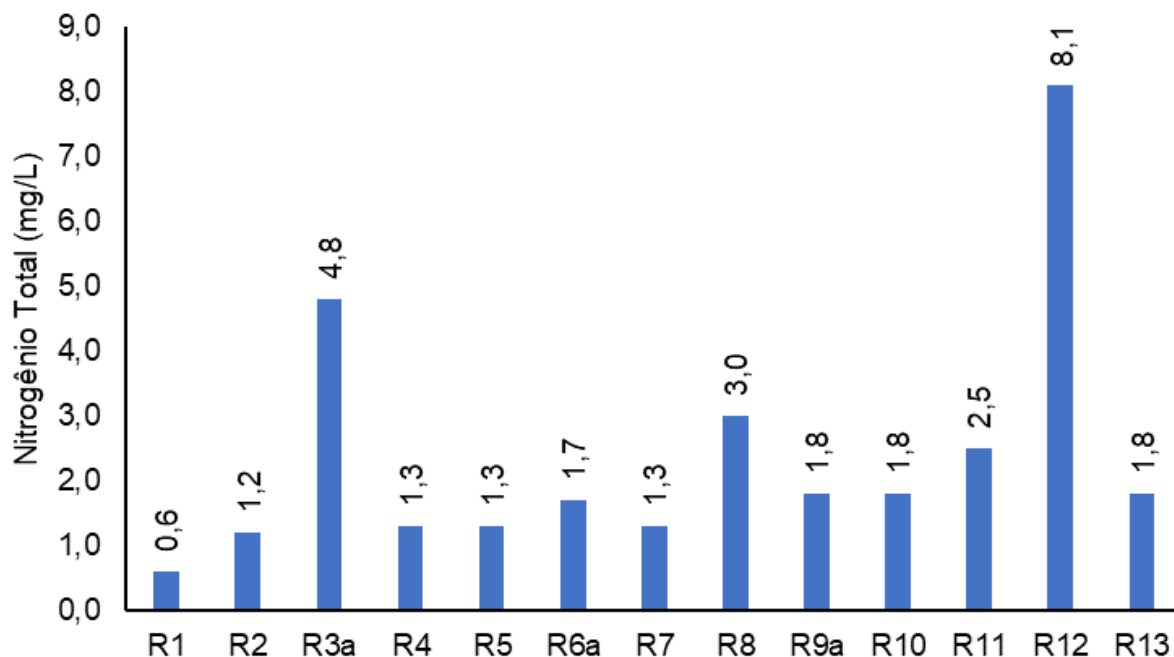
Figura V.2.1-34. Distribuição de nitrogênio total na Bacia da Lagoa Rodrigo de Freitas durante a campanha de novembro de 2023.
