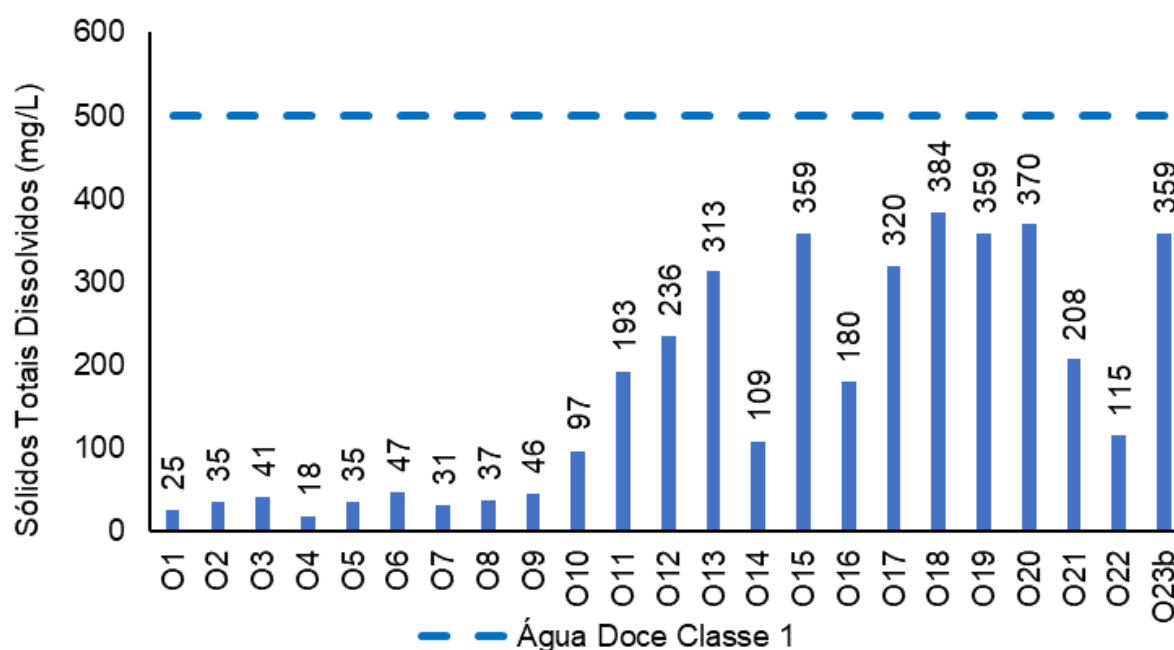
Figura V.2.1-71. Distribuição de STD na Sub-bacia Oeste durante a campanha de novembro de 2023.
