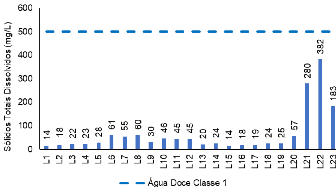
Figura V.2.1-59. Distribuição de STD na Sub-bacia Leste durante a campanha de novembro de 2023.
