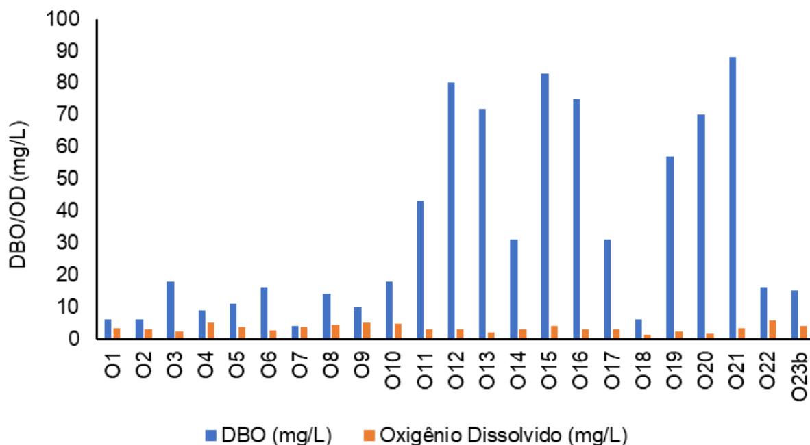
Figura V.2.1-65. Comparativo de OD e DBO na Sub-bacia Oeste durante a campanha de novembro de 2023.
