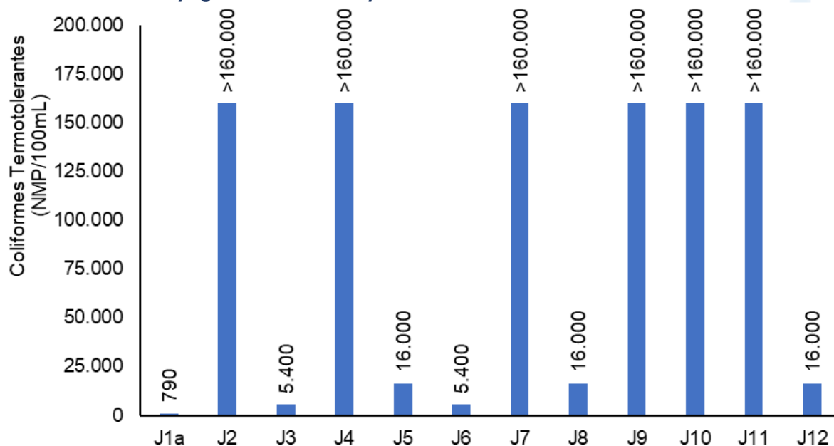
Figura V.2.1-24. Distribuição de coliformes termotolerantes na Sub-bacia do Sistema Lagunar de Jacarepaguá durante a campanha de novembro de 2023.
