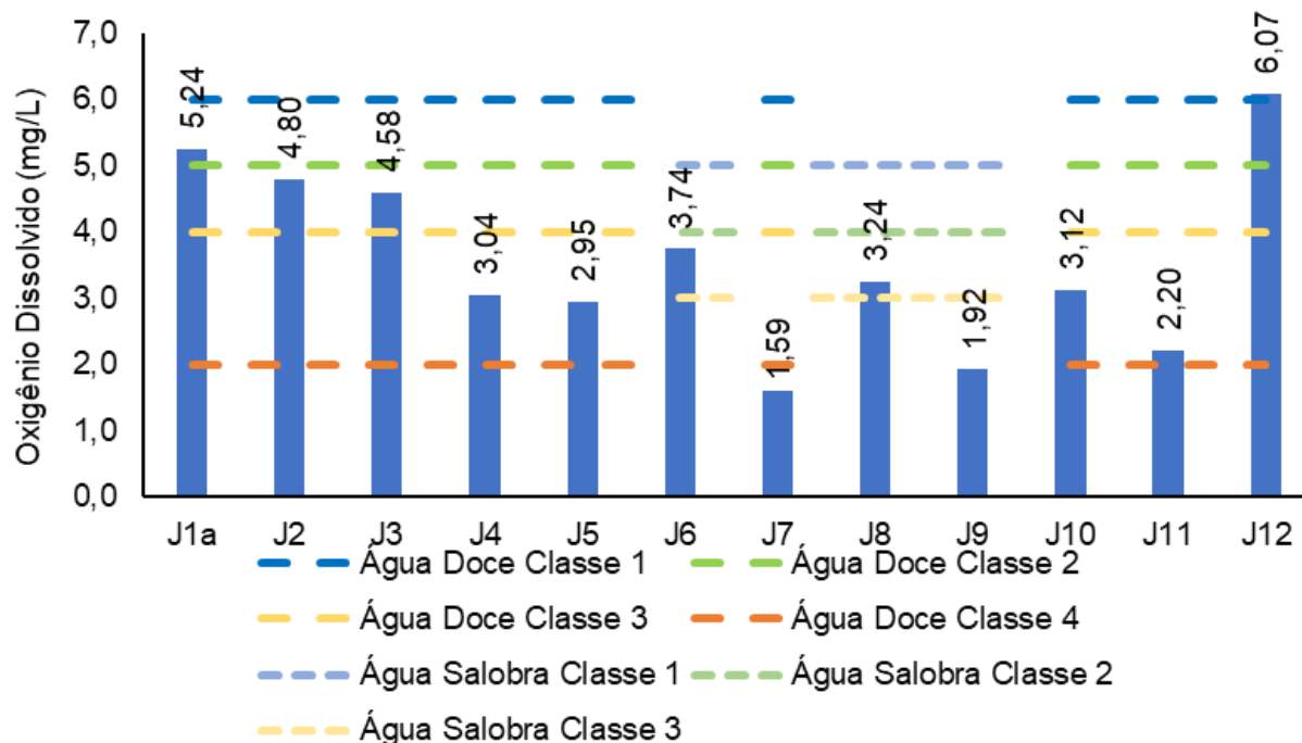
Figura V.2.1-15. Distribuição de oxigênio dissolvido na Sub-bacia do Sistema Lagunar de Jacarepaguá durante a campanha de novembro de 2023.
