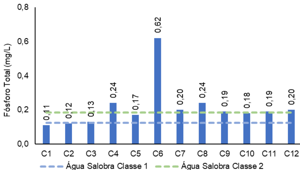
Figura V.2.1-44. Distribuição de fósforo total na Sub-bacia do Sistema Lagunar Itaipu-Piratininga durante a campanha de novembro de 2023.
