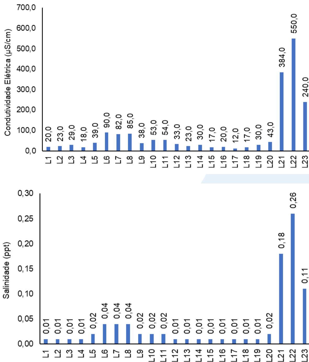
Figura V.2.1-49. Distribuição de condutividade e salinidade na Sub-bacia Leste durante a campanha de novembro de 2023.
