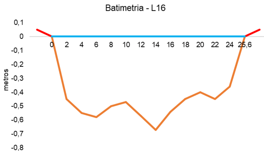
Figura V.2.3-19. Desenho esquemático da batimetria da estação L16 - Rio Guapiaçu.
