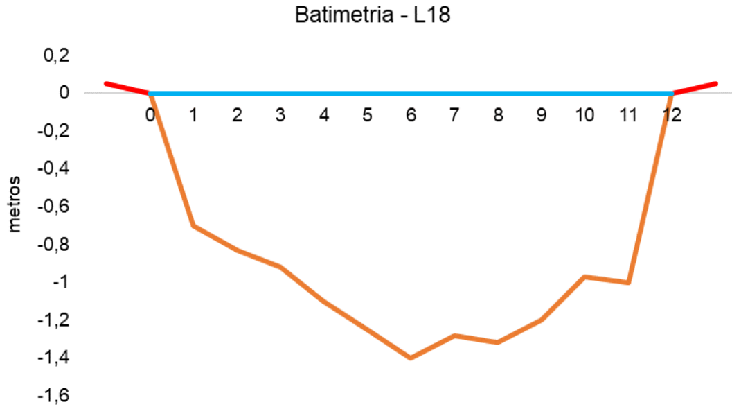
Figura V.2.3-20. Desenho esquemático da batimetria da estação L18 - Rio Guapiaçu.
