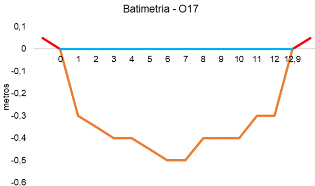
Figura V.2.3-37. Desenho esquemático da batimetria da estação O17 - Rio Sarapuí.
