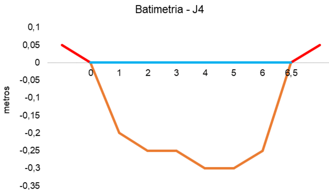
Figura V.2.3-1. Desenho esquemático da batimetria da estação J4 - Canal de Sernambetiba.
