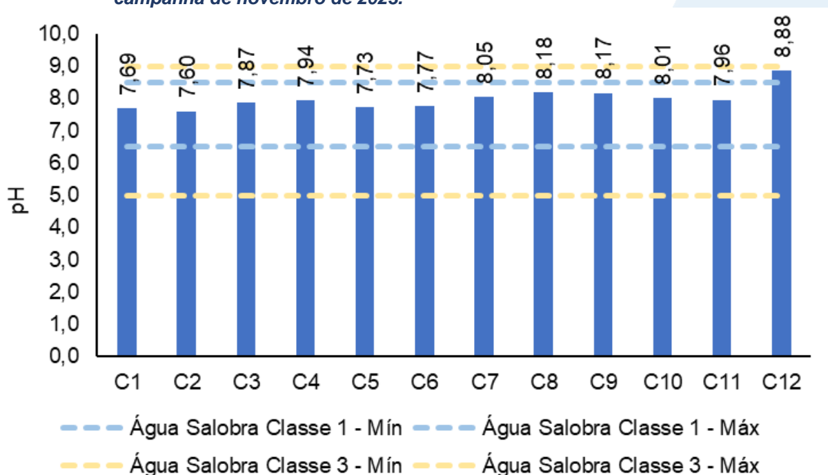
Figura V.2.1-42. Distribuição de pH na Sub-bacia do Sistema Lagunar Itaipu-Piratininga durante a campanha de novembro de 2023.
