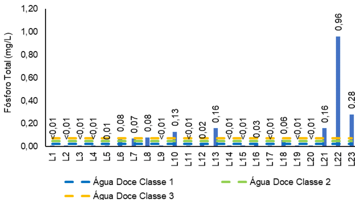
Figura V.2.1-56. Distribuição de fósforo total na Sub-bacia Leste durante a campanha de novembro de 2023.
