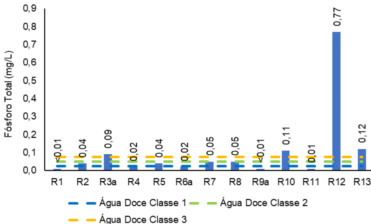
Figura V.2.1-32. Distribuição de fósforo total na Bacia da Lagoa Rodrigo de Freitas durante a campanha de novembro de 2023.
