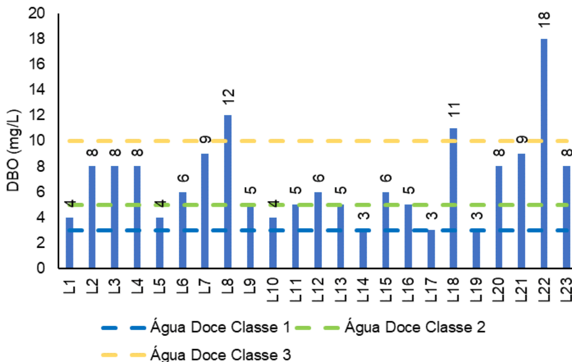
Figura V.2.1-52. Distribuição de DBO na Sub-bacia Leste durante a campanha de novembro de 2023.
