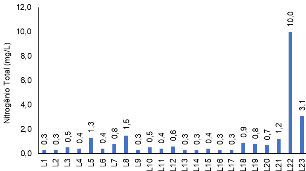
Figura V.2.1-58. Distribuição de nitrogênio total na Sub-bacia Leste durante a campanha de novembro de 2023.
