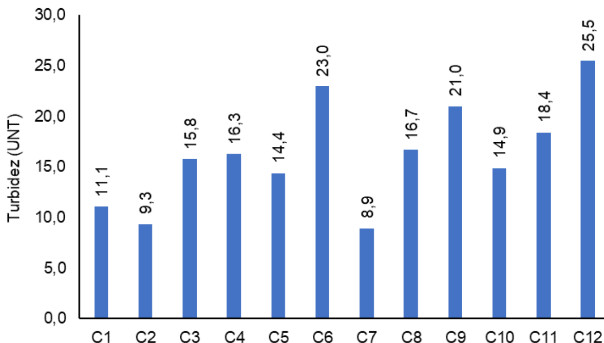
Figura V.2.1-43. Distribuição de turbidez na Sub-bacia do Sistema Lagunar Itaipu-Piratininga durante a campanha de novembro de 2023.
