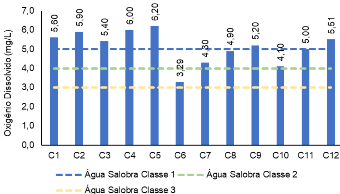
Figura V.2.1-39. Distribuição de oxigênio dissolvido na Sub-bacia do Sistema Lagunar Itaipu-Piratininga durante a campanha de novembro de 2023.
