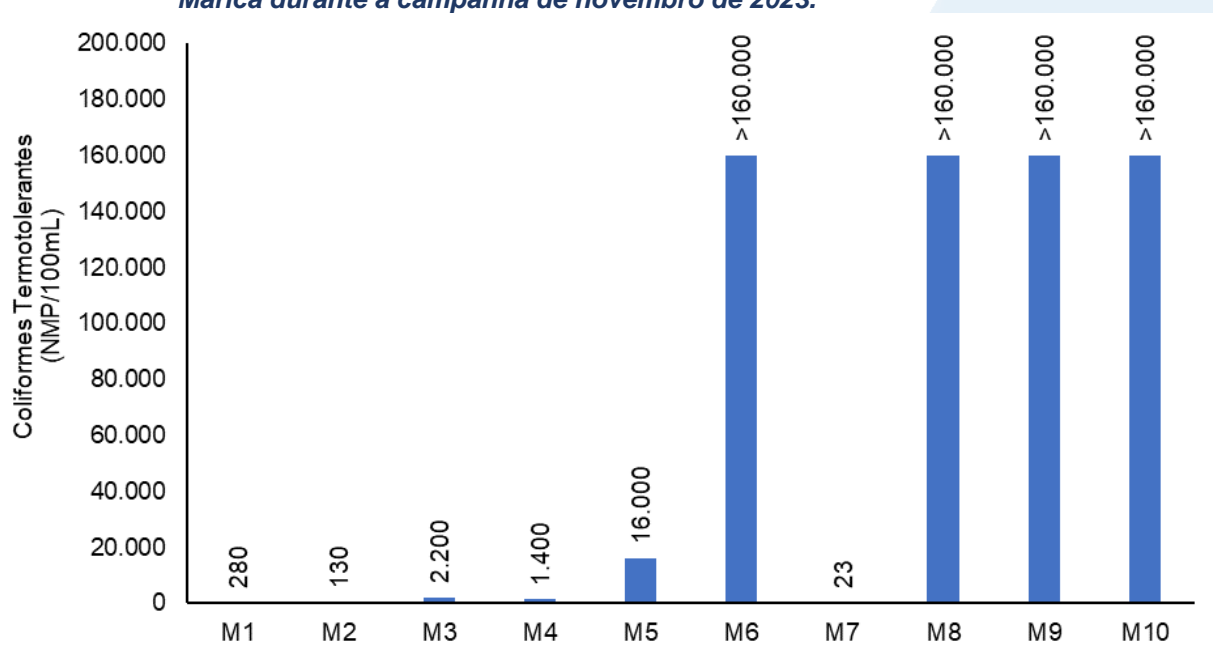
Figura V.2.1-12. Distribuição de coliformes termotolerantes na Sub-bacia do Sistema Lagunar de Maricá durante a campanha de novembro de 2023.
