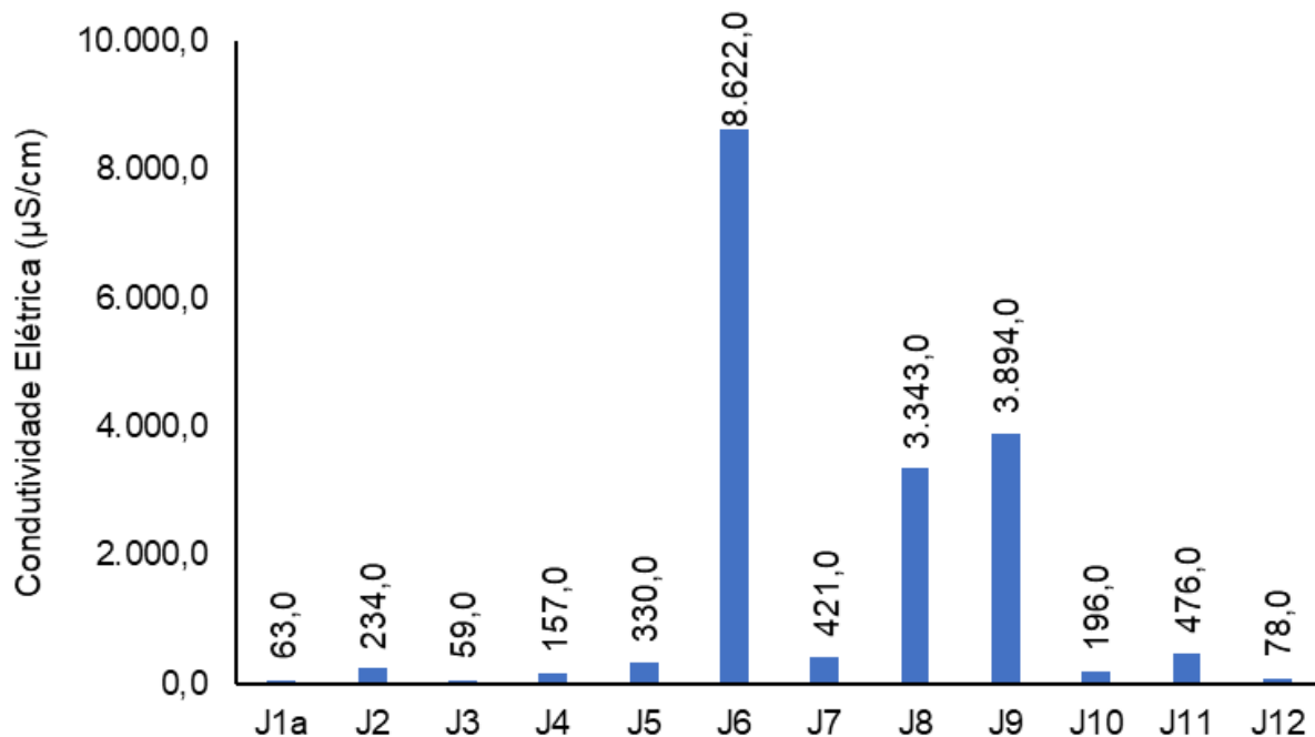
Figura V.2.1-13. Distribuição de condutividade e salinidade na Sub-bacia do Sistema Lagunar de Jacarepaguá durante a campanha de novembro de 2023.
