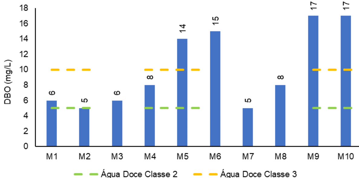
Figura V.2.1-4. Distribuição de DBO na Sub-bacia do Sistema Lagunar de Maricá durante a campanha de novembro de 2023.
