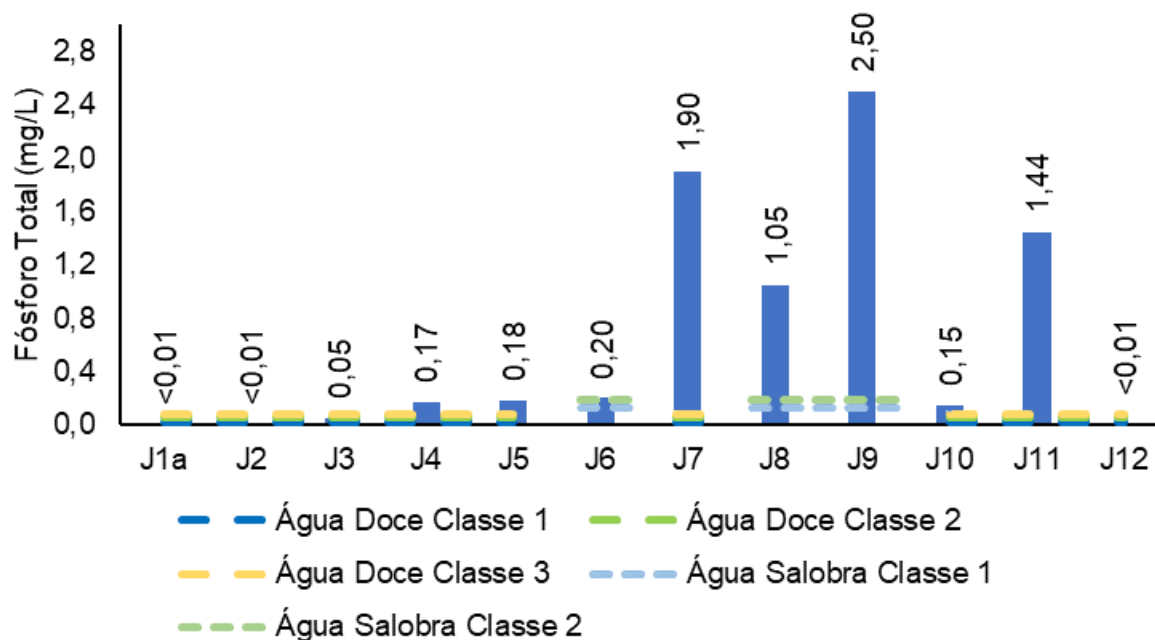
Figura V.2.1-20. Distribuição de fósforo total na Sub-bacia do Sistema Lagunar de Jacarepaguá durante a campanha de novembro de 2023.
