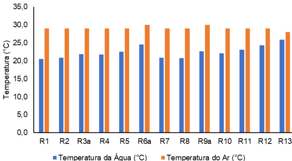
Figura V.2.1-26. Distribuição de temperatura do ar e da água na Bacia da Lagoa Rodrigo de Freitas durante a campanha de novembro de 2023.
