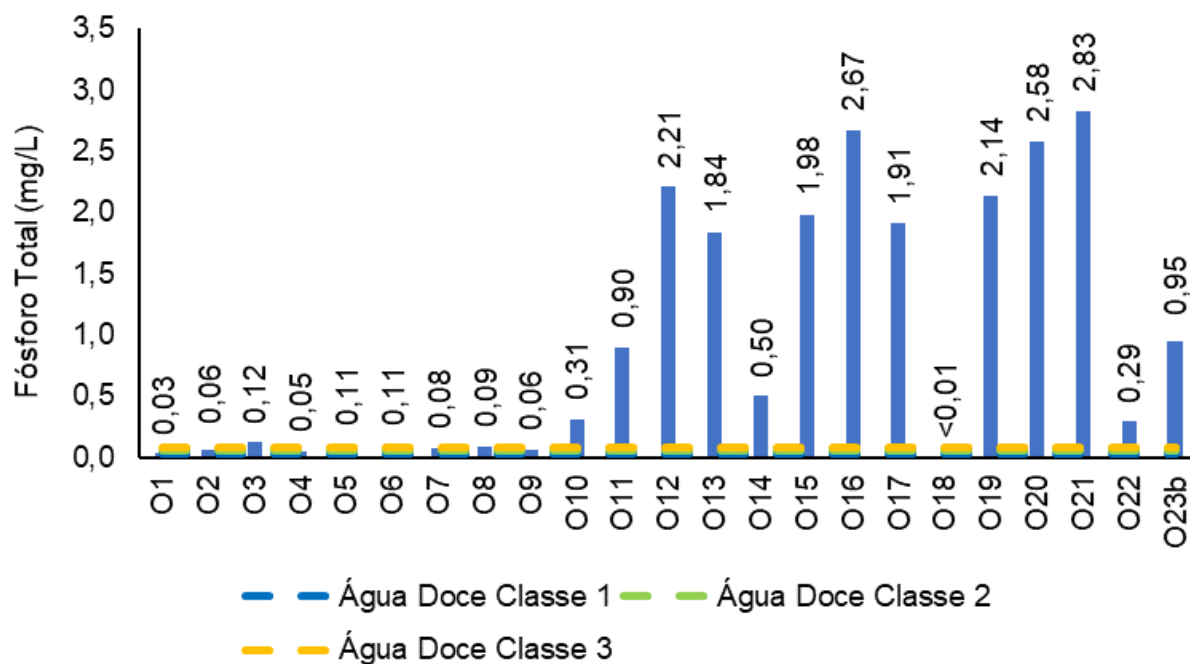
Figura V.2.1-68. Distribuição de fósforo total na Sub-bacia Oeste durante a campanha de novembro de 2023.
