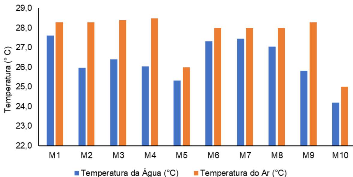
Figura V.2.1-2. Distribuição de temperatura do ar e da água na Sub-bacia do Sistema Lagunar de Maricá durante a campanha de novembro de 2023.
