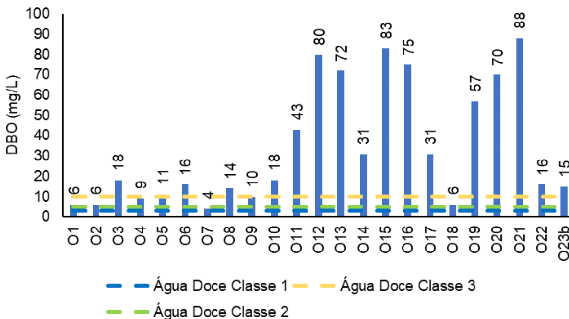
Figura V.2.1-64. Distribuição de DBO na Sub-bacia Oeste durante a campanha de novembro de 2023.
