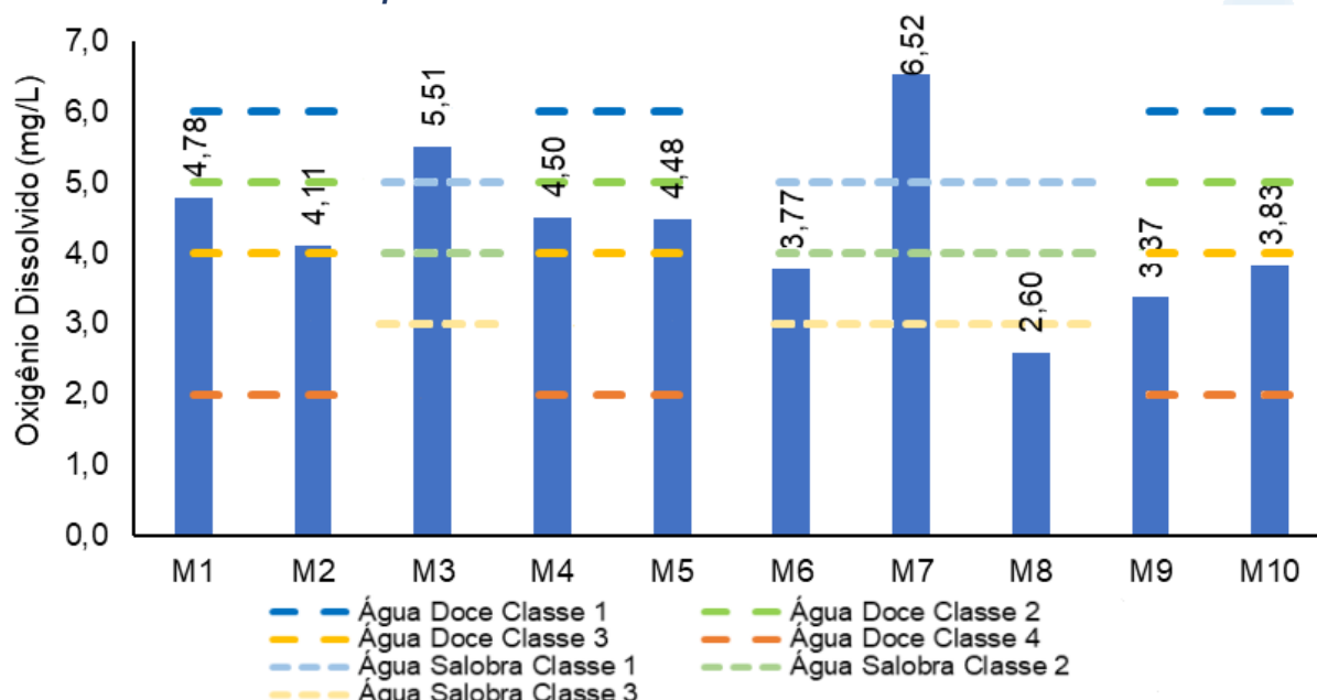
Figura V.2.1-3. Distribuição de oxigênio dissolvido na Sub-bacia do Sistema Lagunar de Maricá durante a campanha de novembro de 2023.
