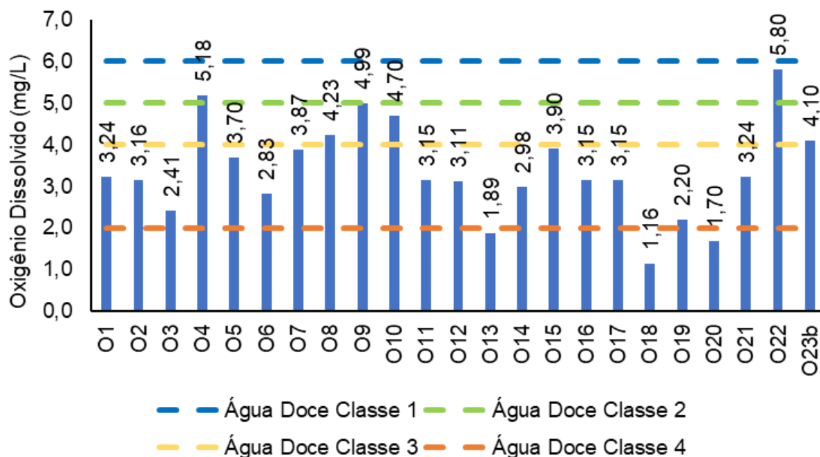
Figura V.2.1-63. Distribuição de oxigênio dissolvido na Sub-bacia Oeste durante a campanha de novembro de 2023.
