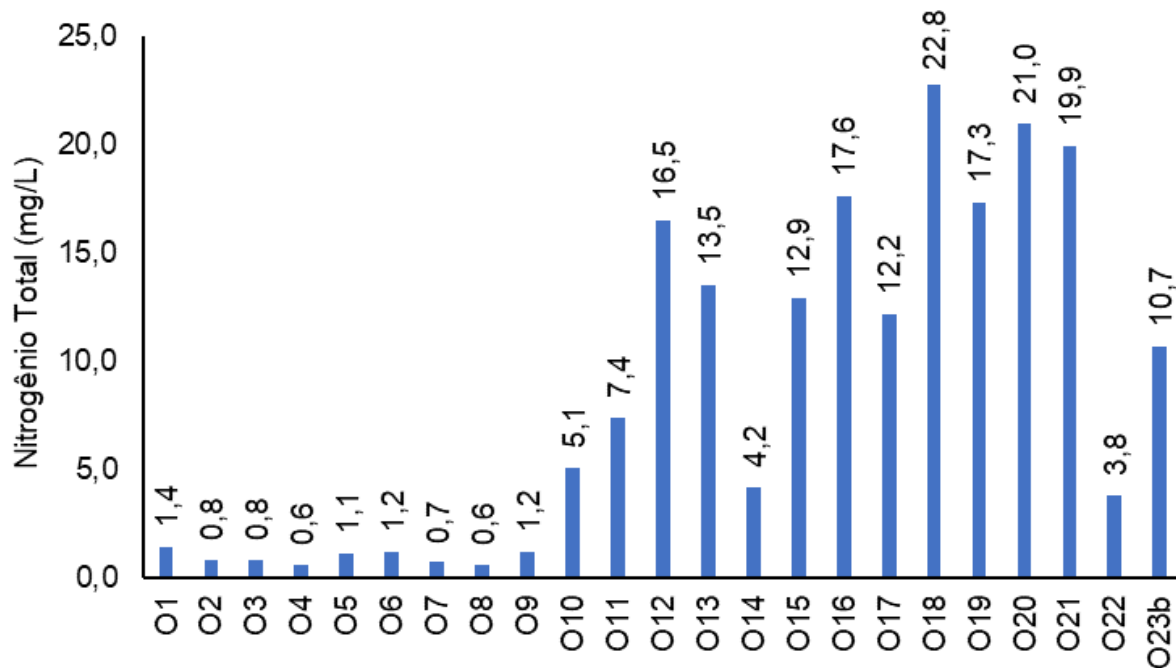
Figura V.2.1-70. Distribuição de nitrogênio total na Sub-bacia Oeste durante a campanha de novembro de 2023.
