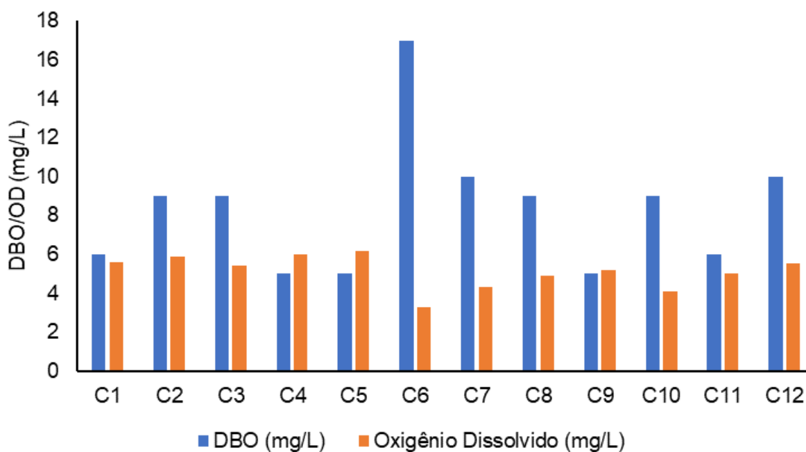
Figura V.2.1-41. Comparativo de DBO e OD na Sub-bacia do Sistema Lagunar Itaipu-Piratininga durante a campanha de novembro de 2023.
