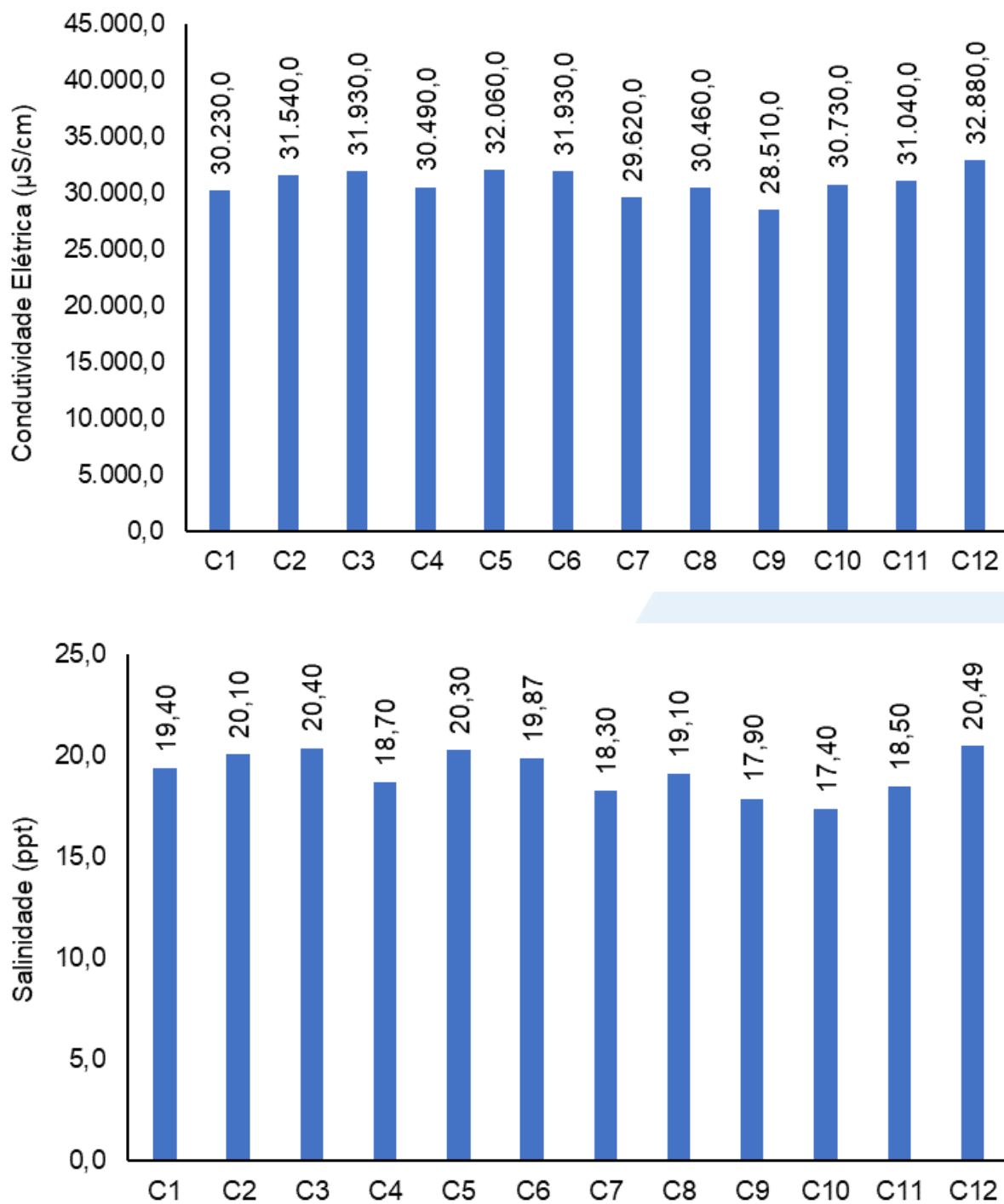
Figura V.2.1-37. Distribuição de condutividade e salinidade na Sub-bacia do Sistema Lagunar Itaipu-Piratininga durante a campanha de novembro de 2023.
