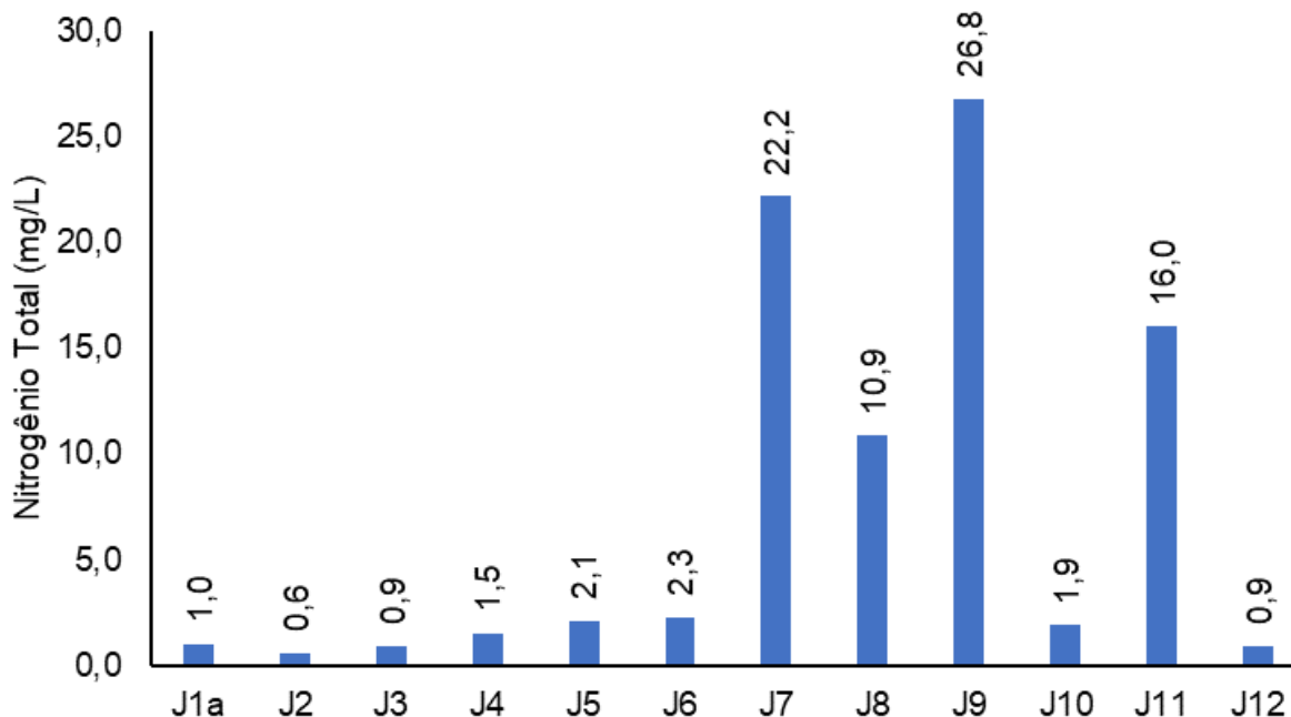
Figura V.2.1-22. Distribuição de nitrogênio total na Sub-bacia do Sistema Lagunar de Jacarepaguá durante a campanha de novembro de 2023.
