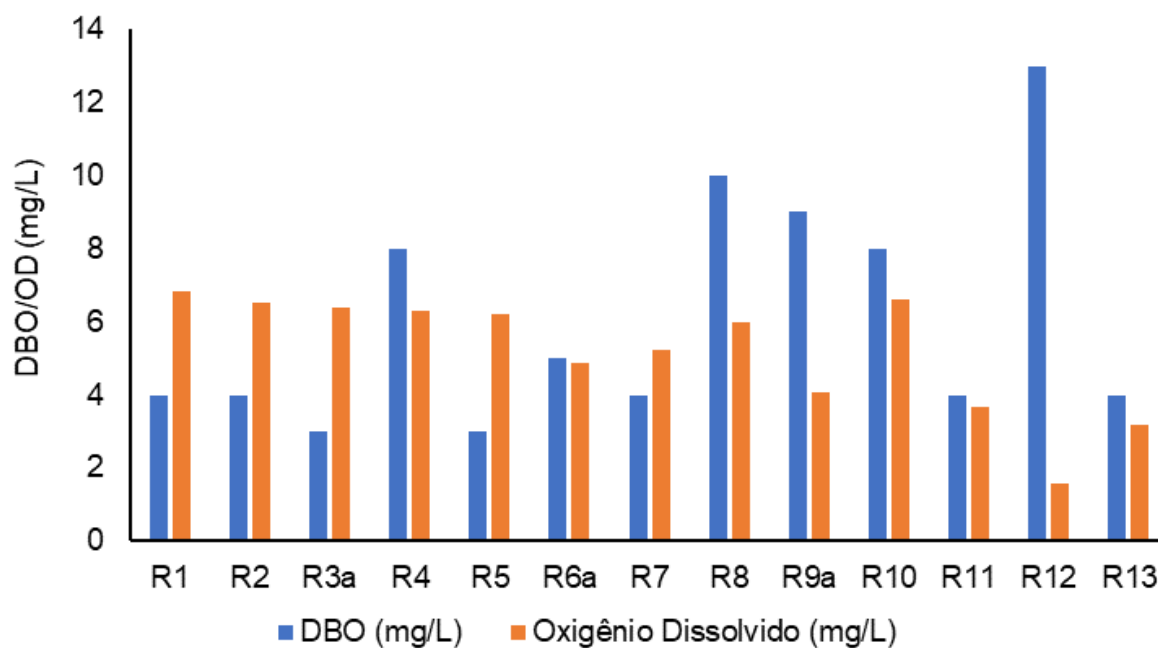
Figura V.2.1-29. Comparativo entre disponibilidade de OD e DBO na Bacia da Lagoa Rodrigo de Freitas durante a campanha de novembro de 2023.
