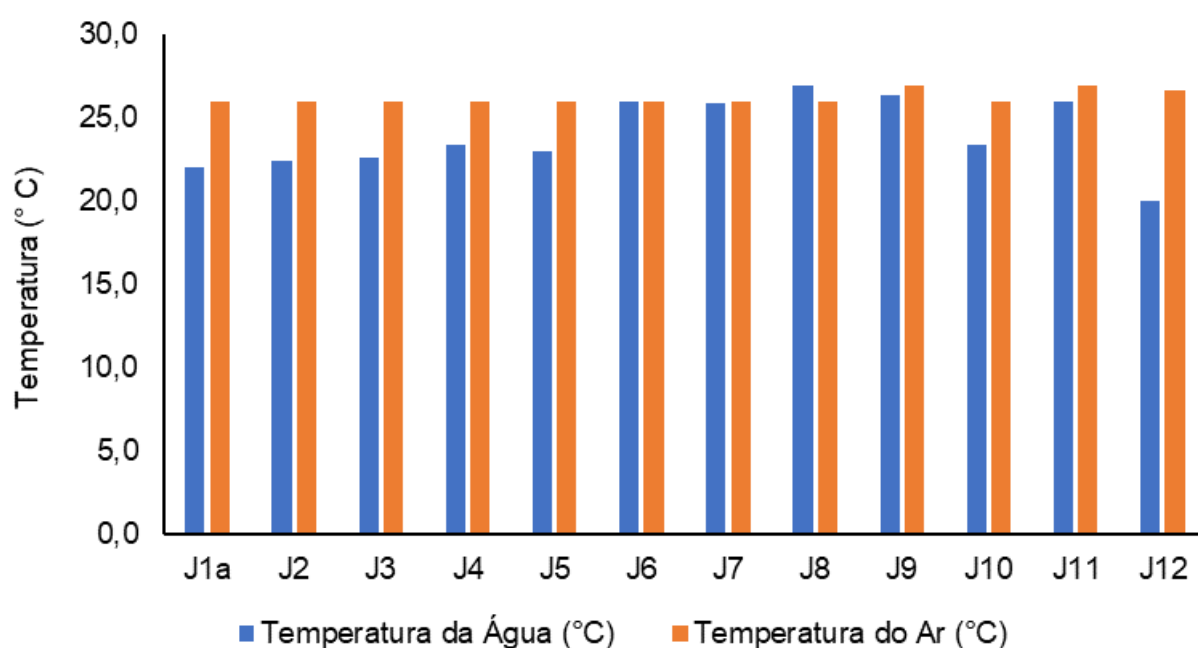
Figura V.2.1-14. Distribuição de temperatura do ar e da água na Sub-bacia do Sistema Lagunar de Jacarepaguá durante a campanha de novembro de 2023.
