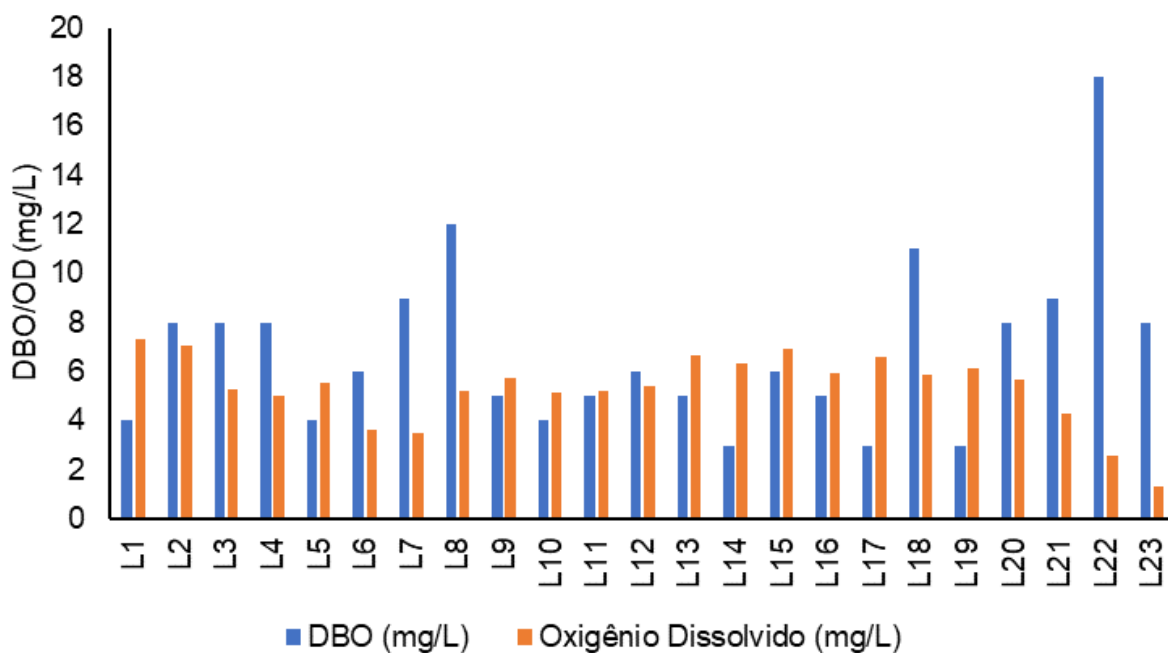
Figura V.2.1-53. Comparativo da concentração de OD e DBO na Sub-bacia Leste durante a campanha de novembro de 2023.
