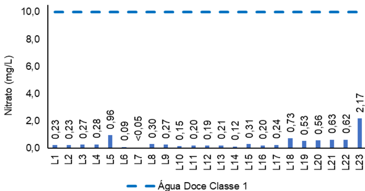
Figura V.2.1-57. Distribuição de nitrato na região Leste da Baía de Guanabara durante a campanha de novembro de 2023.
