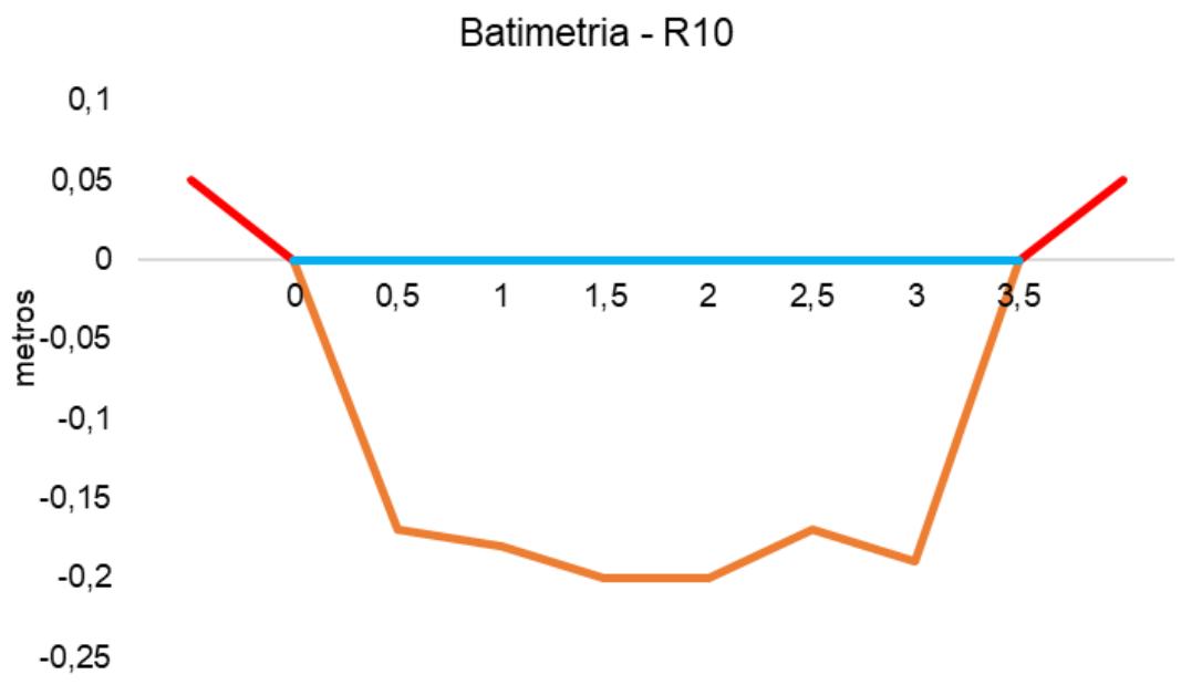
Figura V-78. Desenho esquemático da batimetria da estação R10 - Rio Rainha.
