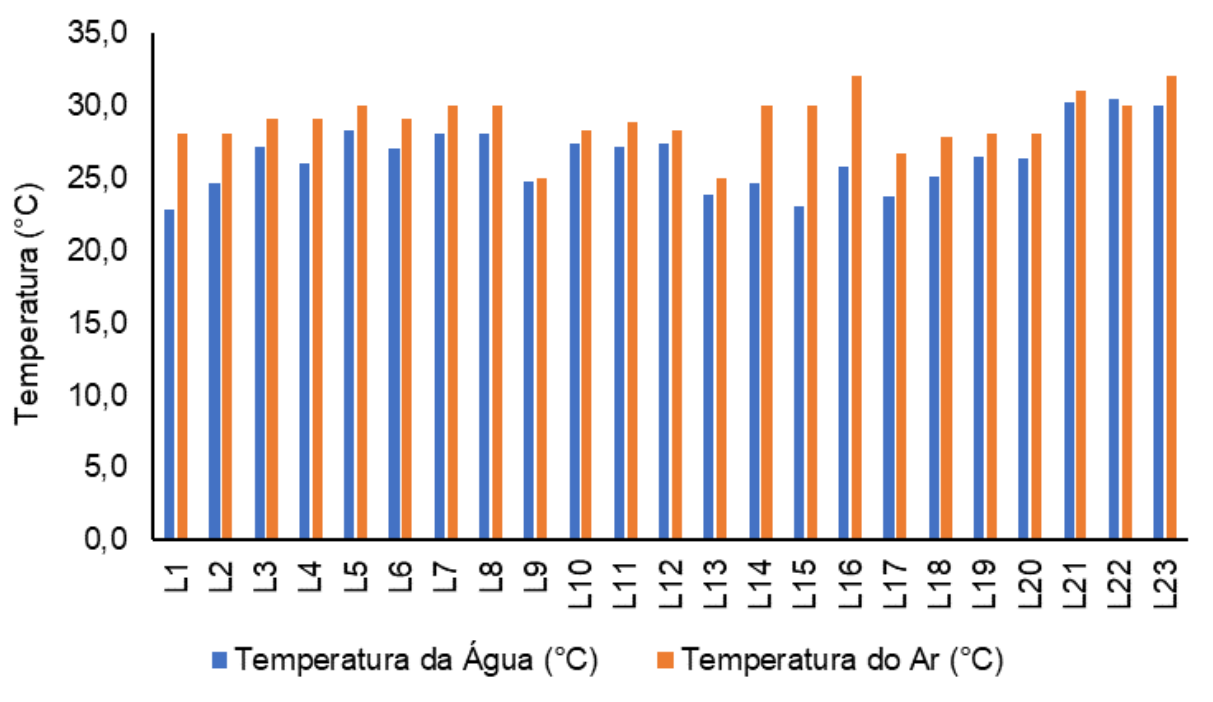
Figura V-50. Distribuição de temperatura do ar e da água na Sub-bacia Leste durante a campanha de outubro de 2023.
