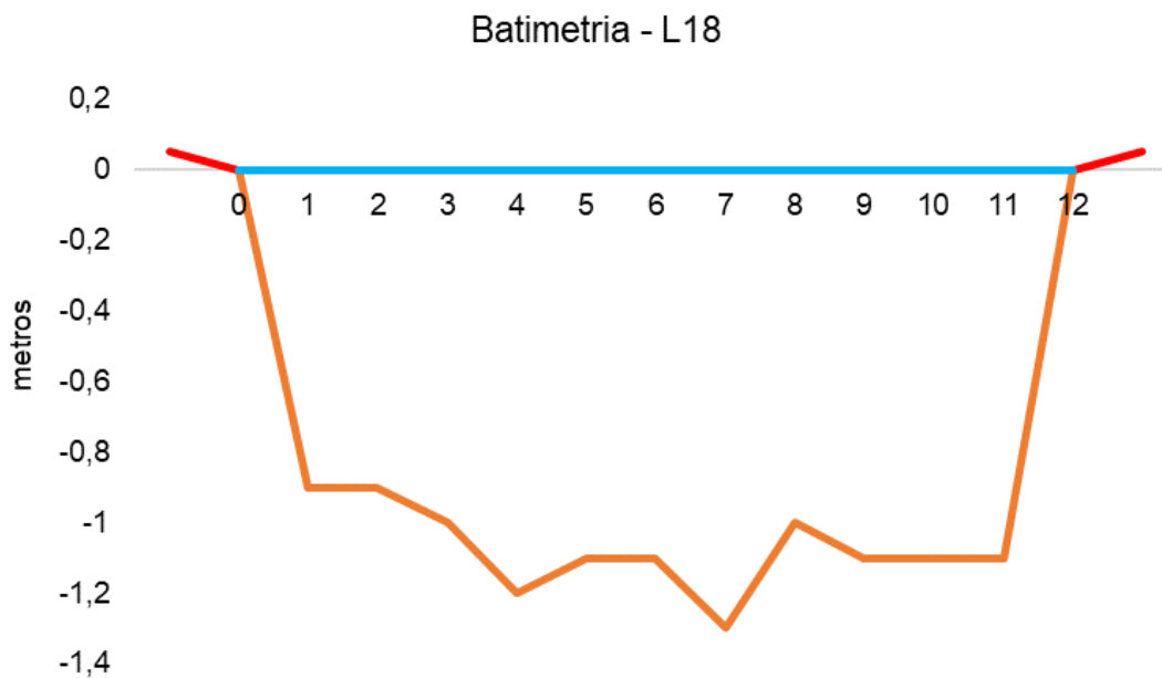
Figura V-92. Desenho esquemático da batimetria da estação L18 - Rio Guapiaçu.
