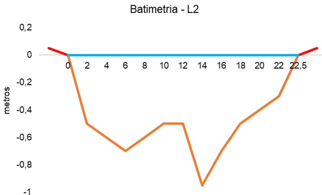
Figura V-80. Desenho esquemático da batimetria da estação L2 - Rio Macacu.
