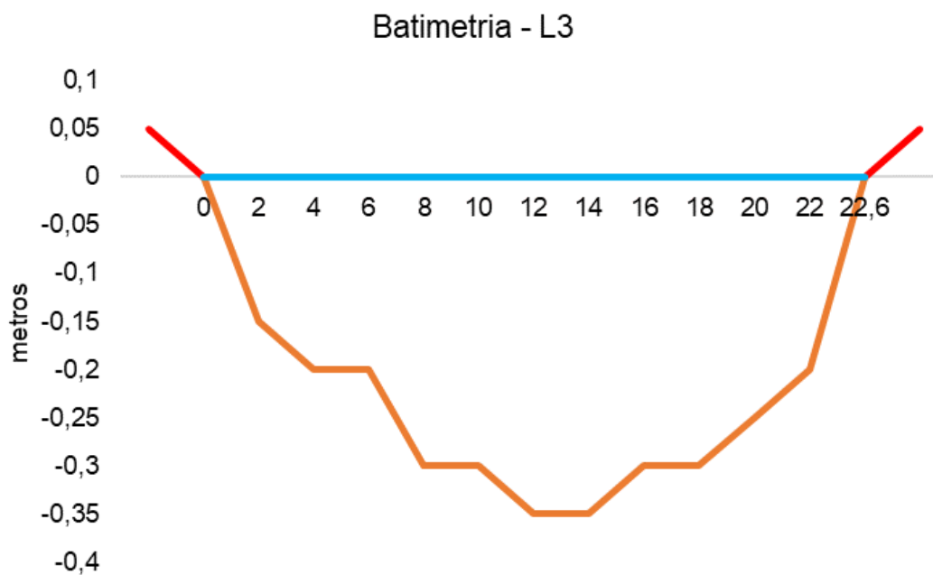
Figura V-81. Desenho esquemático da batimetria da estação L3 - Rio Macacu.
