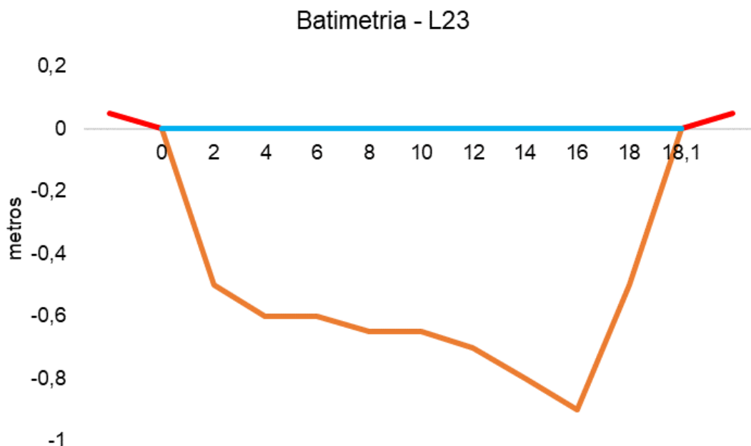
Figura V-96. Desenho esquemático da batimetria da estação L23 - Afluente do Rio Caceribu.
