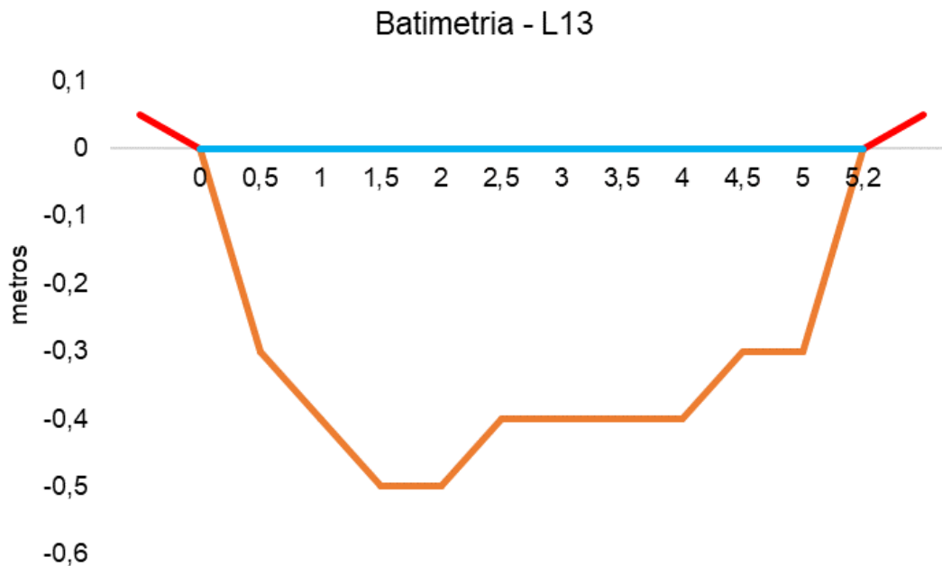
Figura V-88. Desenho esquemático da batimetria da estação L13 - Rio Itaperi.
