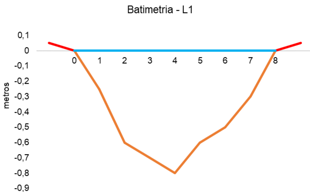
Figura V-79. Desenho esquemático da batimetria da estação L1 - Rio Macacu.
