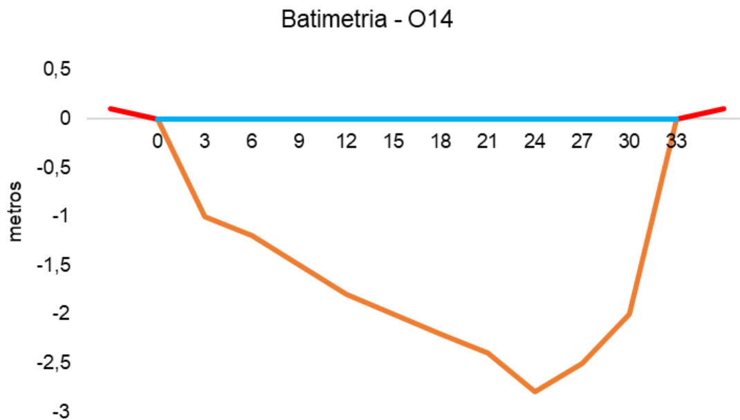
Figura V-108. Desenho esquemático da batimetria da estação O14 - Rio Iguaçu.
