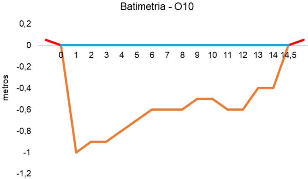
Figura V-104. Desenho esquemático da batimetria da estação O10 - Rio Iguaçu.
