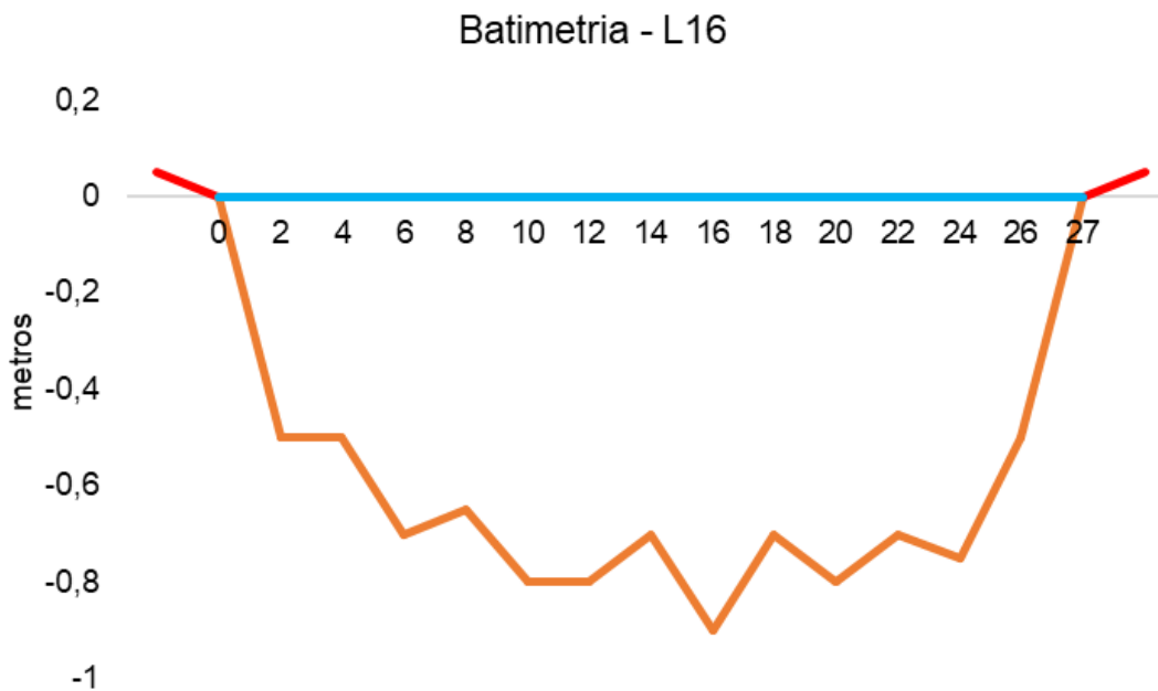
Figura V-91. Desenho esquemático da batimetria da estação L16 - Rio Guapiaçu.
