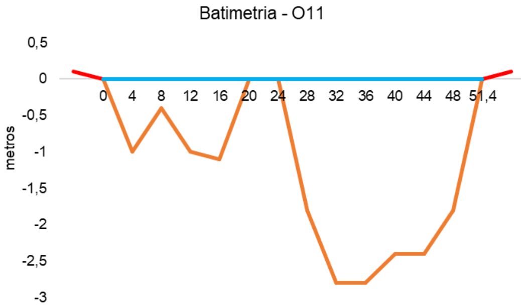
Figura V-105. Desenho esquemático da batimetria da estação O11 - Rio Iguaçu.
