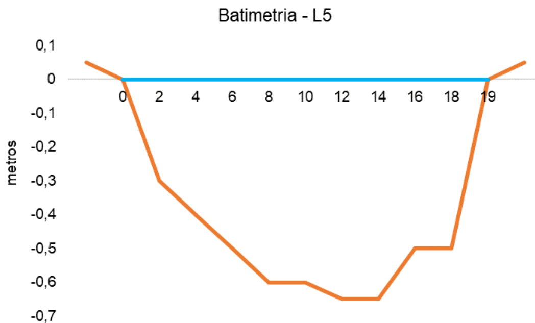
Figura V-83. Desenho esquemático da batimetria da estação L5 - Rio Macacu.
