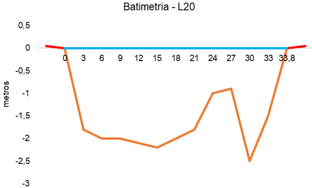
Figura V-94. Desenho esquemático da batimetria da estação L20 - Rio Guapiaçu.
