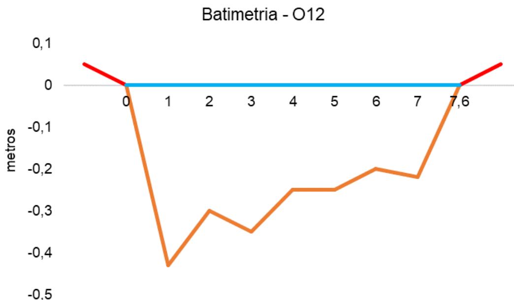
Figura V-106. Desenho esquemático da batimetria da estação O12 - Rio Botas.
