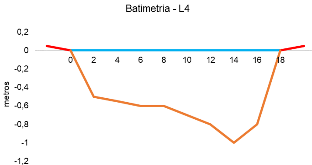
Figura V-82. Desenho esquemático da batimetria da estação L4 - Rio Macacu.
