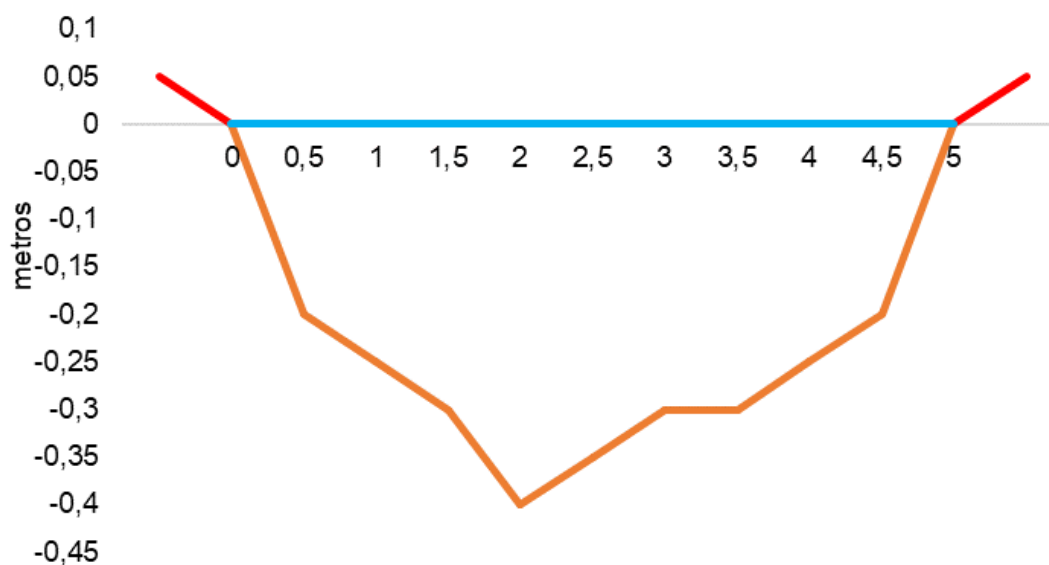
Figura V-85. Desenho esquemático da batimetria da estação L8 - Papucainha.
