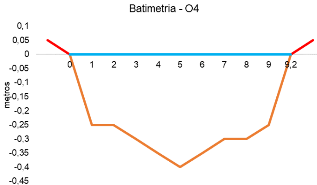
Figura V-99. Desenho esquemático da batimetria da estação O4 - Rio Sapucaia.
