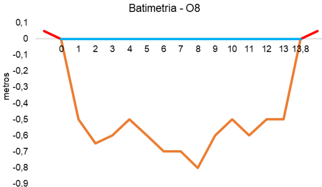
Figura V-102. Desenho esquemático da batimetria da estação O8 - Rio Tinguá.
