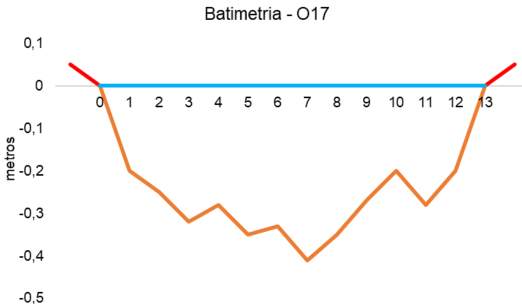
Figura V-110. Desenho esquemático da batimetria da estação O17 - Rio Sarapuí.
