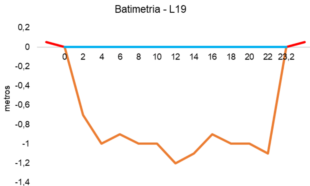
Figura V-93. Desenho esquemático da batimetria da estação L19 - Rio Guapiaçu.
