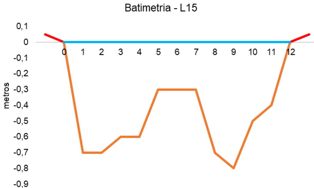
Figura V-90. Desenho esquemático da batimetria da estação L15 - Rio Guapiaçu.
