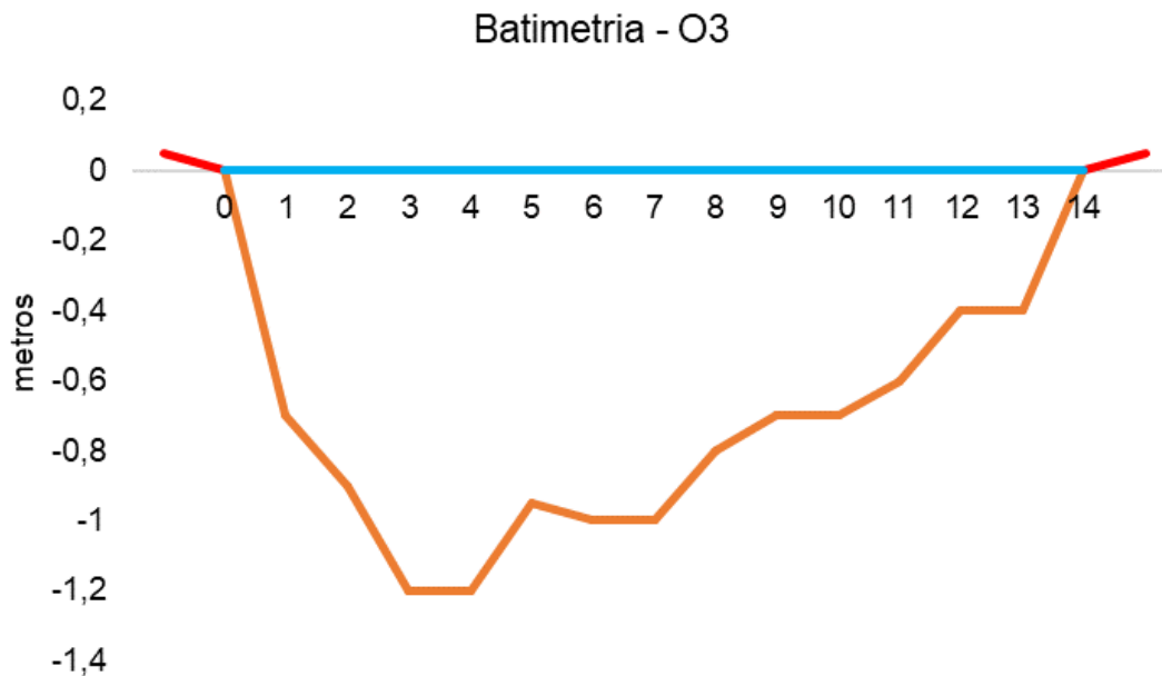
Figura V-98. Desenho esquemático da batimetria da estação O3 - Rio Saracuruna.
