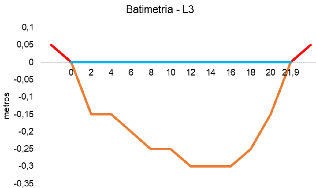
Figura V-79. Desenho esquemático da batimetria da estação L3 - Rio Macacu.
