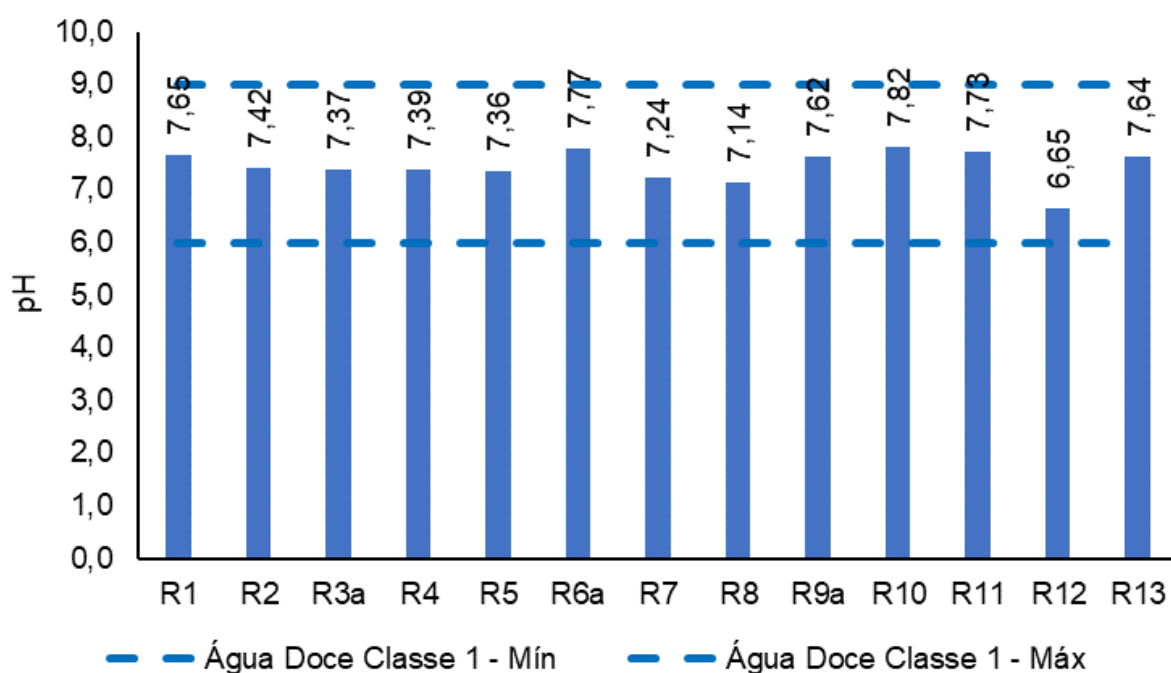
Figura V-30. Distribuição de pH na Bacia da Lagoa Rodrigo de Freitas durante a campanha de julho de 2023.
