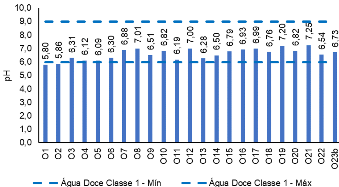
Figura V-66. Distribuição de pH na Sub-bacia Oeste durante a campanha de julho de 2023.
