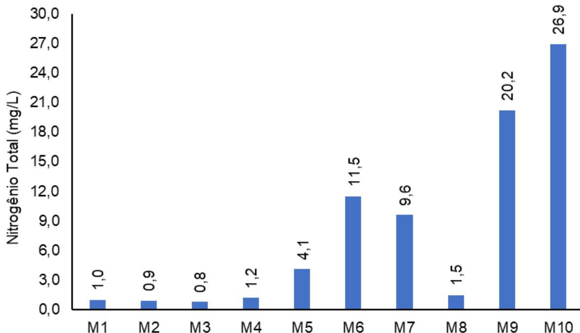
Figura V-10. Distribuição de nitrogênio total na Sub-bacia do Sistema Lagunar de Maricá durante a campanha de julho de 2023.
