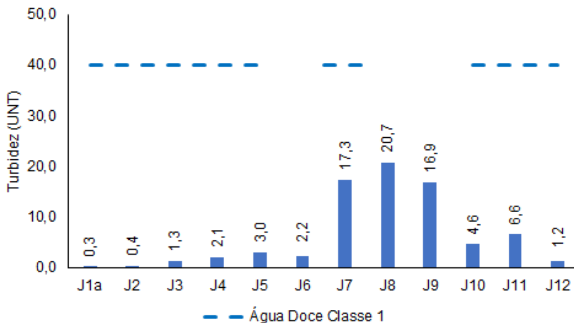
Figura V-19. Distribuição de turbidez na Sub-bacia do Sistema Lagunar de Jacarepaguá durante a campanha de julho de 2023.
