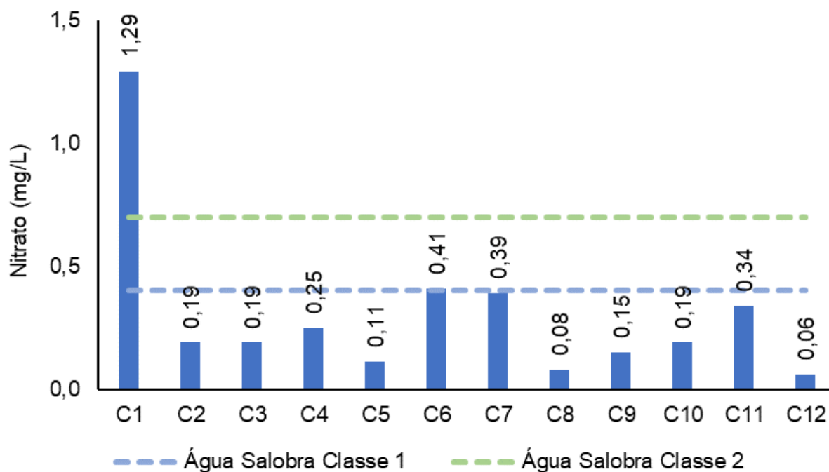
Figura V-45. Distribuição de nitrato na Sub-bacia do Sistema Lagunar Itaipu-Piratininga durante a campanha de julho de 2023.
