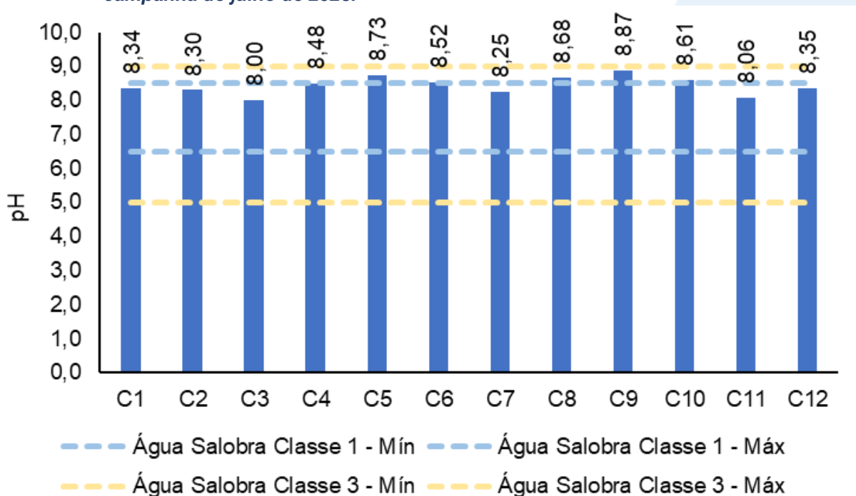
Figura V-42. Distribuição de pH na Sub-bacia do Sistema Lagunar Itaipu-Piratininga durante a campanha de julho de 2023.
