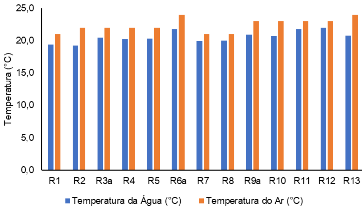
Figura V-26. Distribuição de temperatura do ar e da água na Bacia da Lagoa Rodrigo de Freitas durante a campanha de julho de 2023.
