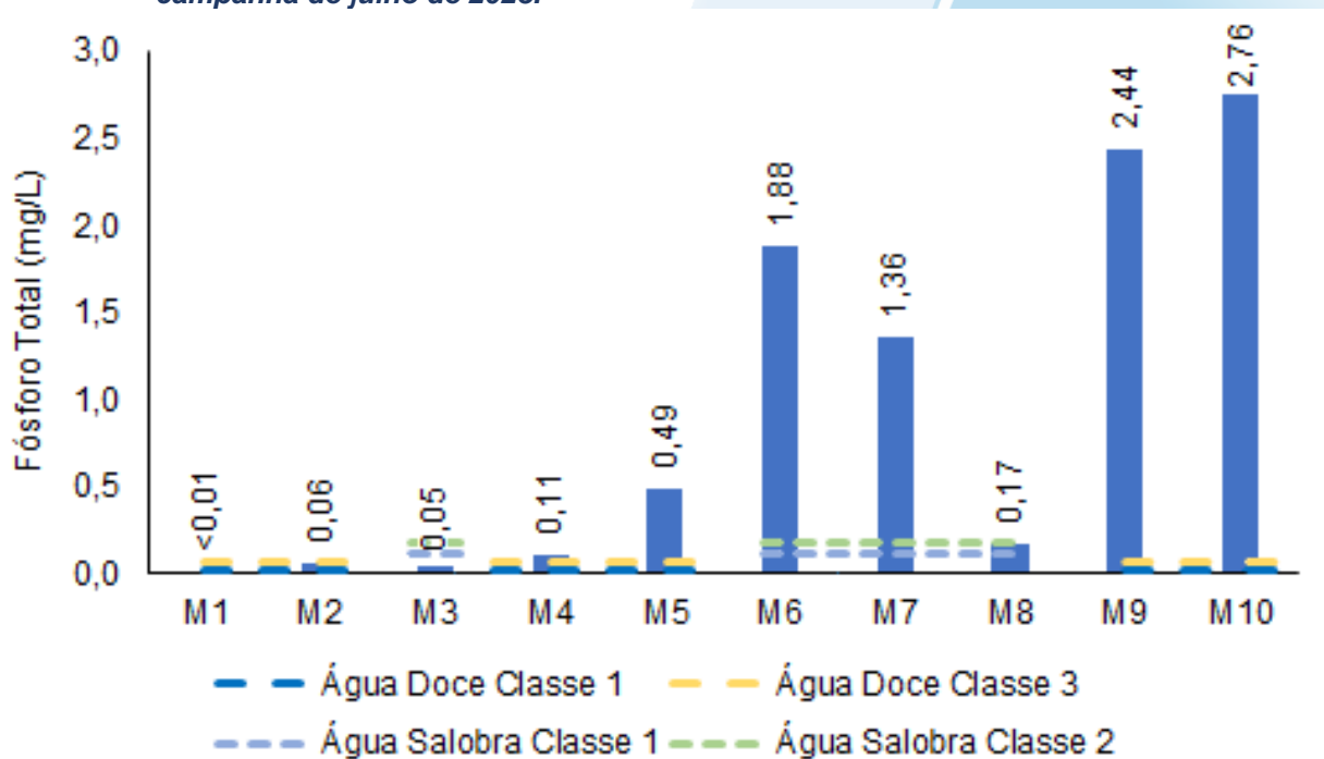
Figura V-8. Distribuição de fósforo total na Sub-bacia do Sistema Lagunar de Maricá durante a campanha de julho de 2023.
