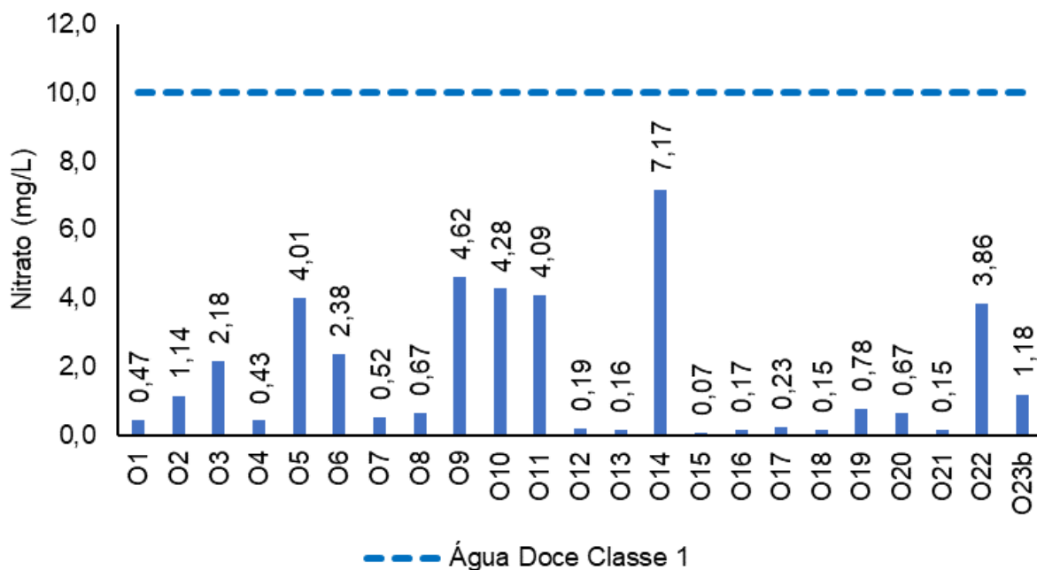
Figura V-69. Distribuição de nitrato na Sub-bacia Oeste durante a campanha de julho de 2023.
