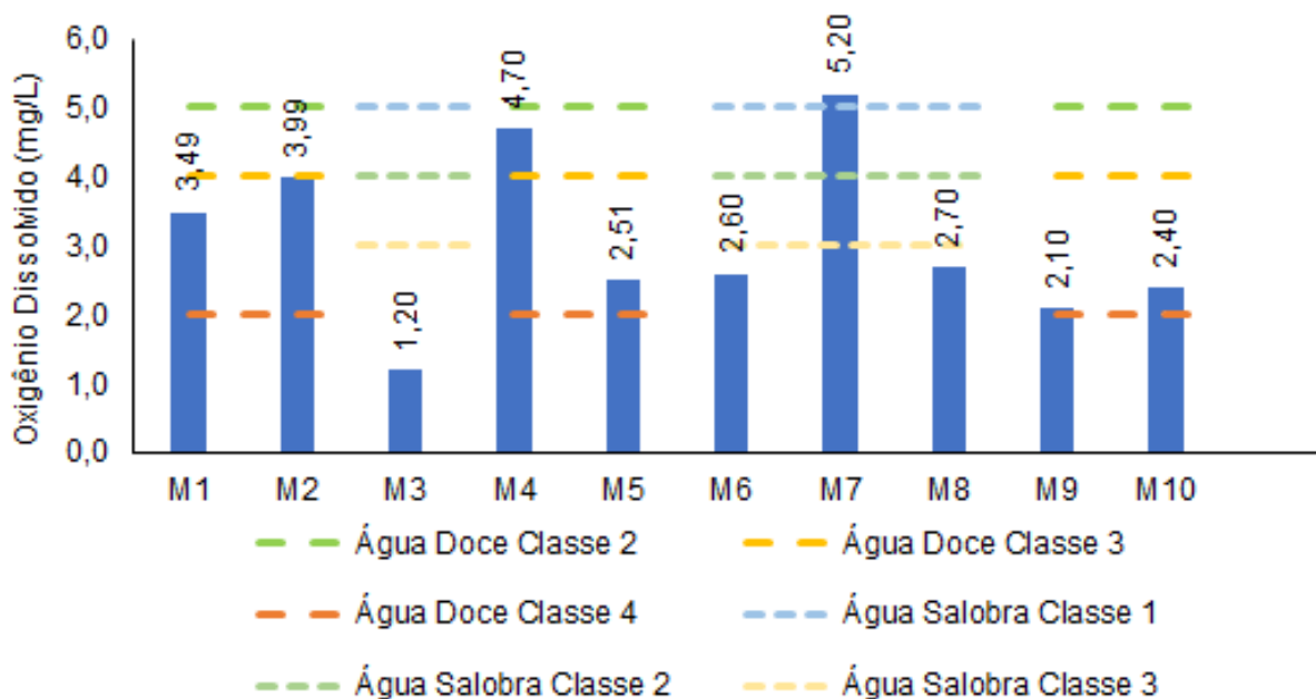
Figura V-3. Distribuição de oxigênio dissolvido na Sub-bacia do Sistema Lagunar de Maricá durante a campanha de julho de 2023.
