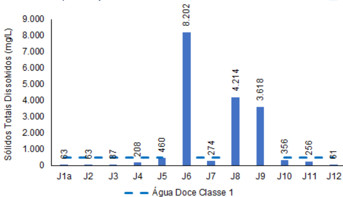
Figura V-23. Distribuição de STD na Sub-bacia do Sistema Lagunar de Jacarepaguá durante a campanha de julho de 2023.
