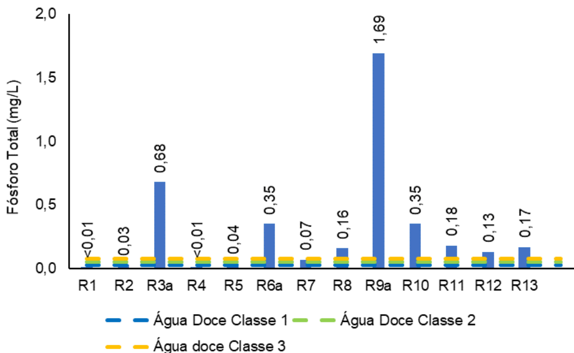
Figura V-32. Distribuição de fósforo total na Bacia da Lagoa Rodrigo de Freitas durante a campanha de julho de 2023.
