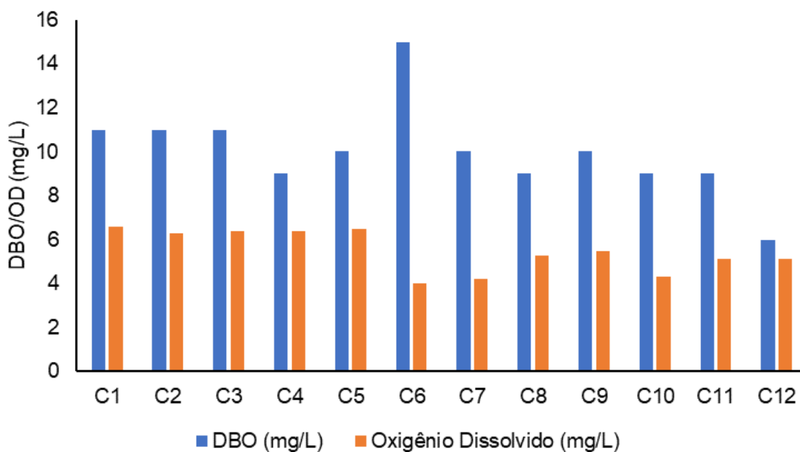
Figura V-41. Comparativo de DBO e OD na Sub-bacia do Sistema Lagunar Itaipu-Piratininga durante a campanha de julho de 2023.
