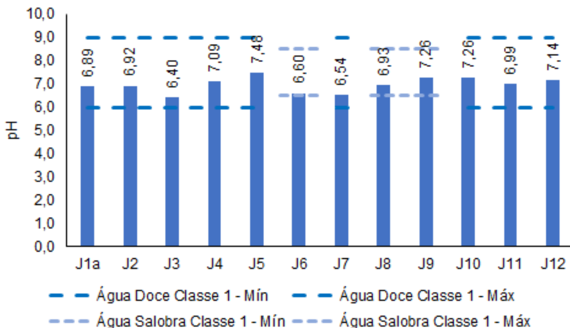
Figura V-18. Distribuição de pH na Sub-bacia do Sistema Lagunar de Jacarepaguá durante a campanha de julho de 2023.
