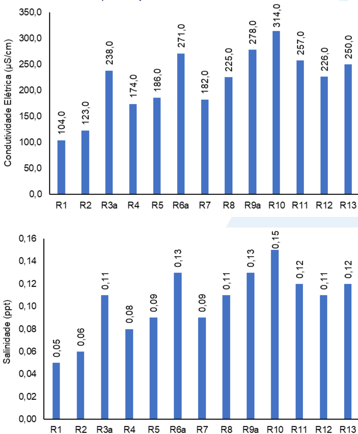
Figura V-25. Distribuição de condutividade e salinidade na Bacia da Lagoa Rodrigo de Freitas durante a campanha de julho de 2023.
