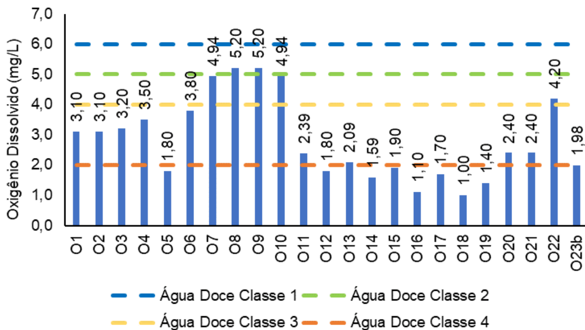
Figura V-63. Distribuição de oxigênio dissolvido na Sub-bacia Oeste durante a campanha de julho de 2023.
