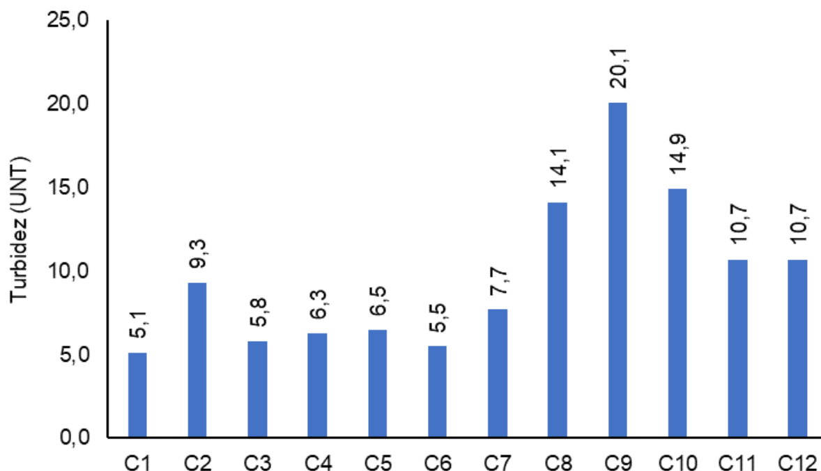
Figura V-43. Distribuição de turbidez na Sub-bacia do Sistema Lagunar Itaipu-Piratininga durante a campanha de julho de 2023.
