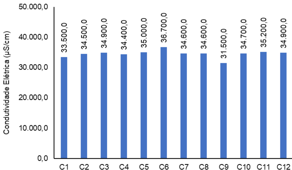
Figura V-37. Distribuição de condutividade e salinidade na Sub-bacia do Sistema Lagunar Itaipu-Piratininga durante a campanha de julho de 2023.
