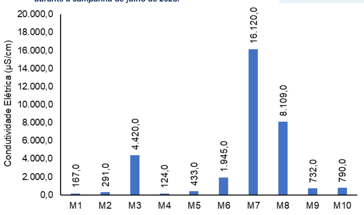
Figura V-1. Distribuição de condutividade e salinidade na Sub-bacia do Sistema Lagunar de Maricá durante a campanha de julho de 2023.
