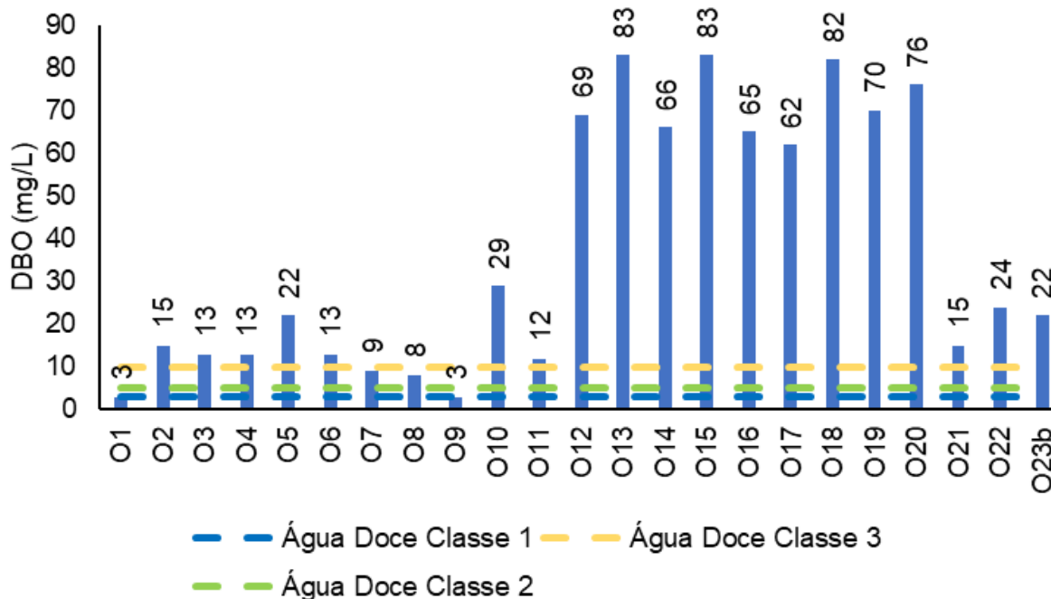
Figura V-64. Distribuição de DBO na Sub-bacia Oeste durante a campanha de julho de 2023.
