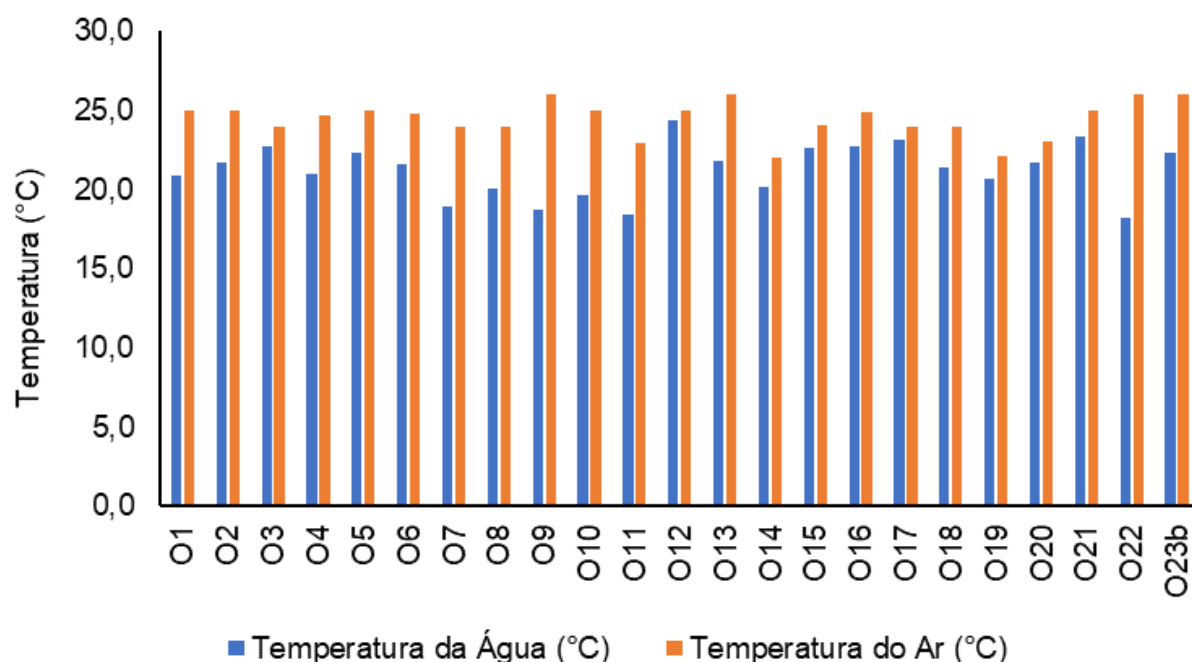
Figura V-62. Distribuição de temperatura do ar e da água na Sub-bacia Oeste durante a campanha de julho de 2023.
