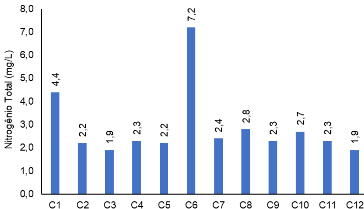
Figura V-46. Distribuição de nitrogênio total na Sub-bacia do Sistema Lagunar Itaipu-Piratininga durante a campanha de julho de 2023.
