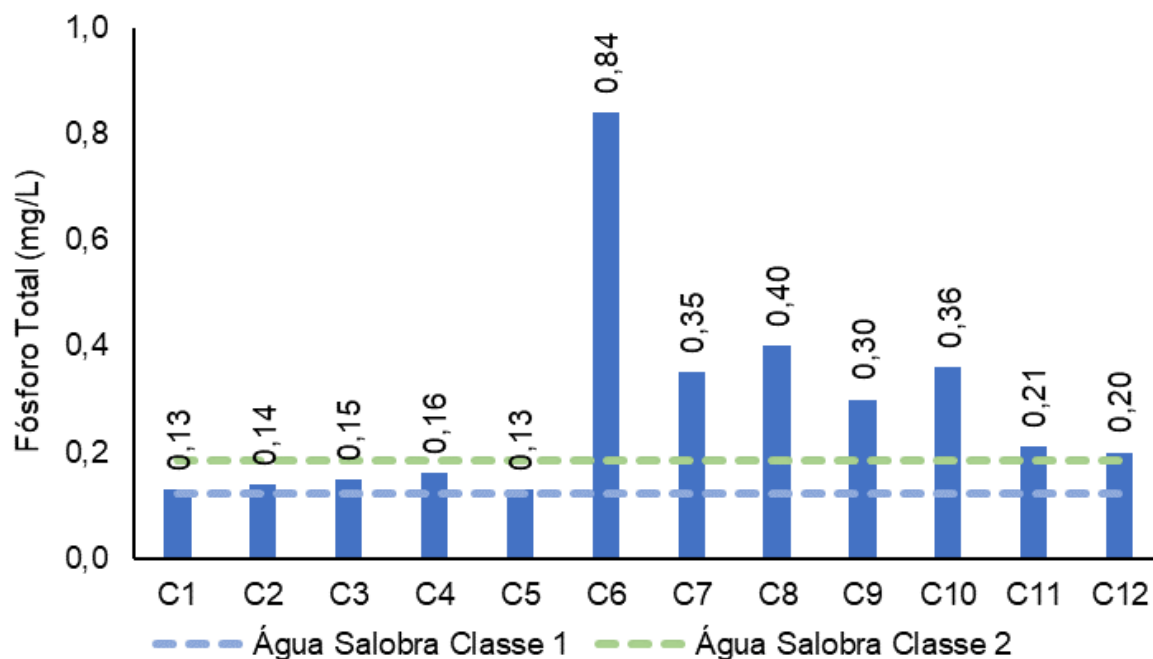
Figura V-44. Distribuição de fósforo total na Sub-bacia do Sistema Lagunar Itaipu-Piratininga durante a campanha de julho de 2023.
