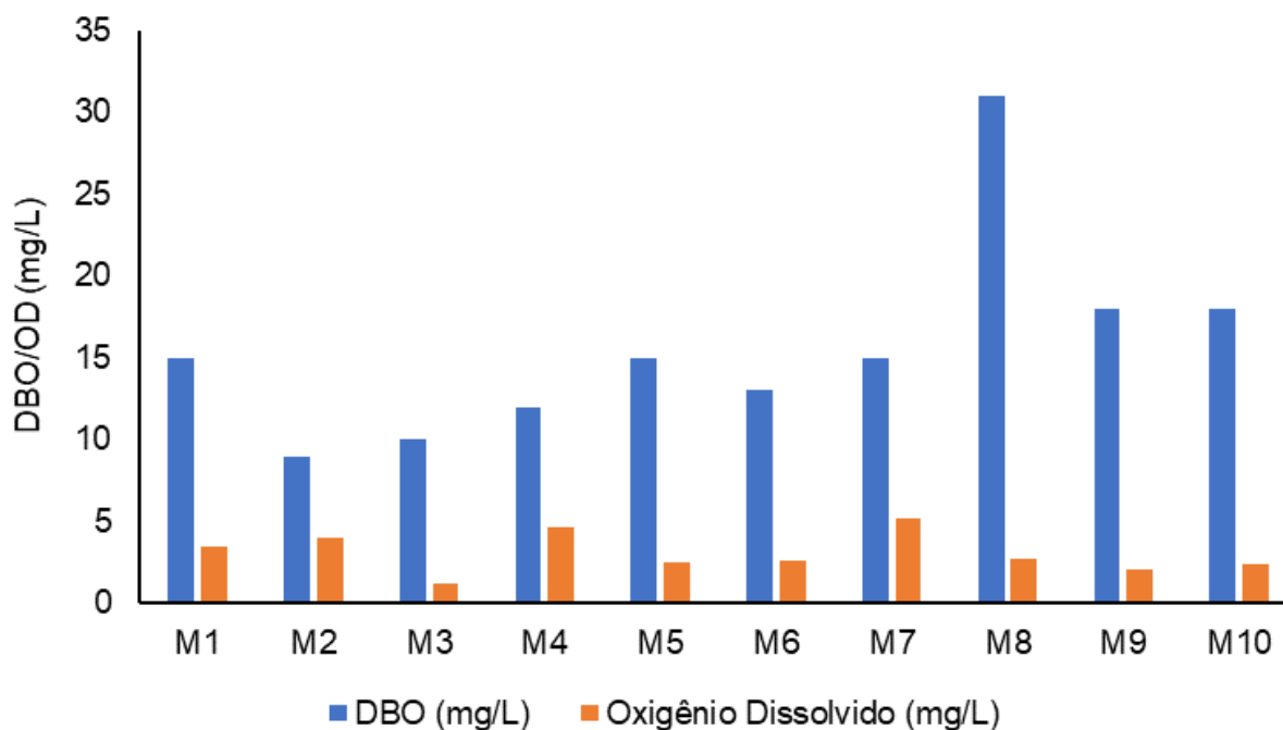
Figura V-5. Comparativo entre disponibilidade de oxigênio dissolvido e DBO na Sub-bacia do Sistema Lagunar de Maricá durante a campanha de julho de 2023.
