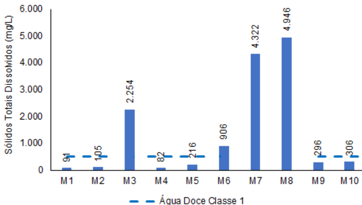
Figura V-11. Distribuição de STD na Sub-bacia do Sistema Lagunar de Maricá durante a campanha de julho de 2023.
