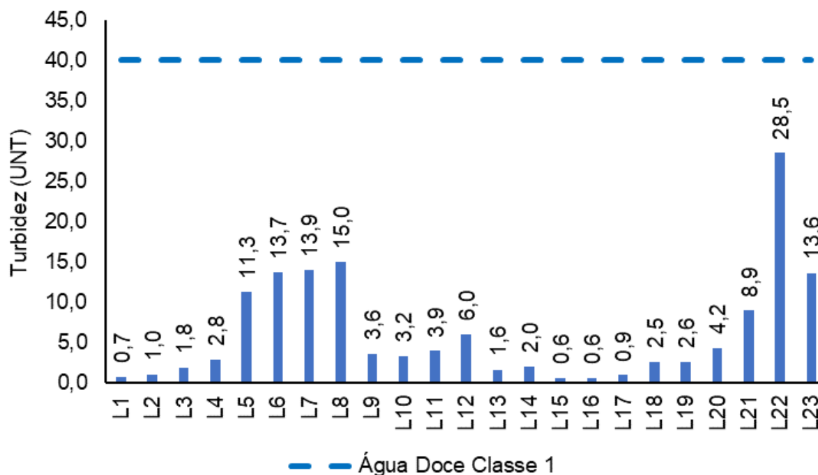
Figura V-55. Distribuição de turbidez na Sub-bacia Leste durante a campanha de julho de 2023.
