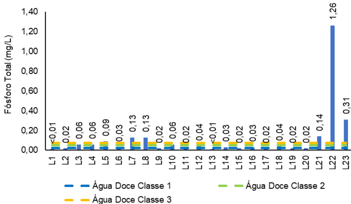
Figura V-56. Distribuição de fósforo total na Sub-bacia Leste durante a campanha de julho de 2023.
