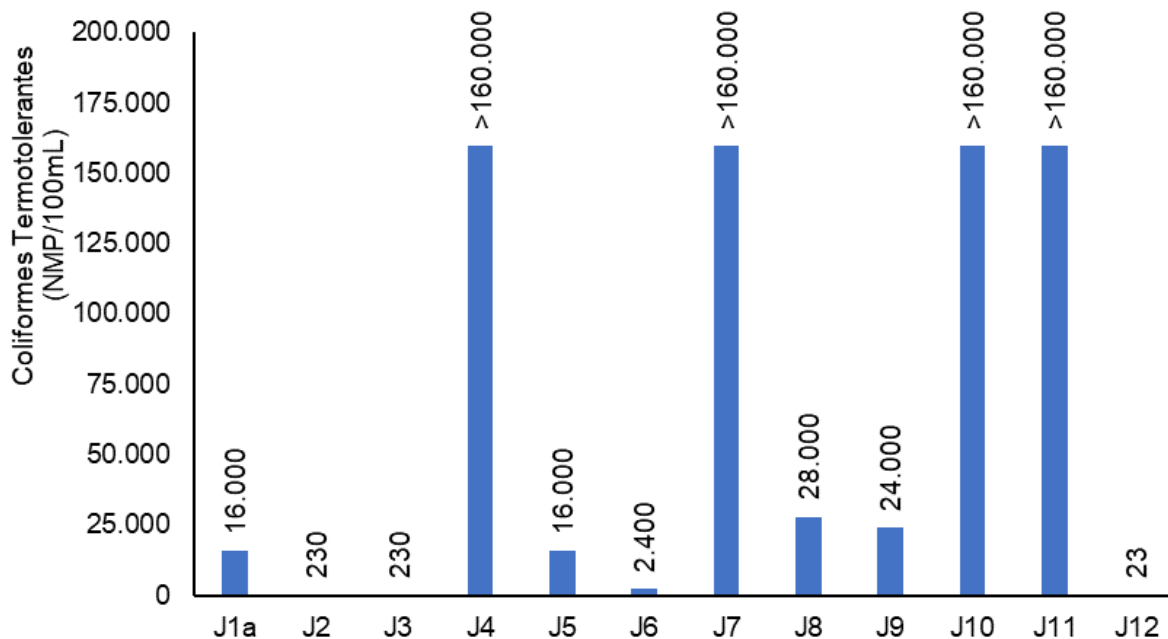
Figura V-24. Distribuição de coliformes termotolerantes na Sub-bacia do Sistema Lagunar de Jacarepaguá durante a campanha de julho de 2023.
