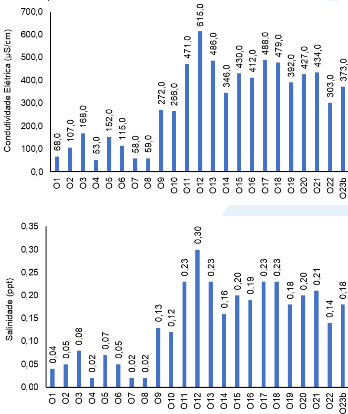
Figura V-61. Distribuição de condutividade e salinidade na Sub-bacia Oeste durante a campanha de julho de 2023.
