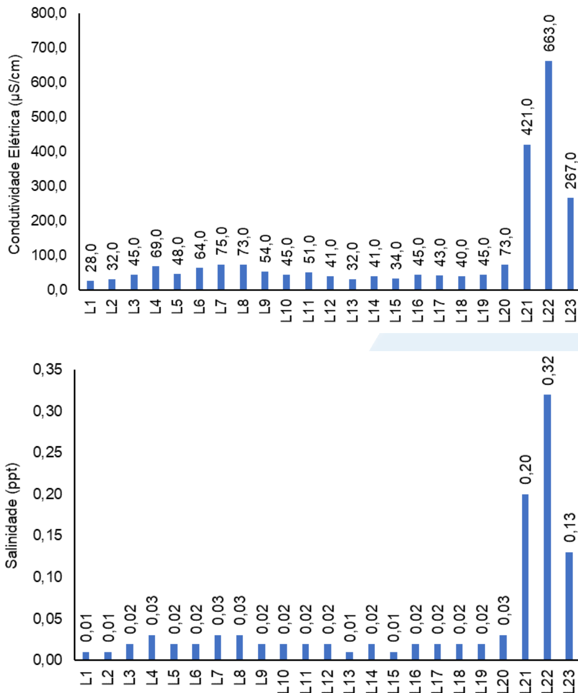
Figura V-49. Distribuição de condutividade e salinidade na Sub-bacia Leste durante a campanha de julho de 2023.
