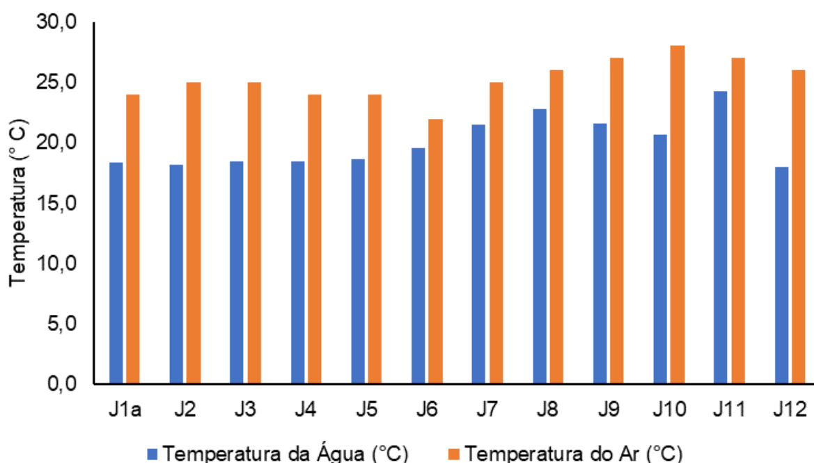
Figura V-14. Distribuição de temperatura do ar e da água na Sub-bacia do Sistema Lagunar de Jacarepaguá durante a campanha de julho de 2023.
