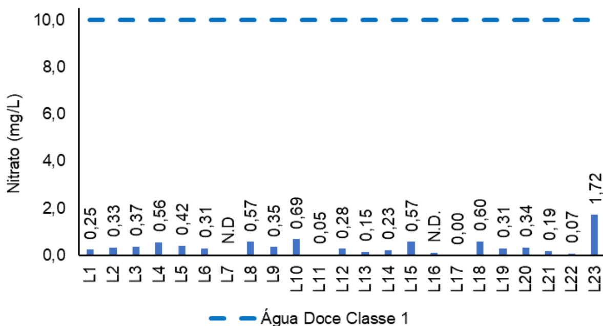
Figura V-57. Distribuição de nitrato na região Leste da Baía de Guanabara durante a campanha de julho de 2023.
