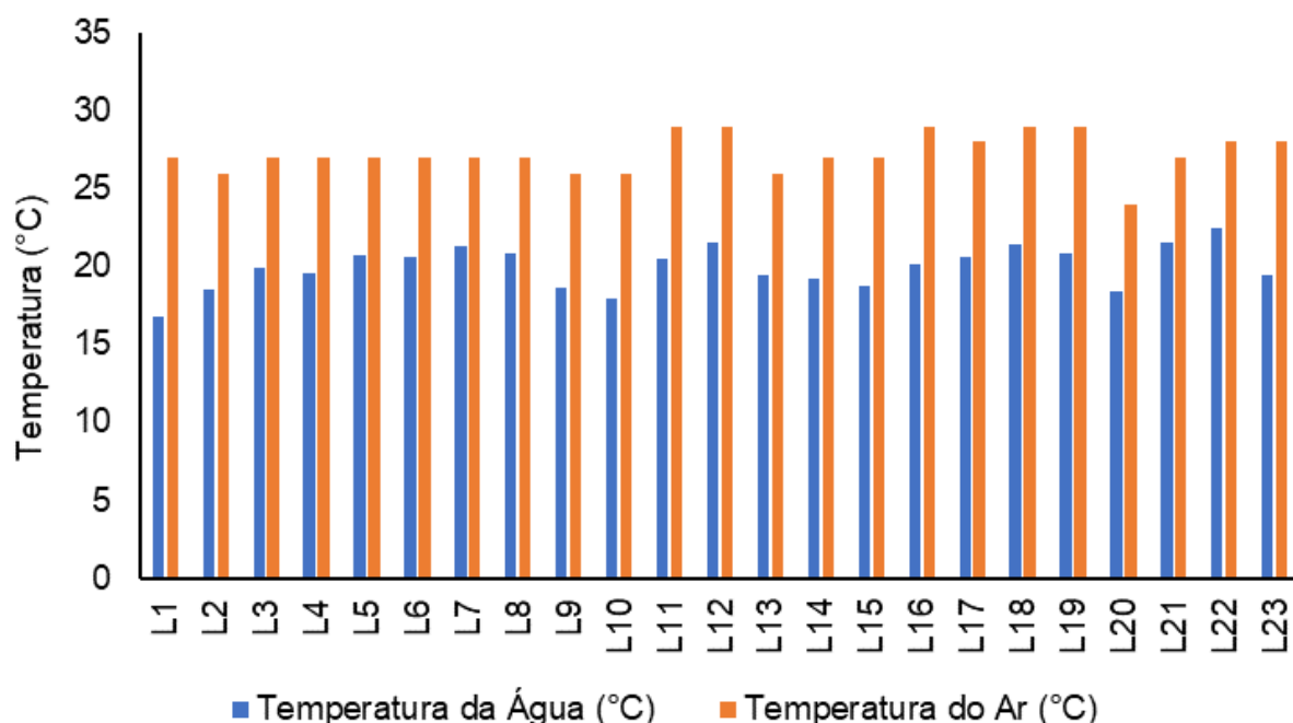
Figura V-50. Distribuição de temperatura do ar e da água na Sub-bacia Leste durante a campanha de julho de 2023.
