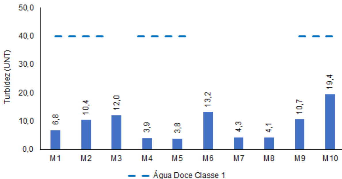
Figura V-7. Distribuição de turbidez na Sub-bacia do Sistema Lagunar de Maricá durante a campanha de julho de 2023.
