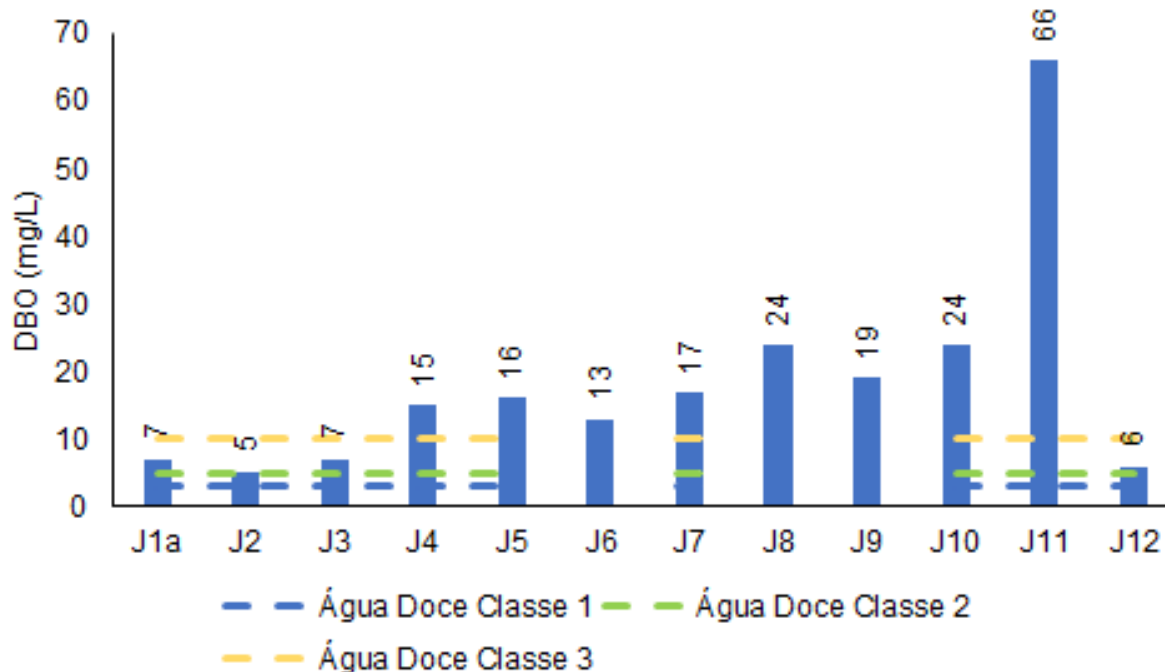
Figura V-16. Distribuição de DBO na Sub-bacia do Sistema Lagunar de Jacarepaguá durante a campanha de julho de 2023.
