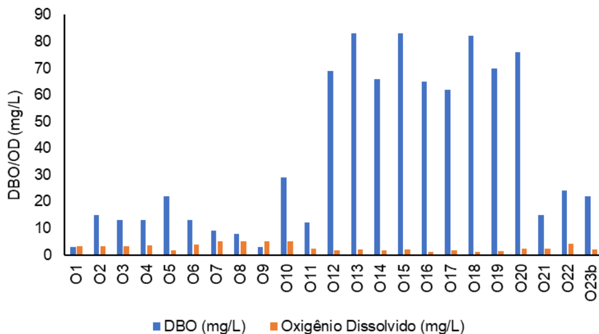
Figura V-65. Comparativo de OD e DBO na Sub-bacia Oeste durante a campanha de julho de 2023.
