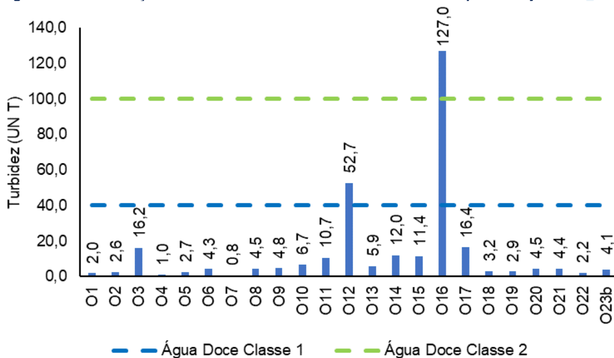
Figura V-67. Distribuição de turbidez na Sub-bacia Oeste durante a campanha de julho de 2023.
