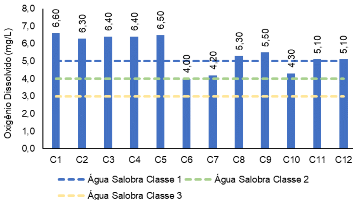
Figura V-39. Distribuição de oxigênio dissolvido na Sub-bacia do Sistema Lagunar Itaipu-Piratininga durante a campanha de julho de 2023.
