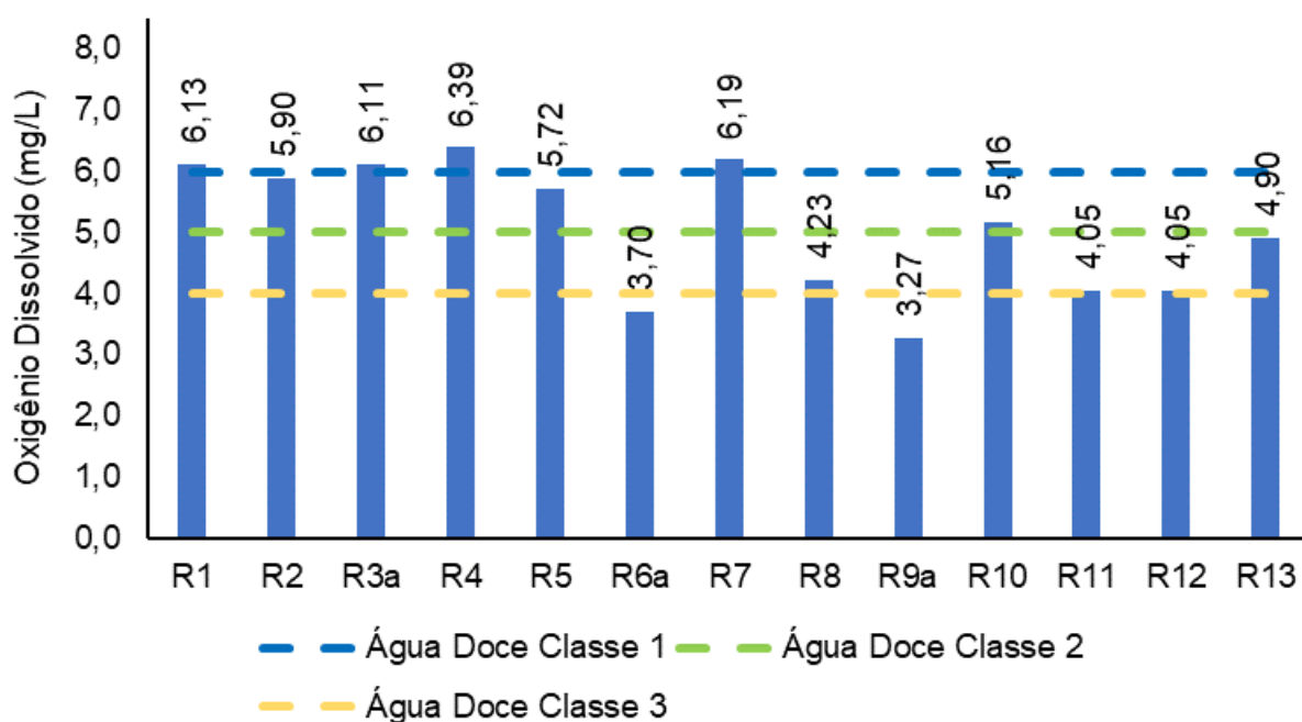
Figura V-27. Distribuição de oxigênio dissolvido na Bacia da Lagoa Rodrigo de Freitas durante a campanha de julho de 2023.
