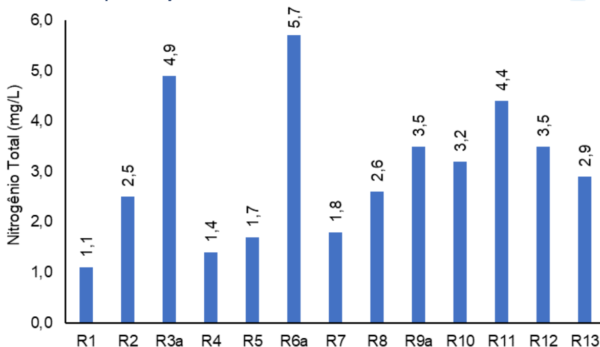
Figura V-34. Distribuição de nitrogênio total na Bacia da Lagoa Rodrigo de Freitas durante a campanha de julho de 2023.
