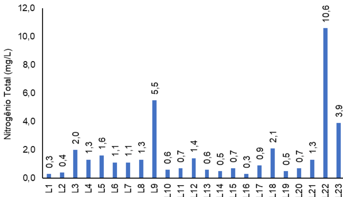
Figura V-58. Distribuição de nitrogênio total na Sub-bacia Leste durante a campanha de julho de 2023.
