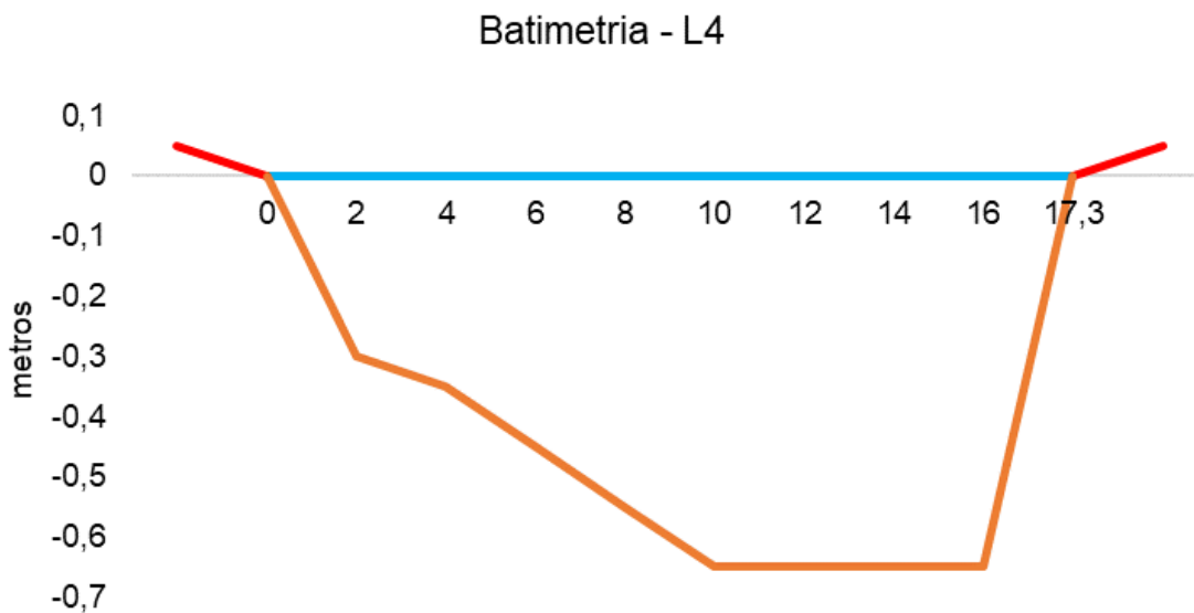
Figura V-80. Desenho esquemático da batimetria da estação L4 - Rio Macacu.
