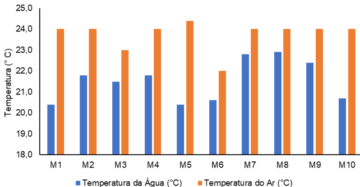
Figura V-2. Distribuição de temperatura do ar e da água na Sub-bacia do Sistema Lagunar de Maricá durante a campanha de julho de 2023.
