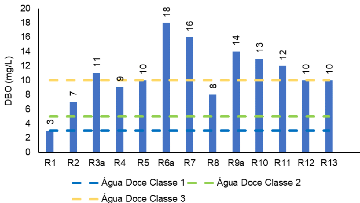
Figura V-28. Distribuição de DBO na Bacia da Lagoa Rodrigo de Freitas durante a campanha de julho de 2023.
