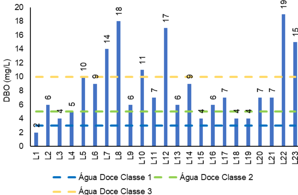
Figura V-52. Distribuição de DBO na Sub-bacia Leste durante a campanha de julho de 2023.
