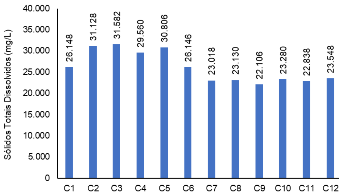
Figura V-47. Distribuição de STD na Sub-bacia do Sistema Lagunar Itaipu-Piratininga durante a campanha de julho de 2023.
