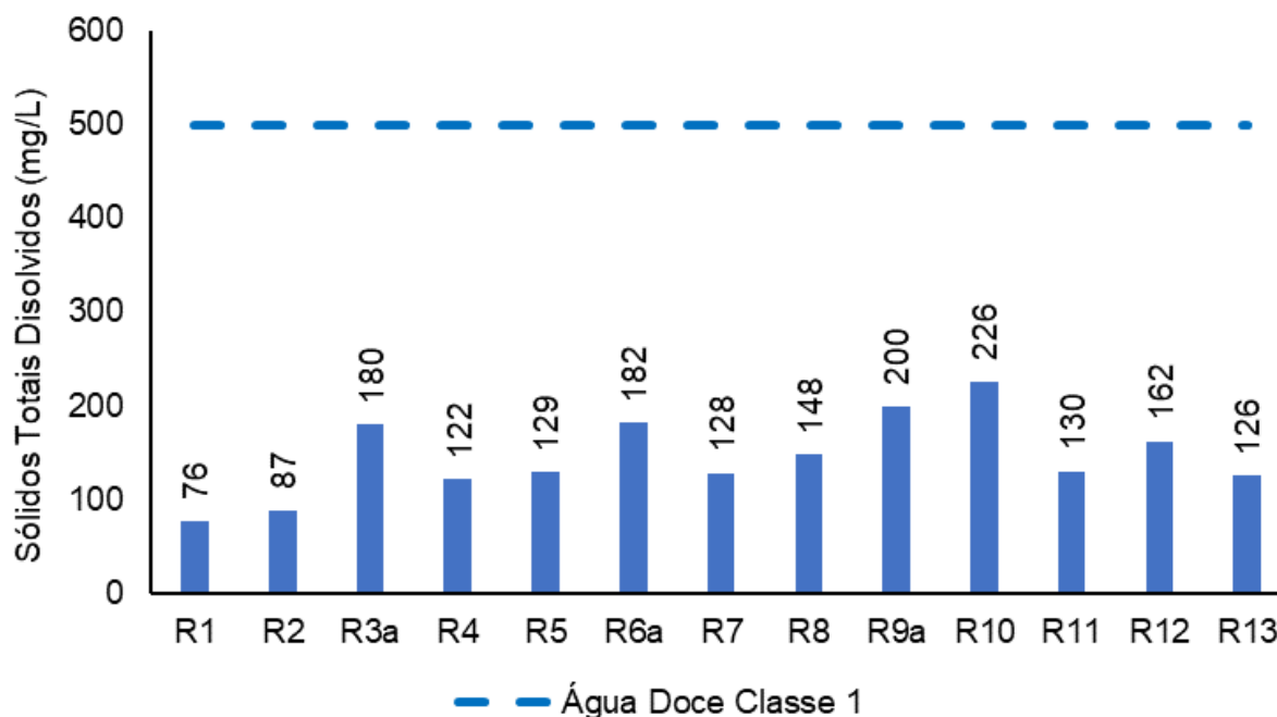
Figura V-35. Distribuição de STD na Bacia da Lagoa Rodrigo de Freitas durante a campanha de julho de 2023.
