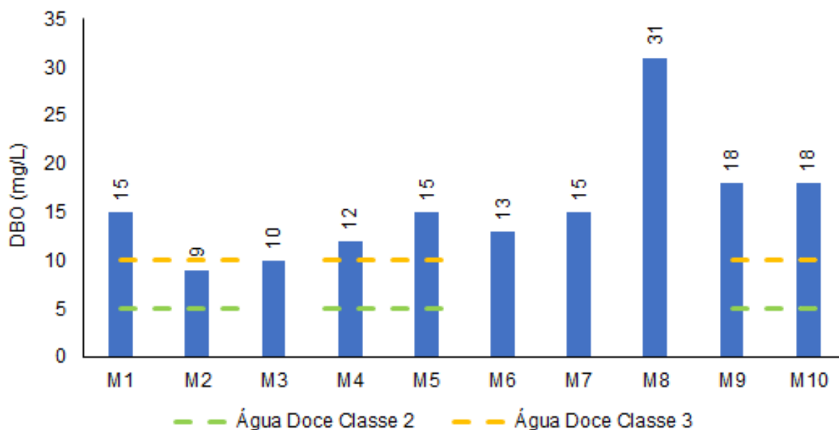
Figura V-4. Distribuição de DBO na Sub-bacia do Sistema Lagunar de Maricá durante a campanha de julho de 2023.
