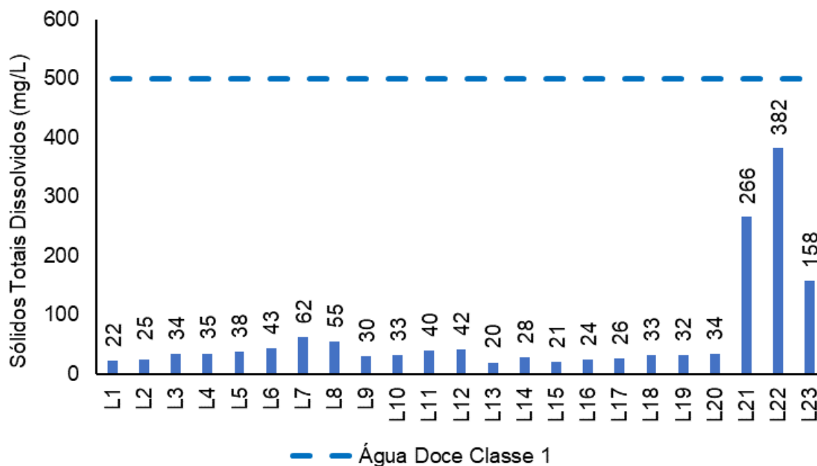
Figura V-59. Distribuição de STD na Sub-bacia Leste durante a campanha de julho de 2023.
