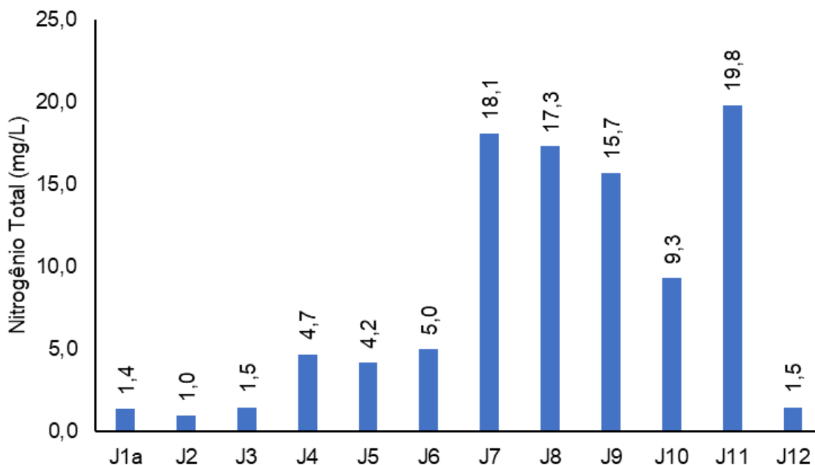
Figura V-22. Distribuição de nitrogênio total na Sub-bacia do Sistema Lagunar de Jacarepaguá durante a campanha de julho de 2023.
