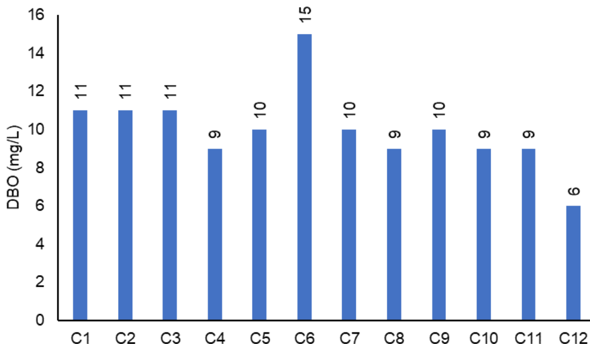
Figura V-40. Distribuição de DBO na Sub-bacia do Sistema Lagunar Itaipu-Piratininga durante a campanha de julho de 2023.
