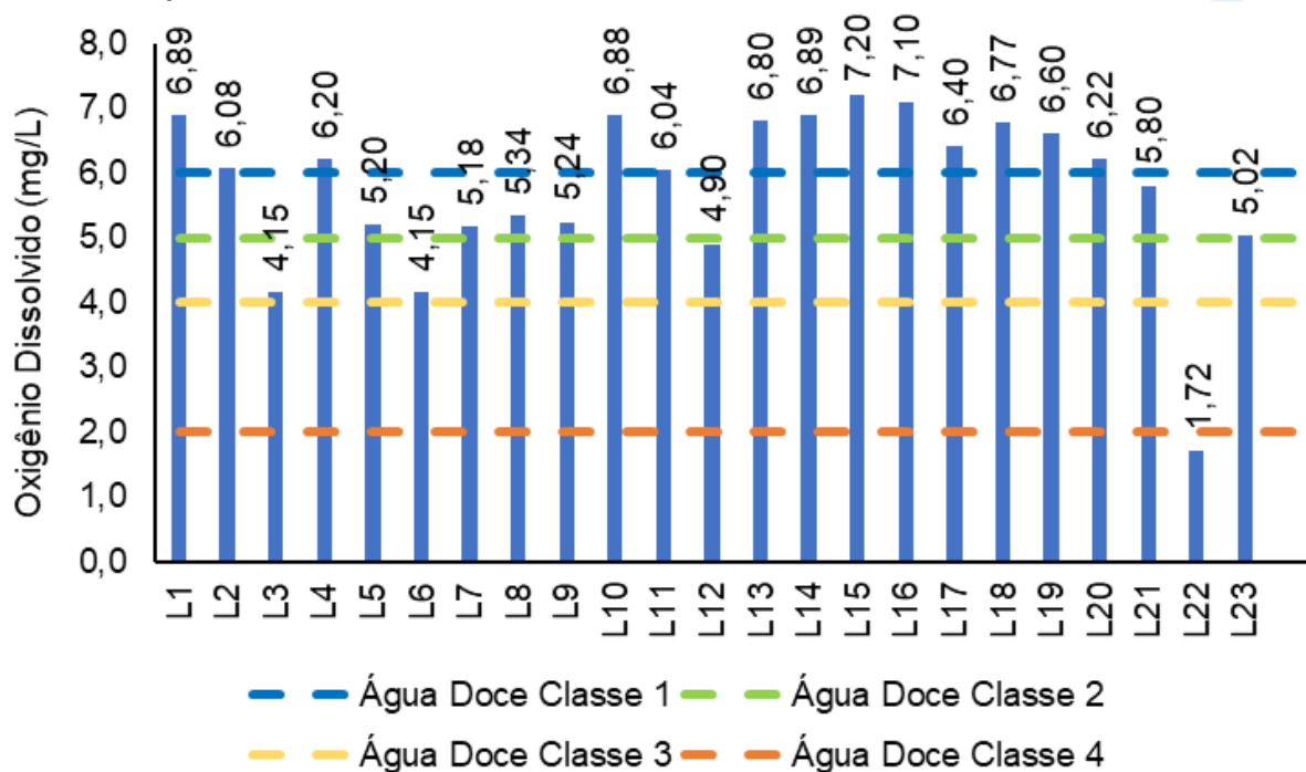
Figura V-51. Distribuição de oxigênio dissolvido na Sub-bacia Leste durante a campanha de julho de 2023.
