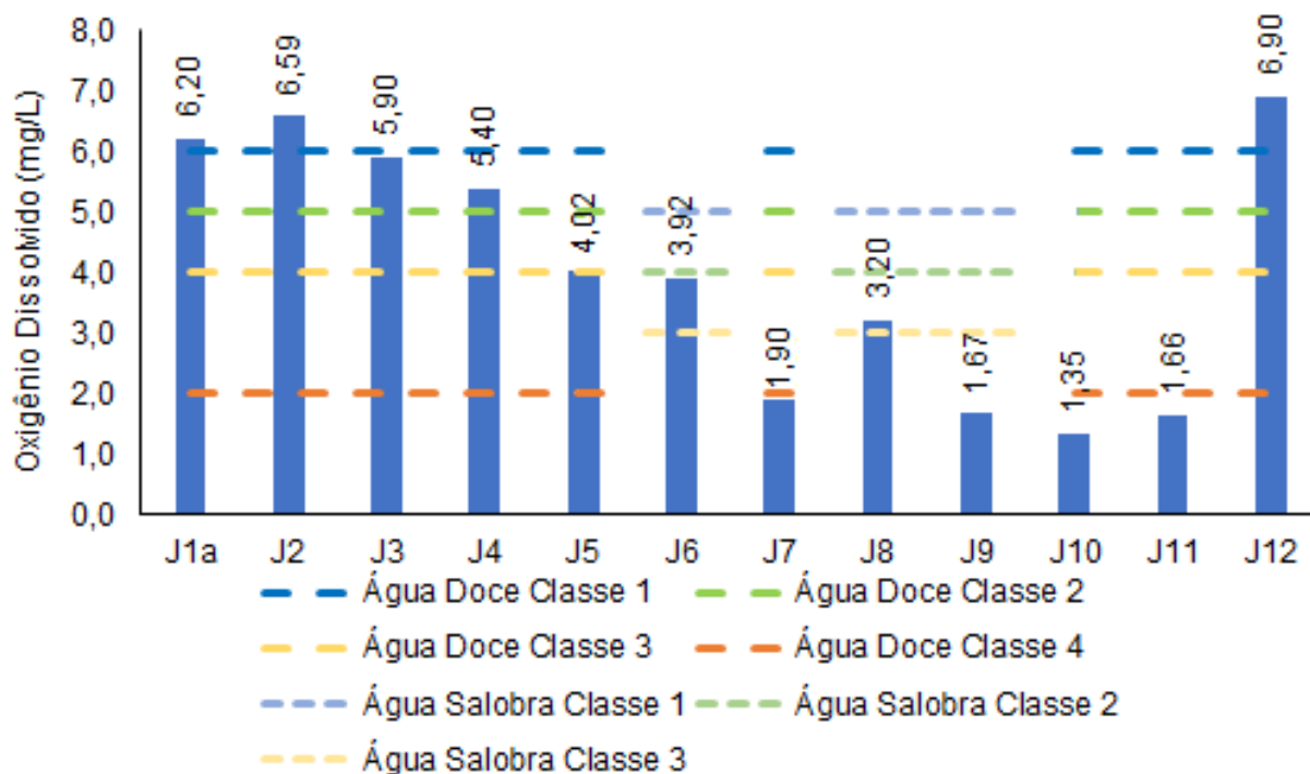
Figura V-15. Distribuição de oxigênio dissolvido na Sub-bacia do Sistema Lagunar de Jacarepaguá durante a campanha de julho de 2023.
