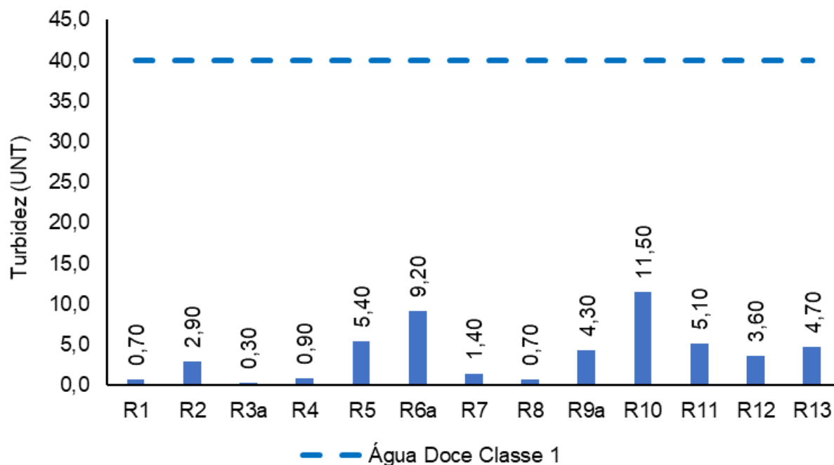
Figura V-31. Distribuição de turbidez na Bacia da Lagoa Rodrigo de Freitas durante a campanha de julho de 2023.
