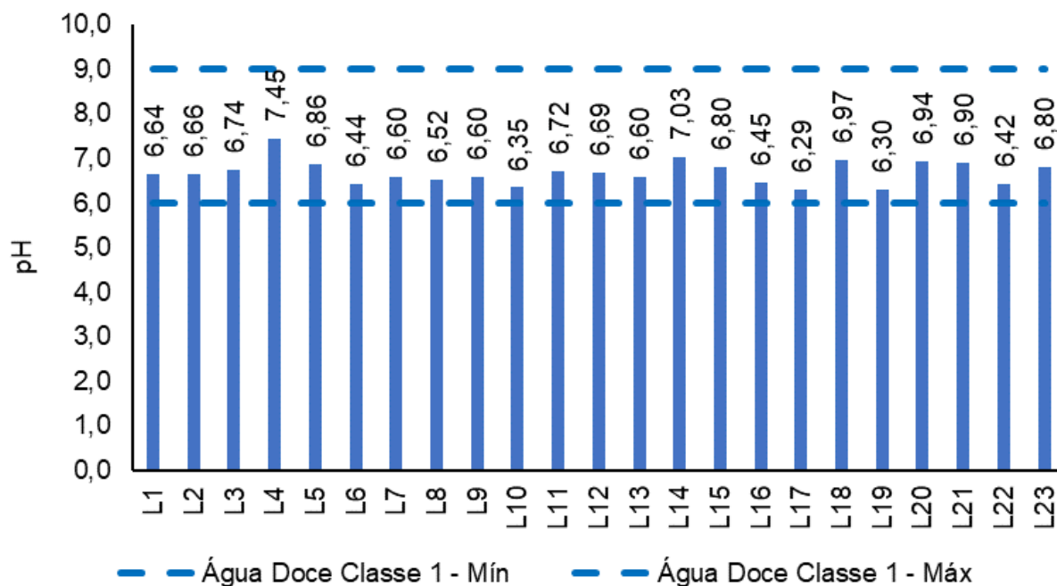
Figura V-54. Distribuição de pH na Sub-bacia Leste durante a campanha de julho de 2023.
