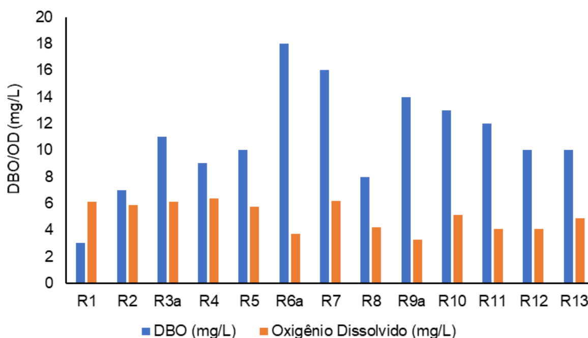
Figura V-29. Comparativo entre disponibilidade de OD e DBO na Bacia da Lagoa Rodrigo de Freitas durante a campanha de julho de 2023.
