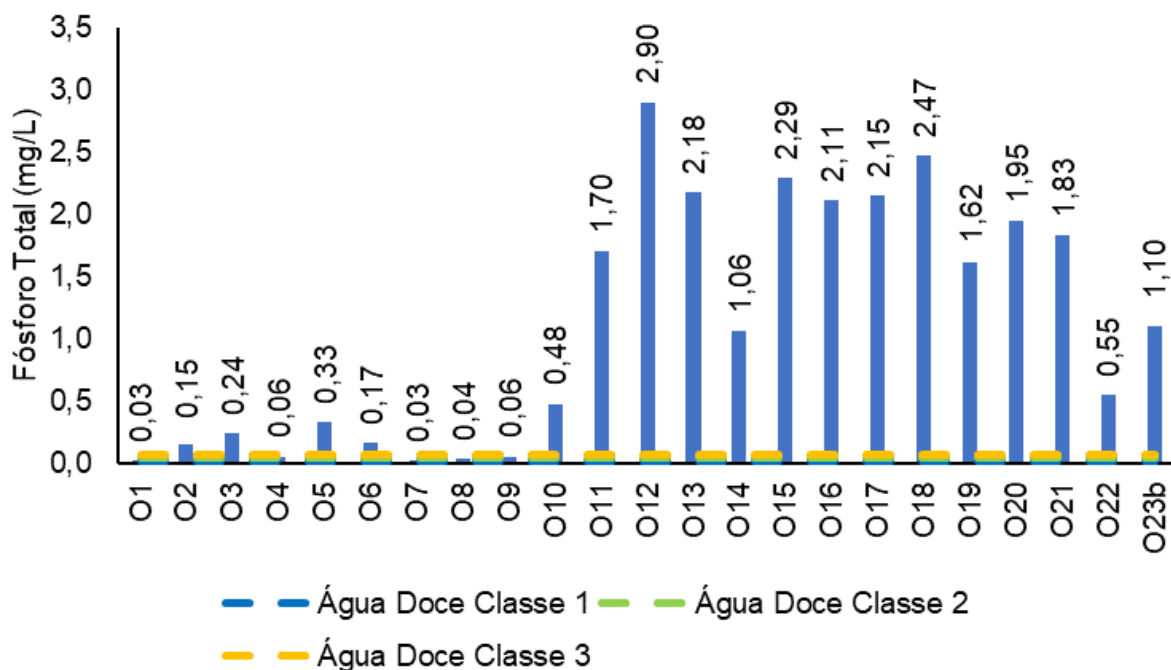
Figura V-68. Distribuição de fósforo total na Sub-bacia Oeste durante a campanha de julho de 2023.
