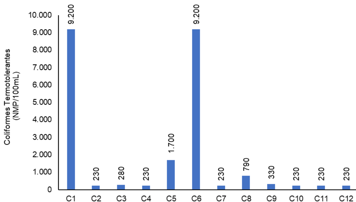
Figura V-48. Distribuição de coliformes termotolerantes na Sub-bacia do Sistema Lagunar Itaipu-Piratininga durante a campanha de julho de 2023.
