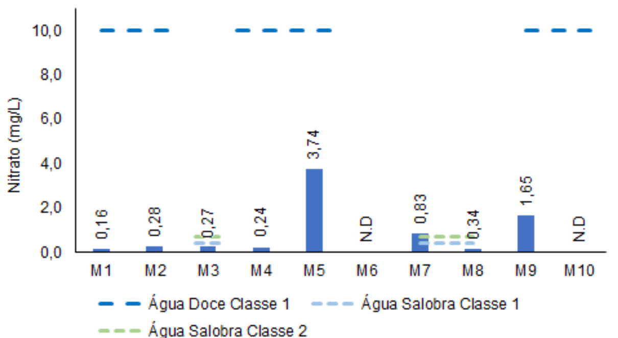
Figura V-9. Distribuição de nitrato na Sub-bacia do Sistema Lagunar de Maricá durante a campanha de julho de 2023.
