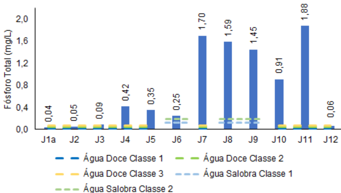
Figura V-20. Distribuição de fósforo total na Sub-bacia do Sistema Lagunar de Jacarepaguá durante a campanha de julho de 2023.
