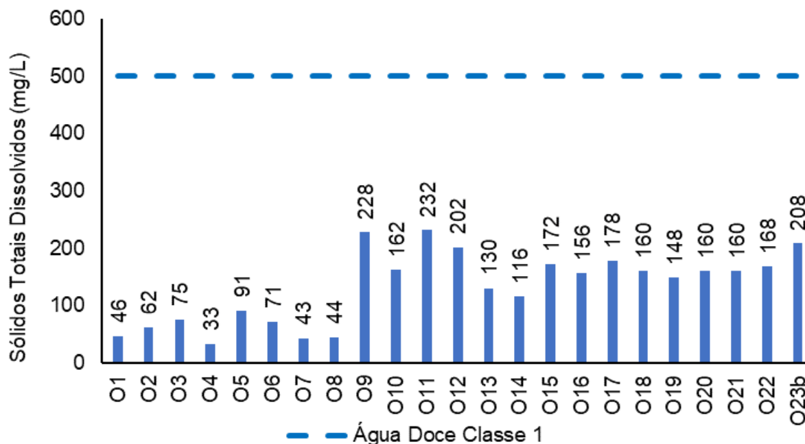
Figura V-71. Distribuição de STD na Sub-bacia Oeste durante a campanha de julho de 2023.
