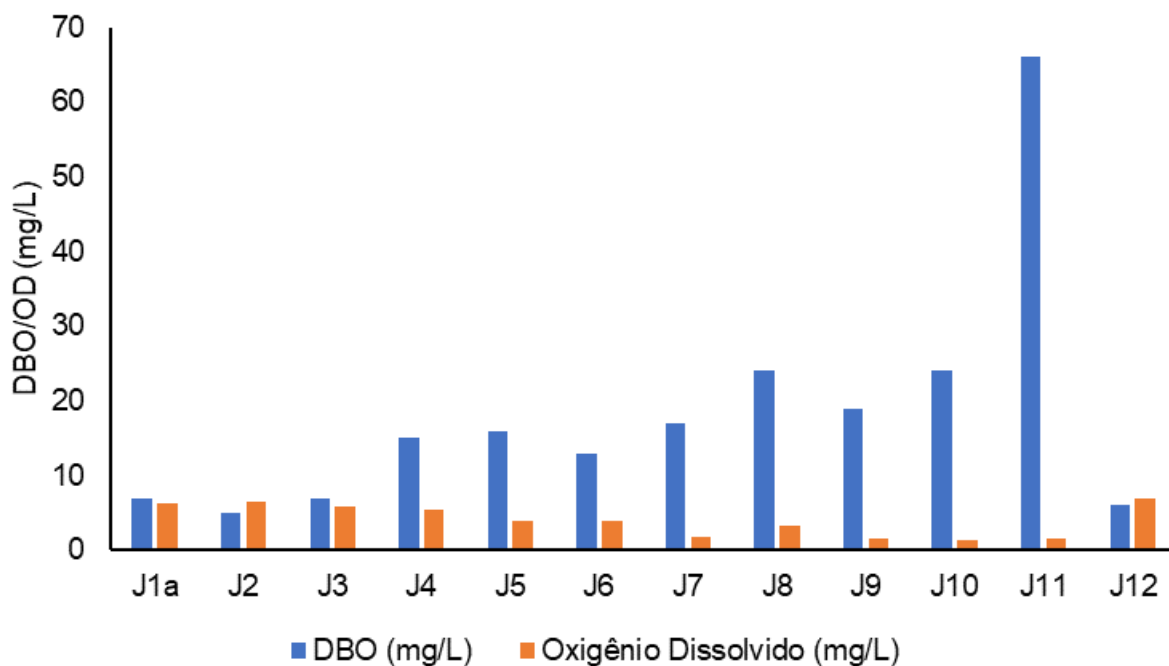
Figura V-17. Comparativo entre disponibilidade de OD e DBO na Sub-bacia do Sistema Lagunar de Jacarepaguá durante a campanha de julho de 2023.
