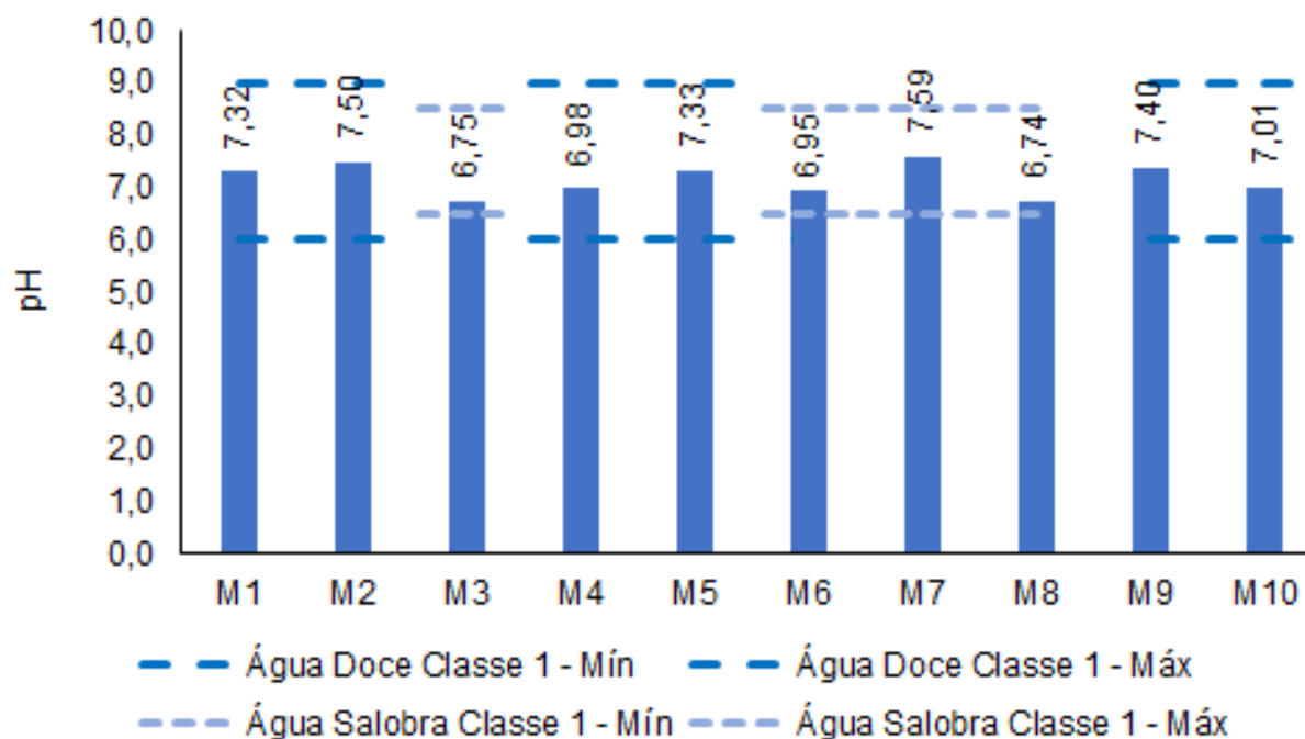
Figura V-6. Distribuição de pH na Sub-bacia do Sistema Lagunar de Maricá durante a campanha de julho de 2023.
