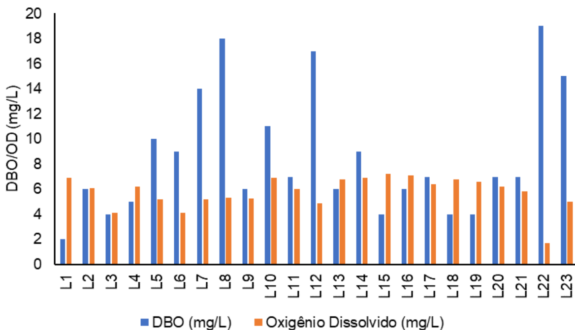
Figura V-53. Comparativo da concentração de OD e DBO na Sub-bacia Leste durante a campanha de julho de 2023.
