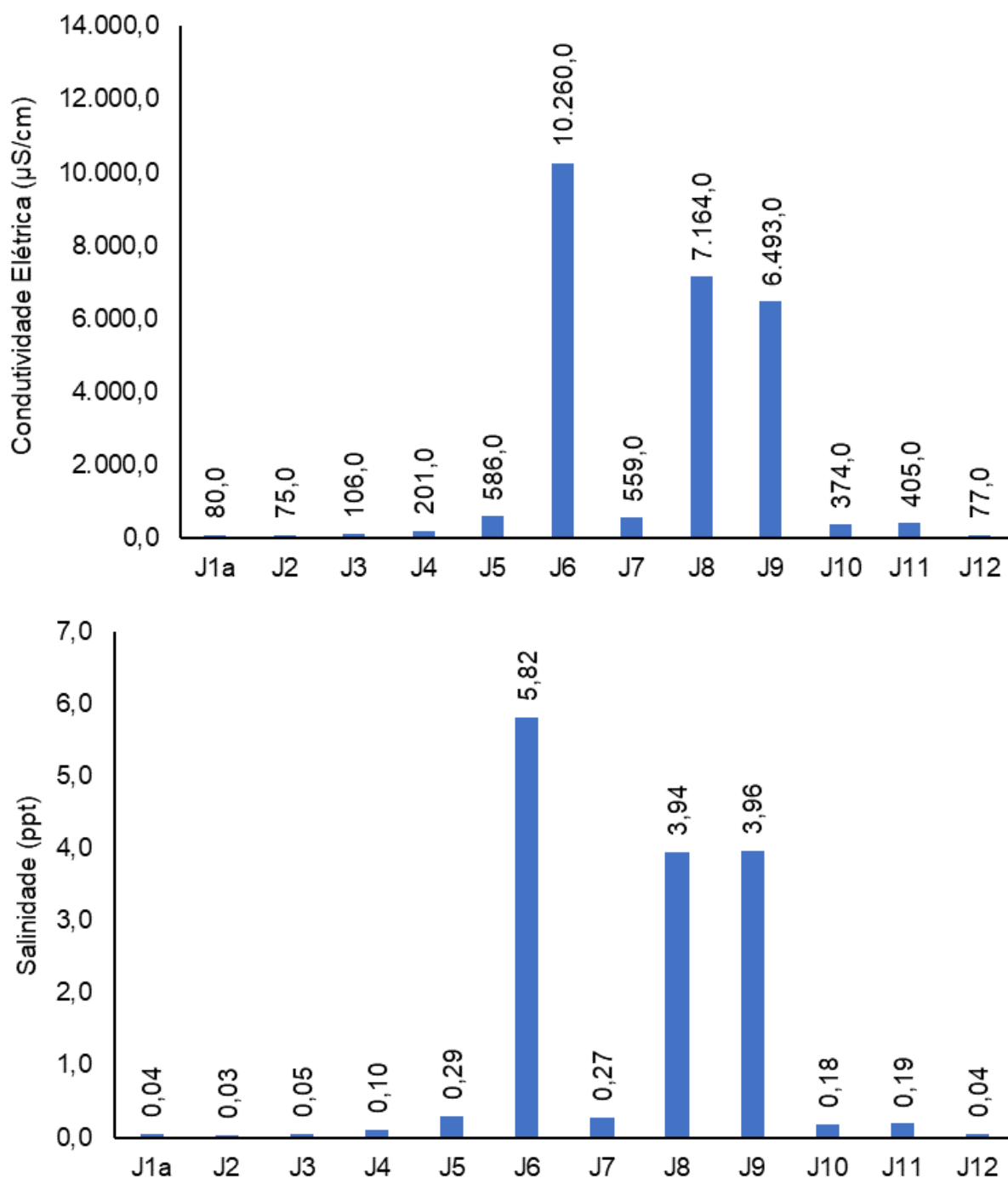
Figura V-13. Distribuição de condutividade e salinidade na Sub-bacia do Sistema Lagunar de Jacarepaguá durante a campanha de julho de 2023.
