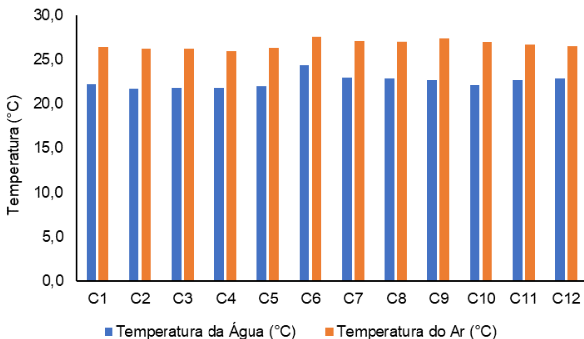
Figura V-38. Distribuição de temperatura do ar e da água na Sub-bacia do Sistema Lagunar Itaipu-Piratininga durante a campanha de julho de 2023.
