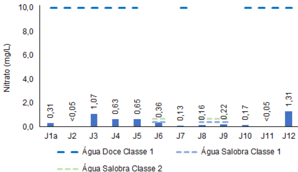
Figura V-21. Distribuição de nitrato na Sub-bacia do Sistema Lagunar de Jacarepaguá durante a campanha de julho de 2023.
