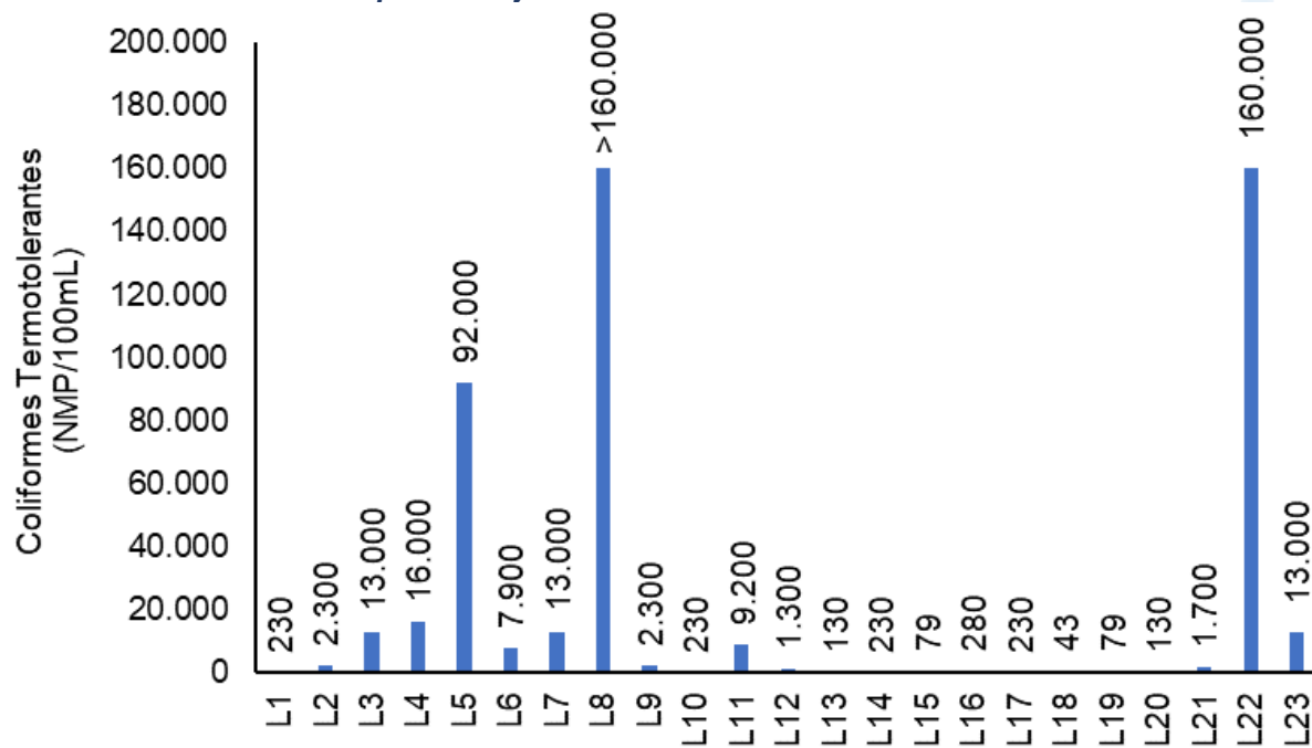
Figura V-60. Distribuição de coliformes termotolerantes na região Leste da Baía de Guanabara durante a campanha de julho de 2023.
