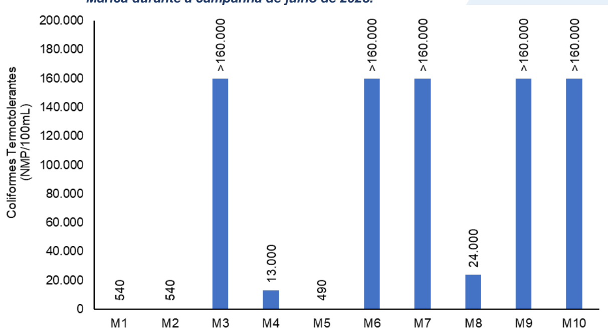
Figura V-12. Distribuição de coliformes termotolerantes na Sub-bacia do Sistema Lagunar de Maricá durante a campanha de julho de 2023.
