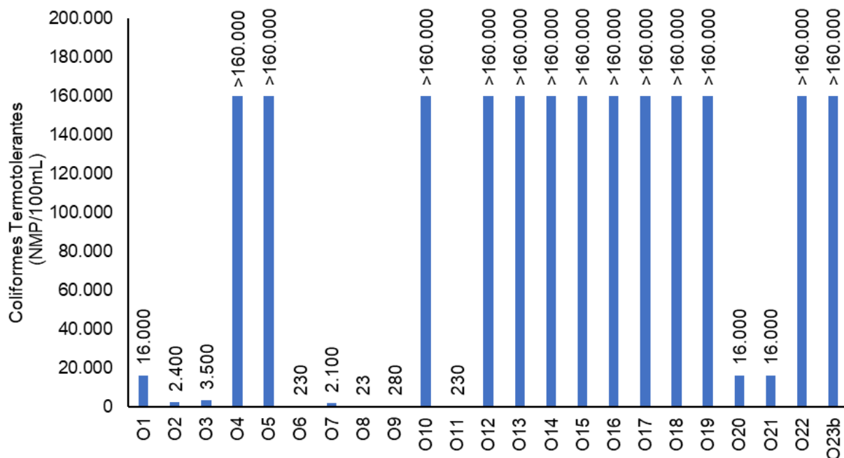
Figura V-72. Distribuição de coliformes termotolerantes na região Oeste durante a campanha de julho de 2023.
