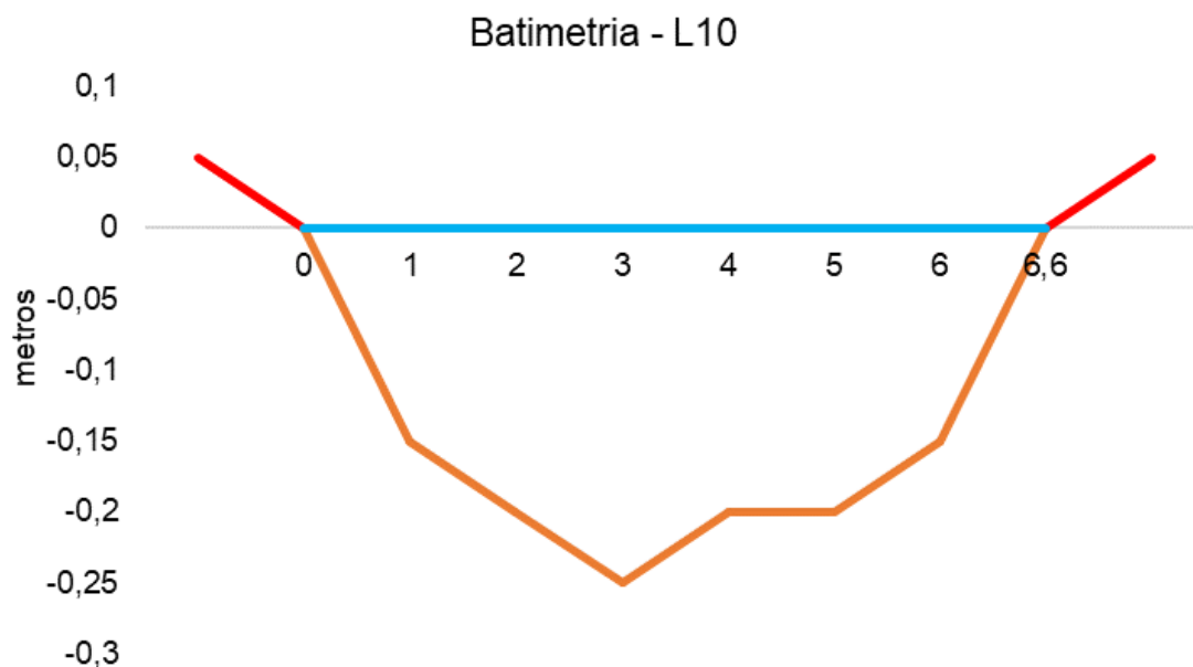
Figura V-84. Desenho esquemático da batimetria da estação L10 - Rio Rabelo.
