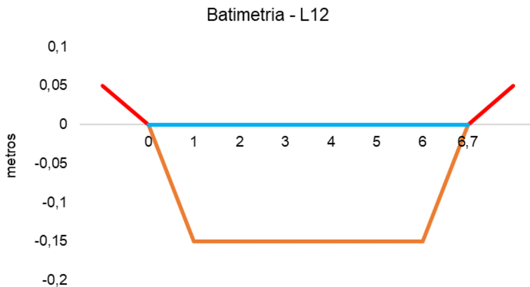
Figura V-85. Desenho esquemático da batimetria da estação L12 - Rio Rabelo.
