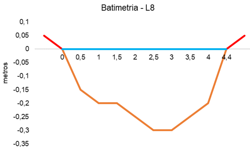
Figura V-83. Desenho esquemático da batimetria da estação L8 - Papucainha.
