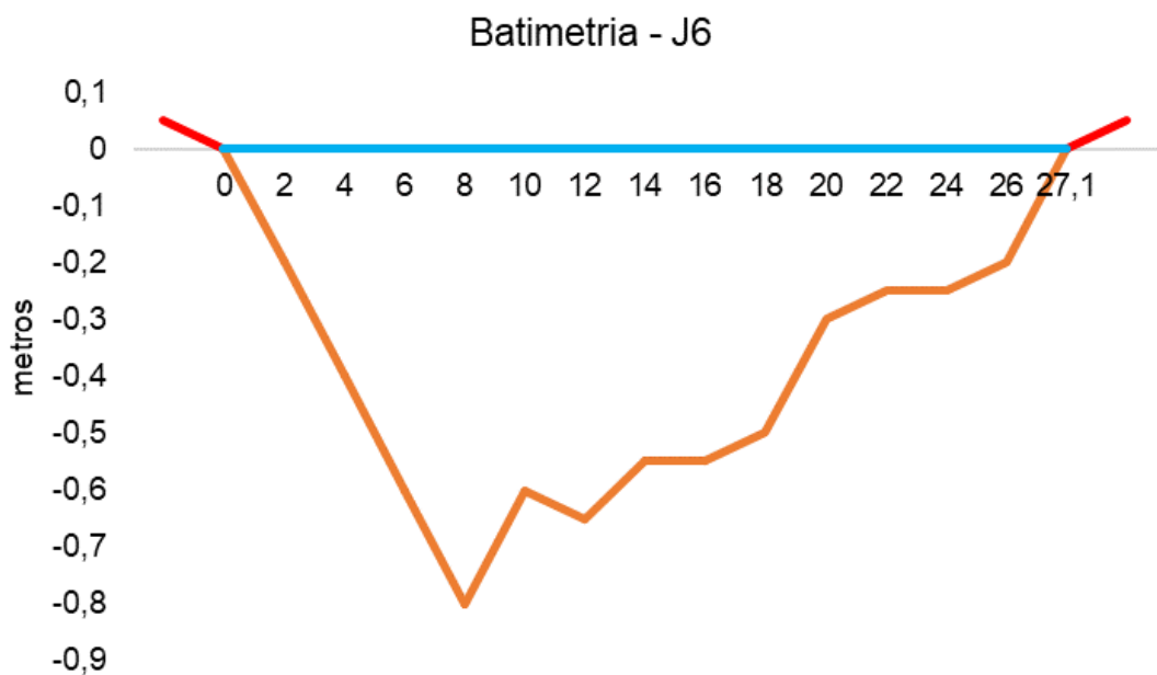
Figura V-75. Desenho esquemático da batimetria da estação J6 - Canal de Sernambetiba.
