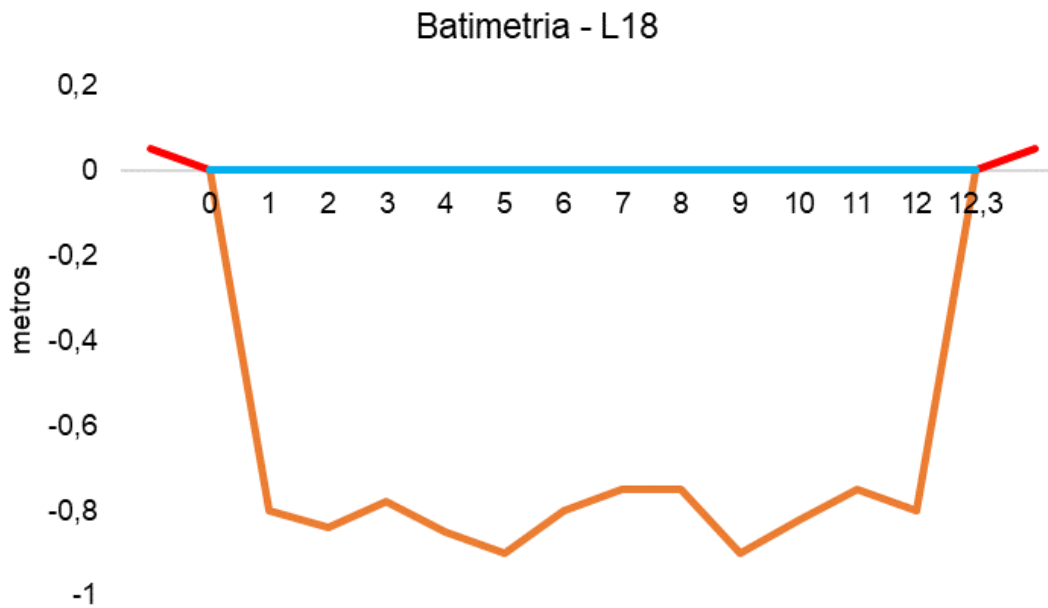
Figura V-93. Desenho esquemático da batimetria da estação L18 - Rio Guapiaçu.
