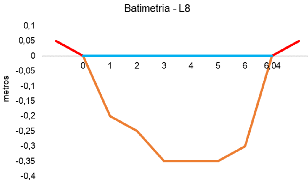
Figura V-86. Desenho esquemático da batimetria da estação L8 - Papucainha.
