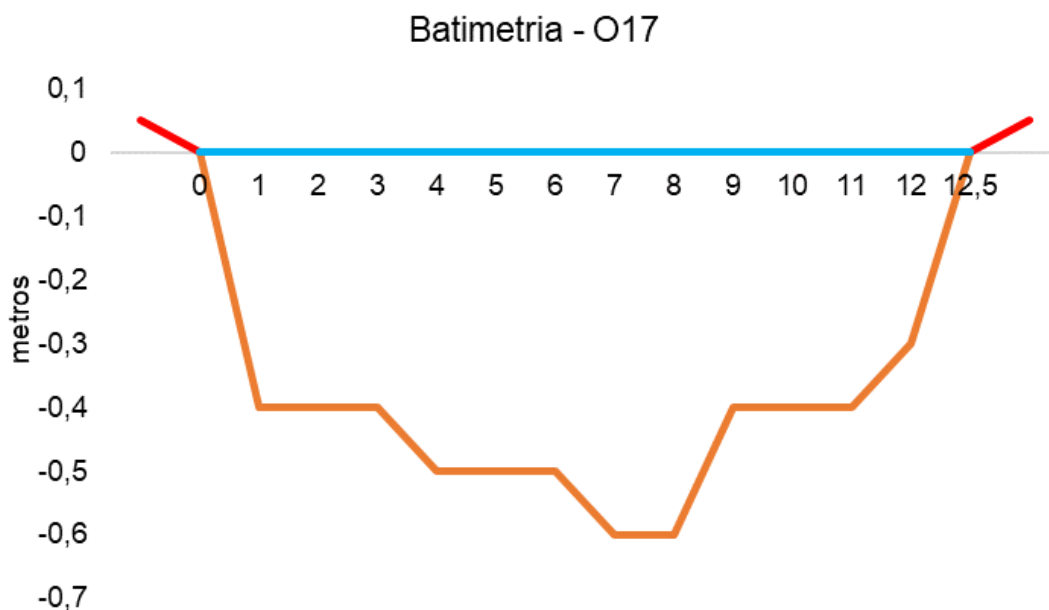
Figura V-111. Desenho esquemático da batimetria da estação O17 - Rio Sarapuí.
