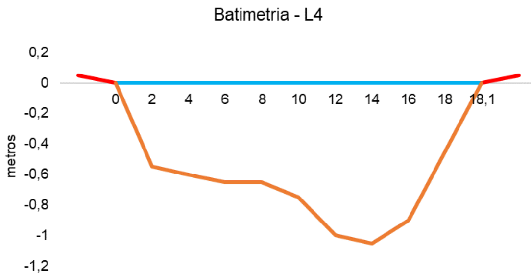
Figura V-83. Desenho esquemático da batimetria da estação L4 - Rio Macacu.
