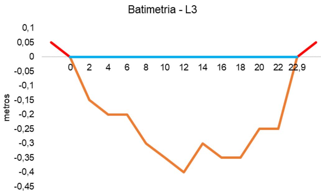
Figura V-82. Desenho esquemático da batimetria da estação L3 - Rio Macacu.
