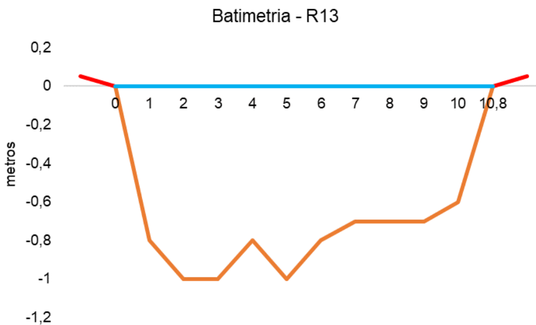
Figura V-79. Desenho esquemático da batimetria da estação R13 - Rio Rainha.
