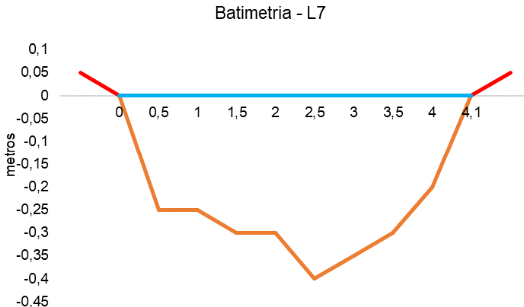
Figura V-85. Desenho esquemático da batimetria da estação L7 - Rio Cassiano.
