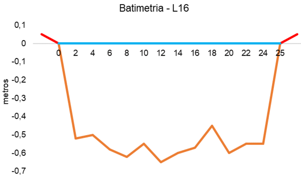
Figura V-92. Desenho esquemático da batimetria da estação L16 - Rio Guapiaçu.
