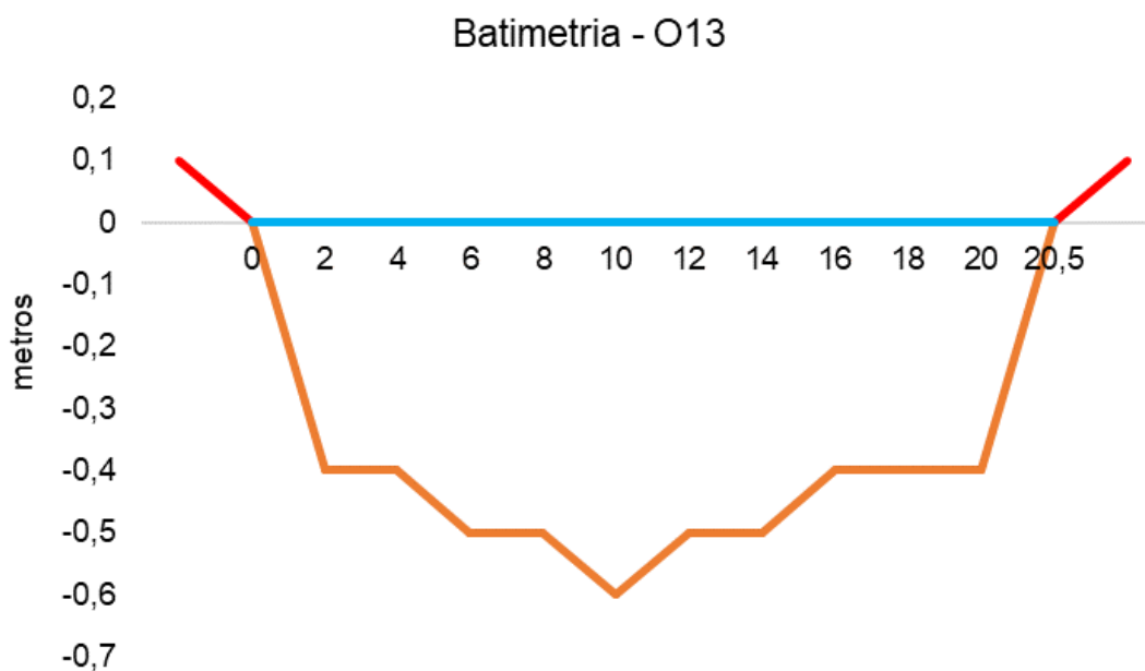
Figura V-108. Desenho esquemático da batimetria da estação O13 - Rio Botas.
