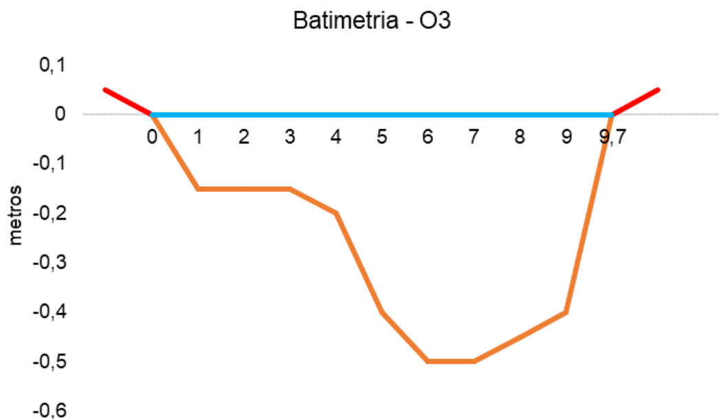
Figura V-99. Desenho esquemático da batimetria da estação O3 - Rio Saracuruna.
