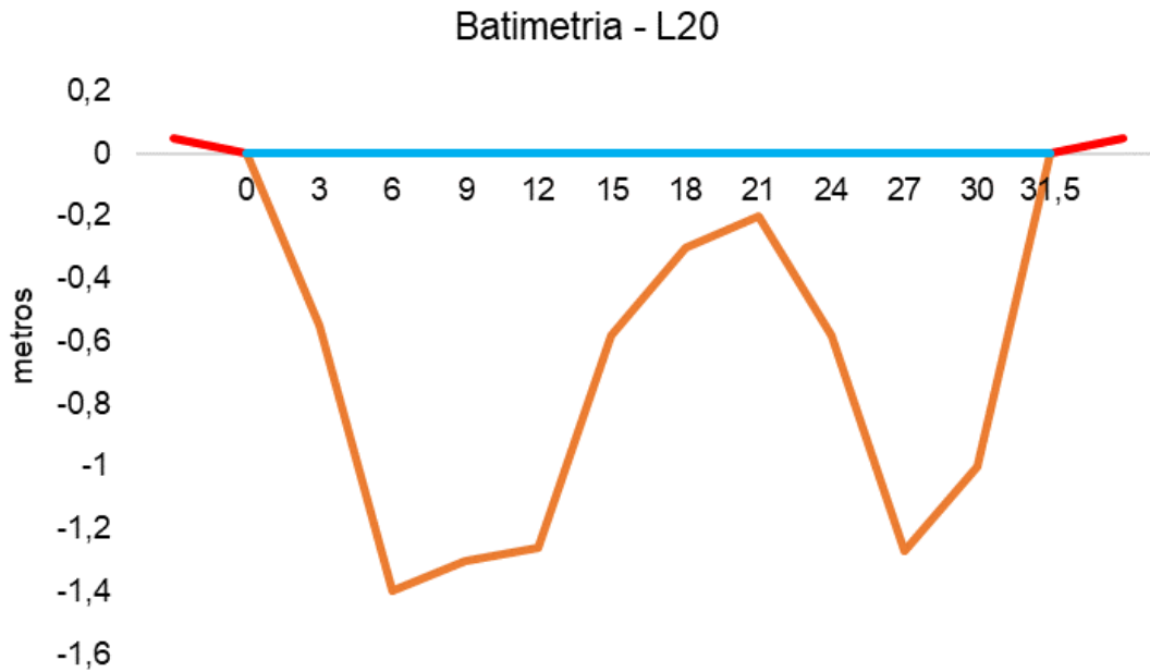
Figura V-95. Desenho esquemático da batimetria da estação L20 - Rio Guapiaçu.
