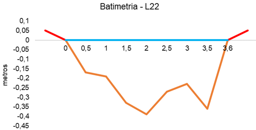
Figura V-96. Desenho esquemático da batimetria da estação L22 - Afluente do Rio Caceribu.
