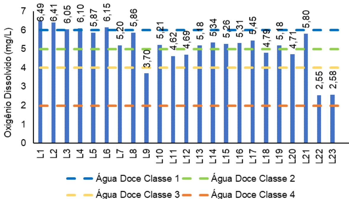
Figura V-51. Distribuição de oxigênio dissolvido na Sub-bacia Leste durante a campanha de junho de 2023.
