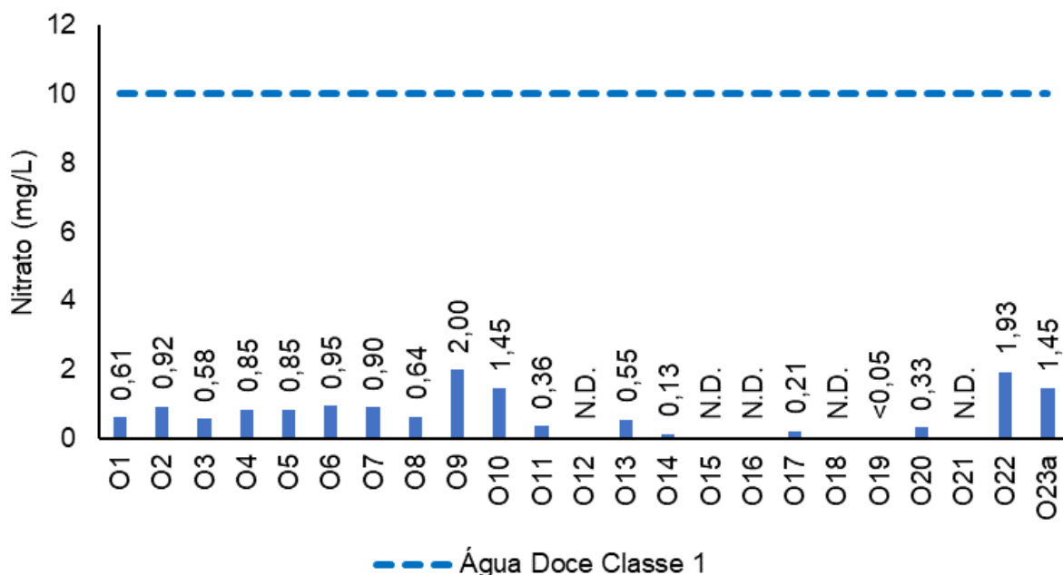
Figura V-69. Distribuição de nitrato na Sub-bacia Oeste durante a campanha de junho de 2023.
