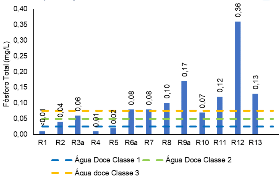
Figura V-32. Distribuição de fósforo total na Bacia da Lagoa Rodrigo de Freitas durante a campanha de junho de 2023.
