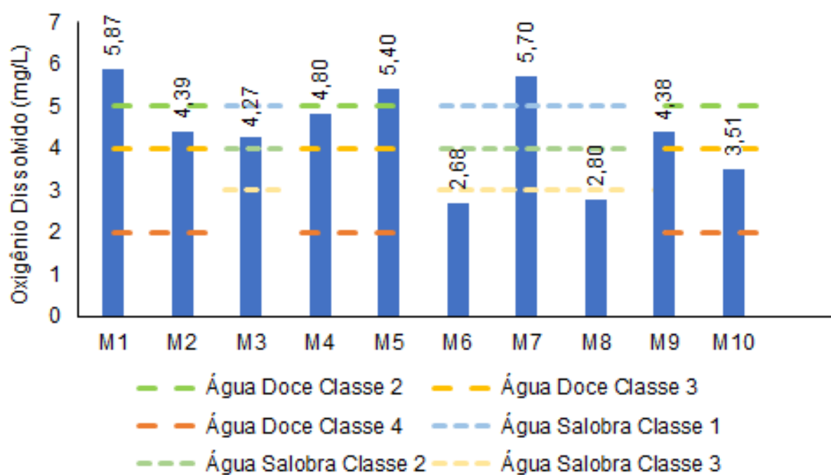
Figura V-3. Distribuição de oxigênio dissolvido na Sub-bacia do Sistema Lagunar de Maricá durante a campanha de junho de 2023.
