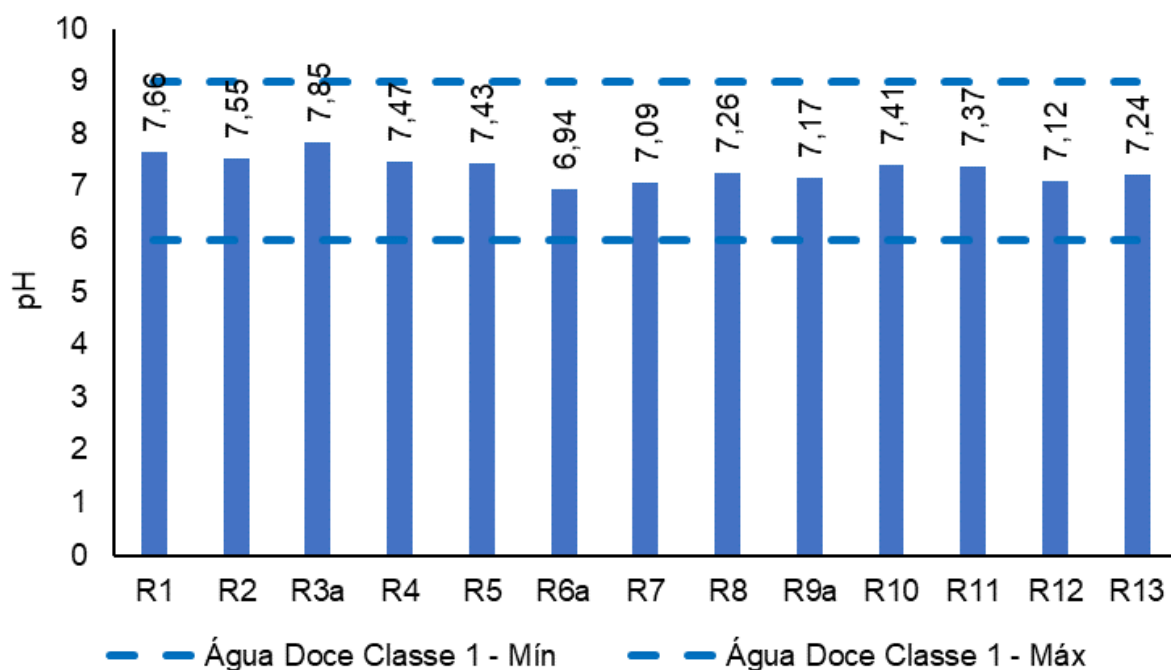
Figura V-30. Distribuição de pH na Bacia da Lagoa Rodrigo de Freitas durante a campanha de junho de 2023.
