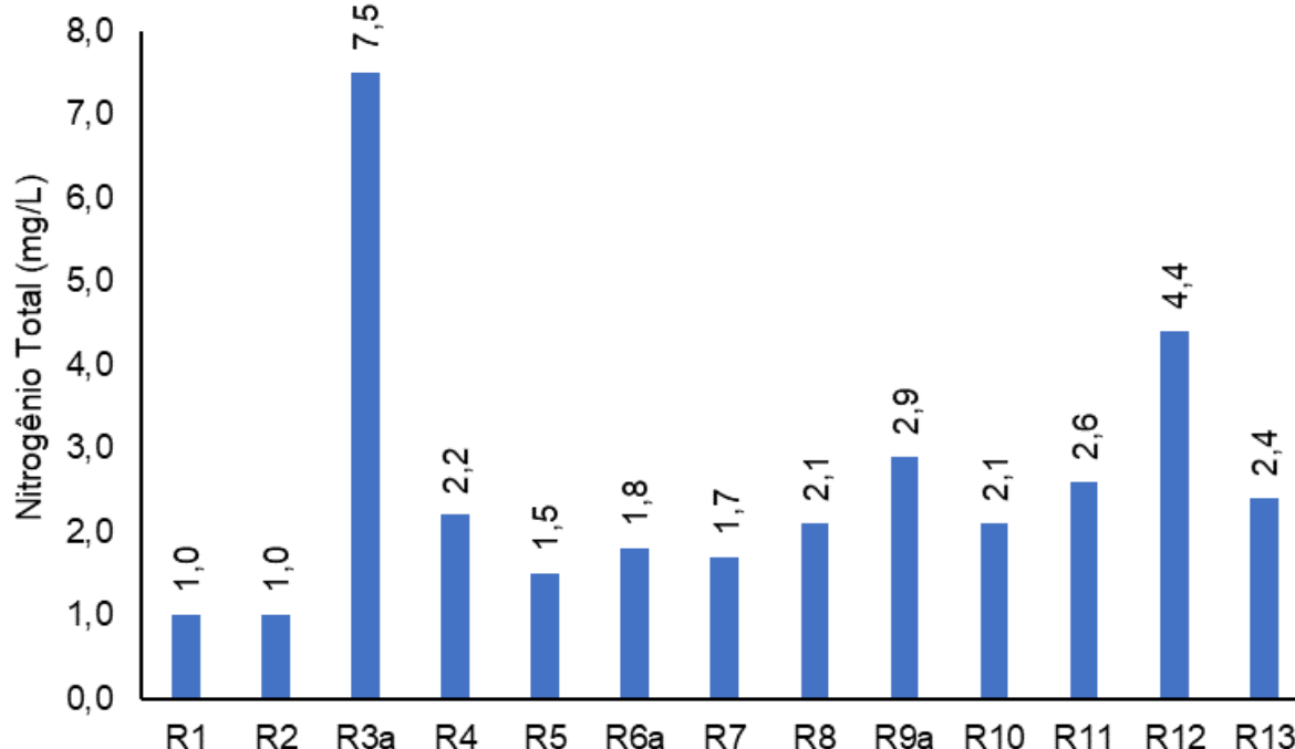
Figura V-34. Distribuição de nitrogênio total na Bacia da Lagoa Rodrigo de Freitas durante a campanha de junho de 2023.
