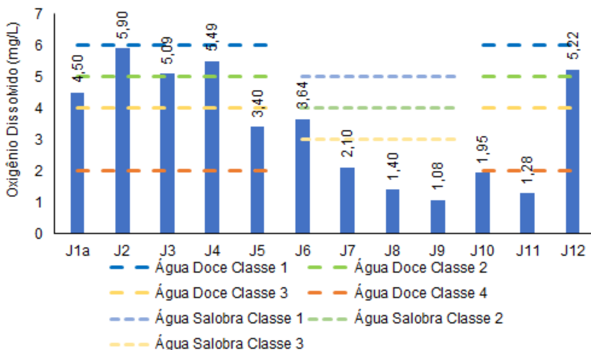
Figura V-15. Distribuição de oxigênio dissolvido na Sub-bacia do Sistema Lagunar de Jacarepaguá durante a campanha de junho de 2023.
