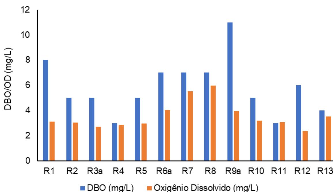
Figura V-29. Comparativo entre disponibilidade de OD e DBO na Bacia da Lagoa Rodrigo de Freitas durante a campanha de junho de 2023.
