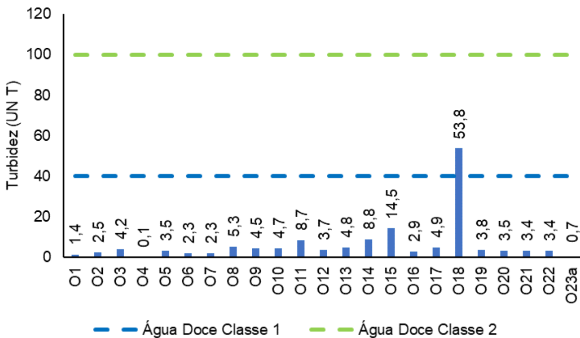
Figura V-67. Distribuição de turbidez na Sub-bacia Oeste durante a campanha de junho de 2023.
