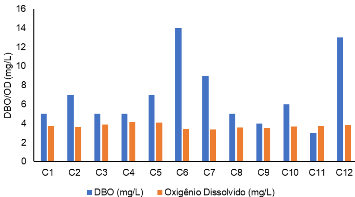
Figura V-41. Comparativo de DBO e OD na Sub-bacia do Sistema Lagunar Itaipu-Piratininga durante a campanha de junho de 2023.
