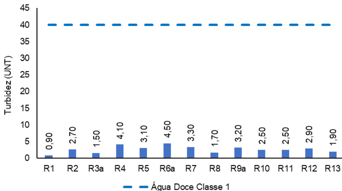
Figura V-31. Distribuição de turbidez na Bacia da Lagoa Rodrigo de Freitas durante a campanha de junho de 2023.
