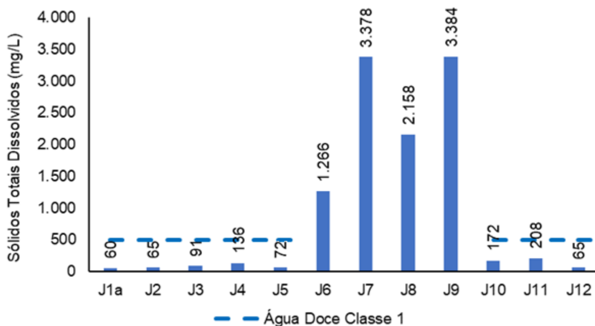
Figura V-23. Distribuição de STD na Sub-bacia do Sistema Lagunar de Jacarepaguá durante a campanha de junho de 2023.
