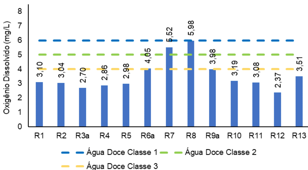
Figura V-27. Distribuição de oxigênio dissolvido na Bacia da Lagoa Rodrigo de Freitas durante a campanha de junho de 2023.
