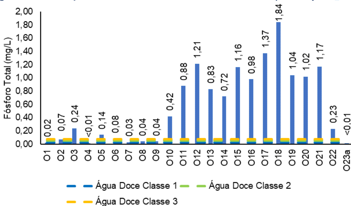
Figura V-68. Distribuição de fósforo total na Sub-bacia Oeste durante a campanha de junho de 2023.
