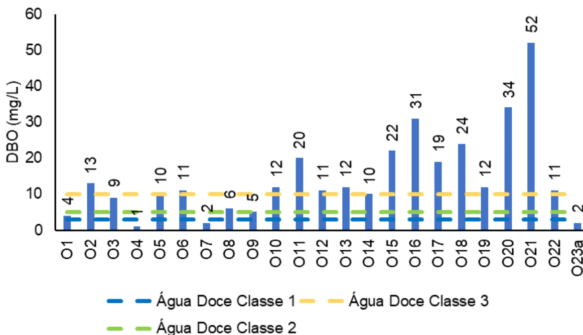
Figura V-64. Distribuição de DBO na Sub-bacia Oeste durante a campanha de junho de 2023.
