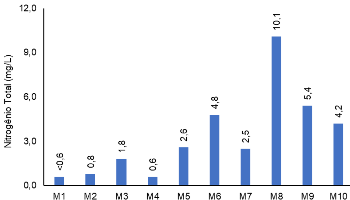
Figura V-10. Distribuição de nitrogênio total na Sub-bacia do Sistema Lagunar de Maricá durante a campanha de junho de 2023.
