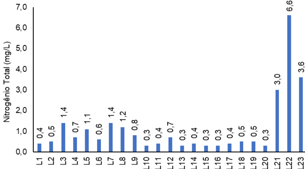
Figura V-58. Distribuição de nitrogênio total na Sub-bacia Leste durante a campanha de junho de 2023.
