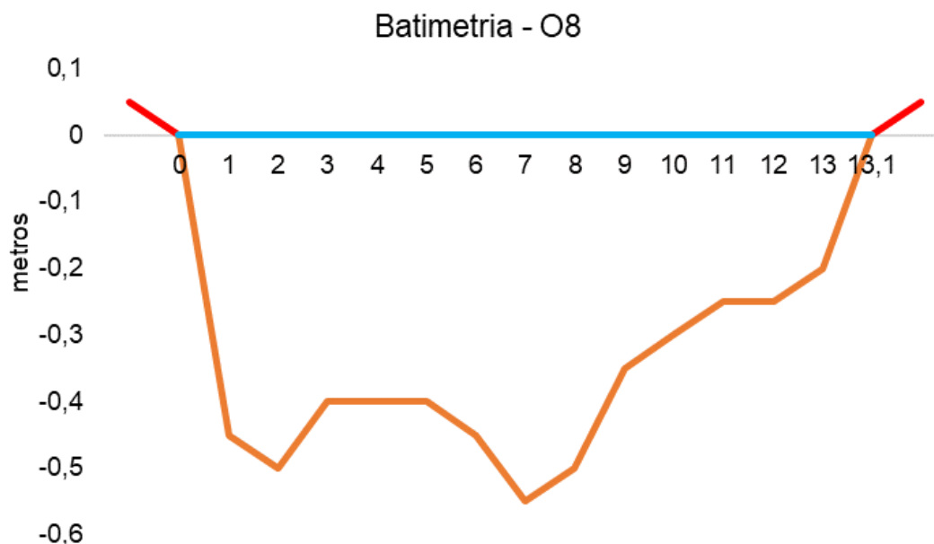
Figura V-103. Desenho esquemático da batimetria da estação O8 - Rio Tinguá.
