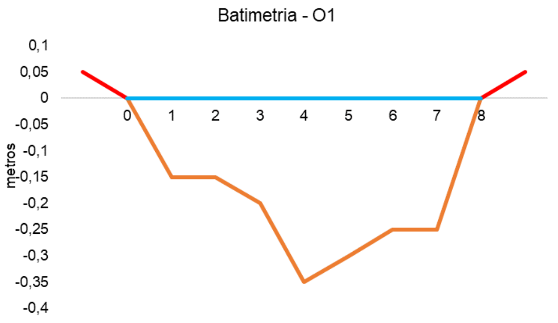
Figura V-98. Desenho esquemático da batimetria da estação O1 - Rio Saracuruna.
