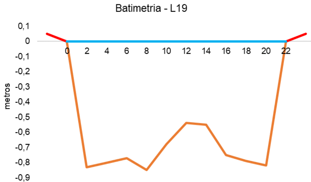
Figura V-94. Desenho esquemático da batimetria da estação L19 - Rio Guapiaçu.
