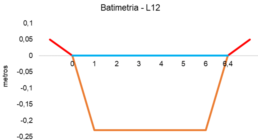
Figura V-88. Desenho esquemático da batimetria da estação L12 - Rio Rabelo.
