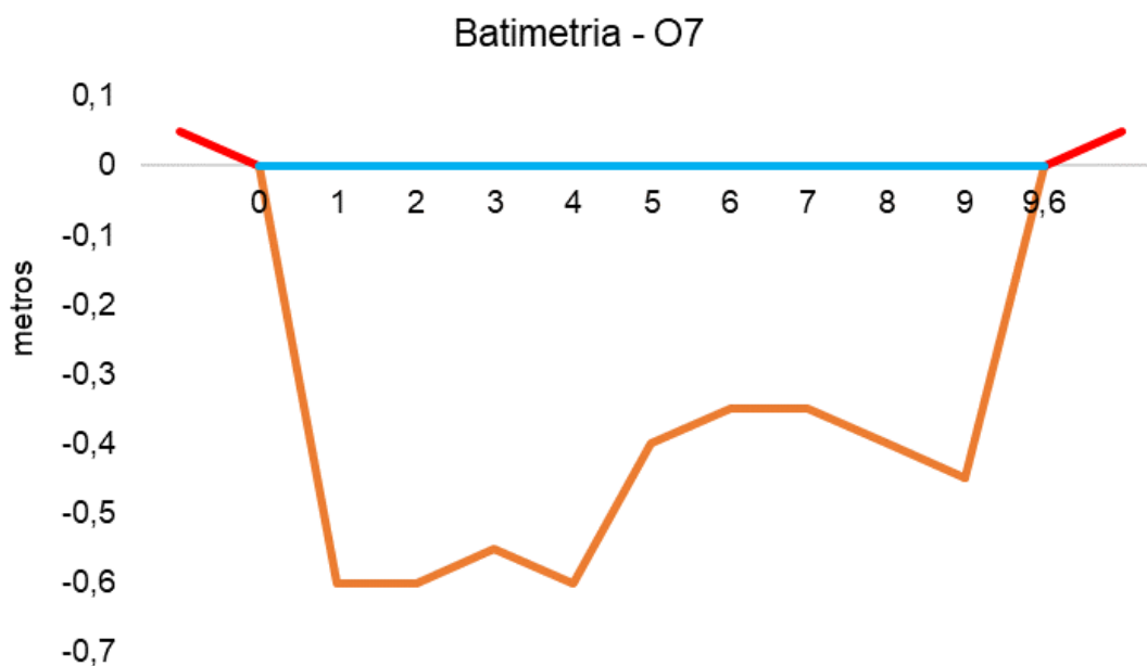
Figura V-102. Desenho esquemático da batimetria da estação O7 - Rio Tinguá.
