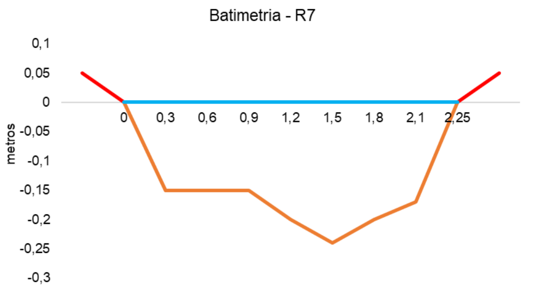
Figura V-77. Desenho esquemático da batimetria da estação R7 - Rio Rainha.
