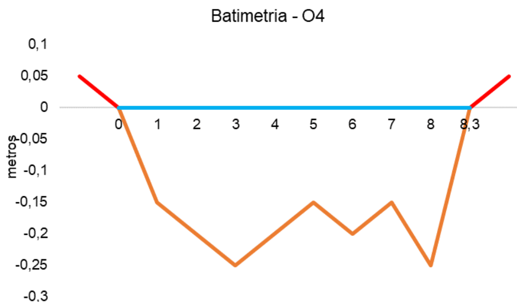
Figura V-100. Desenho esquemático da batimetria da estação O4 - Rio Sapucaia.
