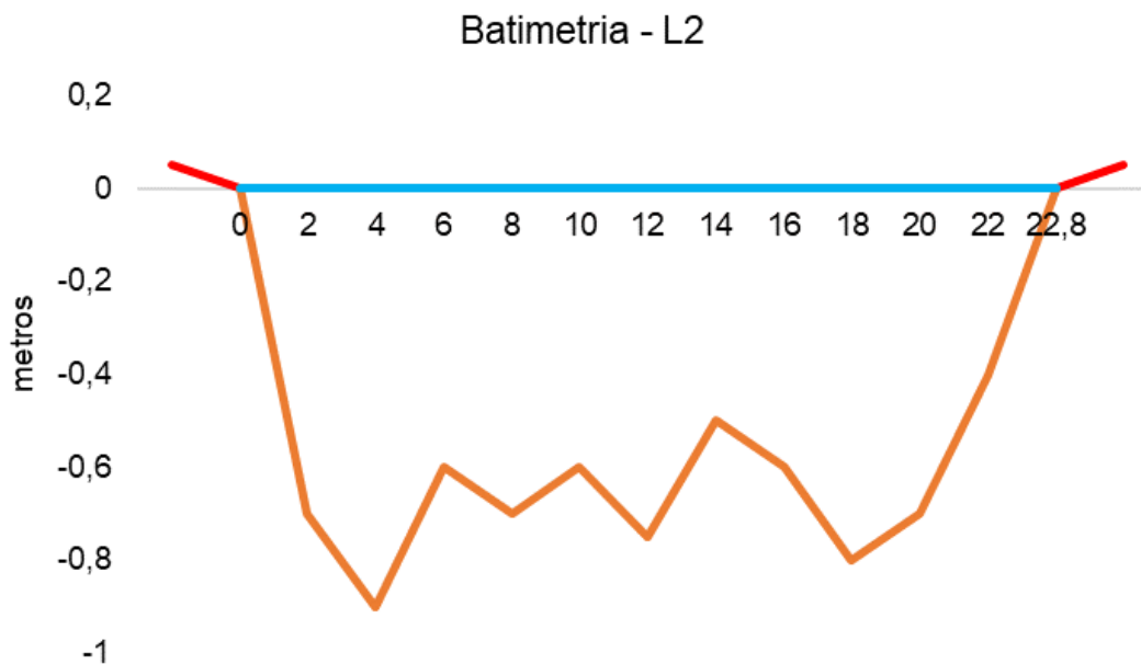
Figura V-81. Desenho esquemático da batimetria da estação L2 - Rio Macacu.
