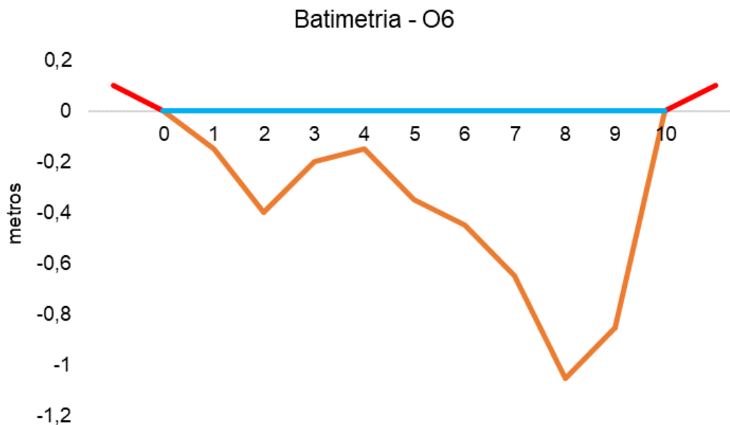
Figura V-101. Desenho esquemático da batimetria da estação O6 - Rio Sapucaia.
