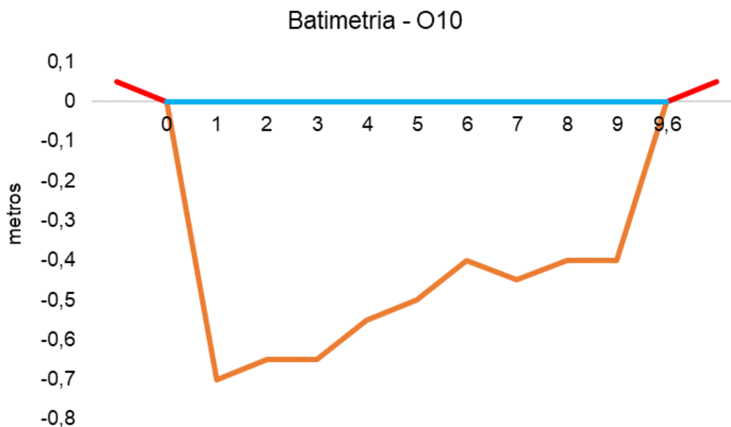
Figura V-105. Desenho esquemático da batimetria da estação O10 - Rio Iguçu.
