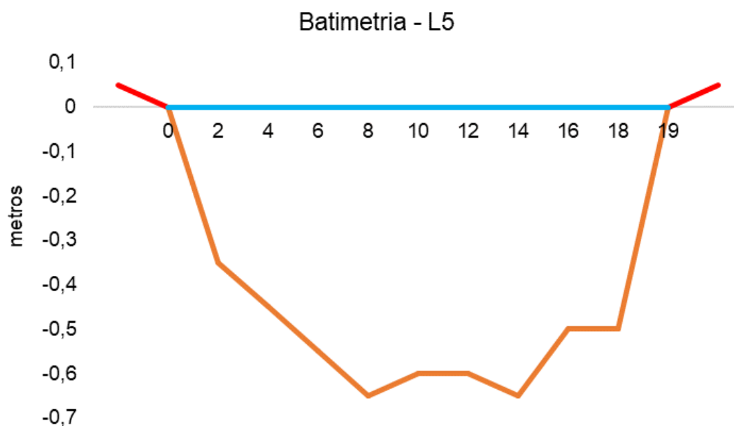
Figura V-84. Desenho esquemático da batimetria da estação L5 - Rio Macacu.
