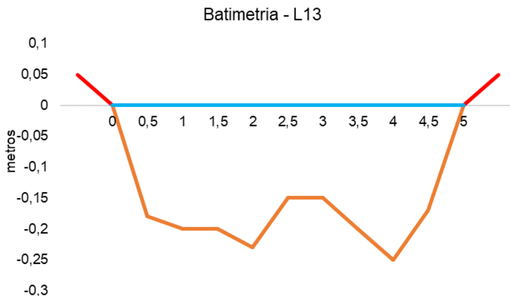
Figura V-89. Desenho esquemático da batimetria da estação L13 - Rio Itaperi.
