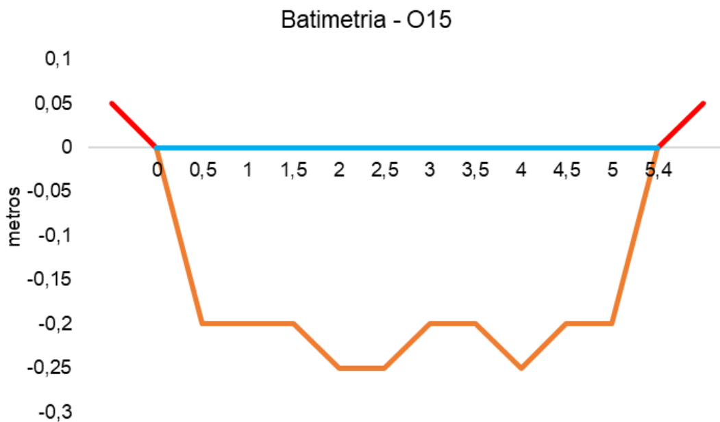
Figura V-110. Desenho esquemático da batimetria da estação O15 - Rio Sarapuí.
