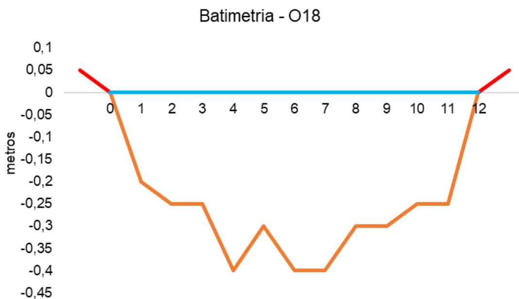
Figura V-112. Desenho esquemático da batimetria da estação O18 - Rio Acari.
