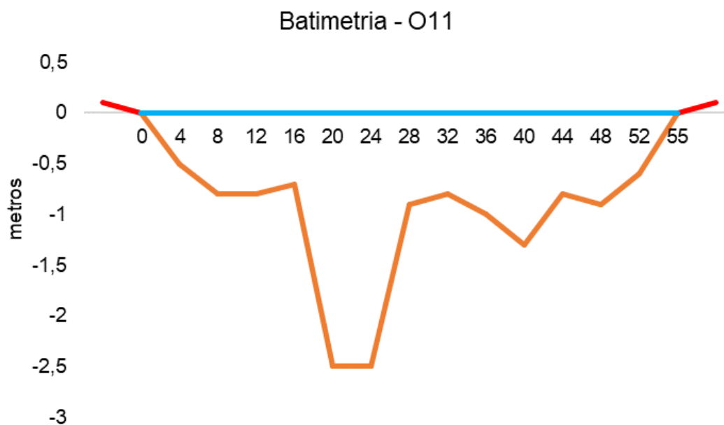
Figura V-106. Desenho esquemático da batimetria da estação O11 - Rio Iguçu.
