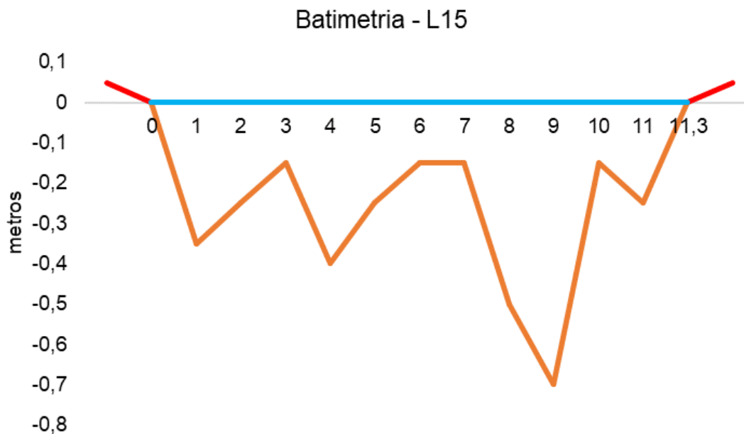
Figura V-91. Desenho esquemático da batimetria da estação L15 - Rio Guapiaçu.
