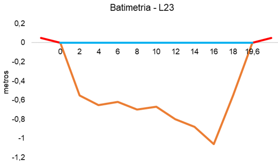
Figura V-97. Desenho esquemático da batimetria da estação L23 - Afluente do Rio Caceribu.
