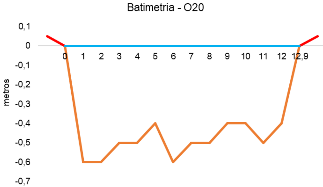
Figura V-113. Desenho esquemático da batimetria da estação O20 - Rio Acari.
