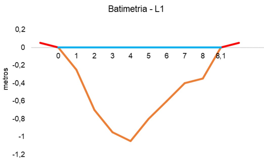
Figura V-80. Desenho esquemático da batimetria da estação L1 - Rio Macacu.
