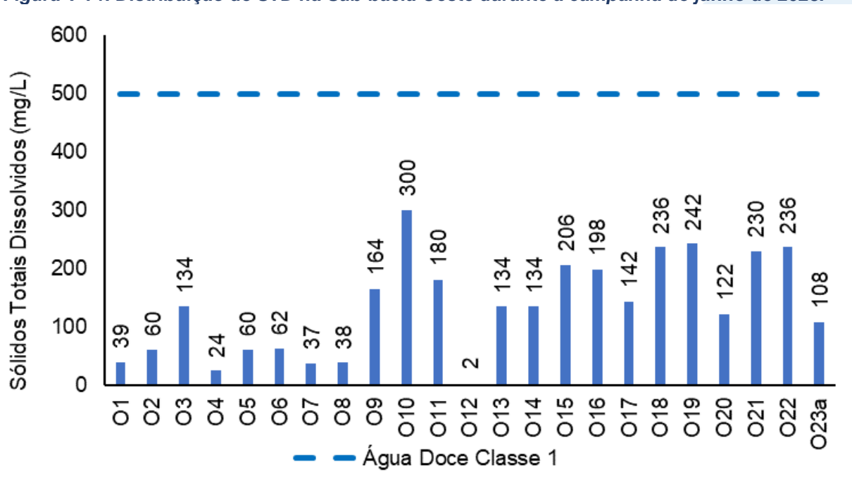
Figura V-71. Distribuição de STD na Sub-bacia Oeste durante a campanha de junho de 2023.
