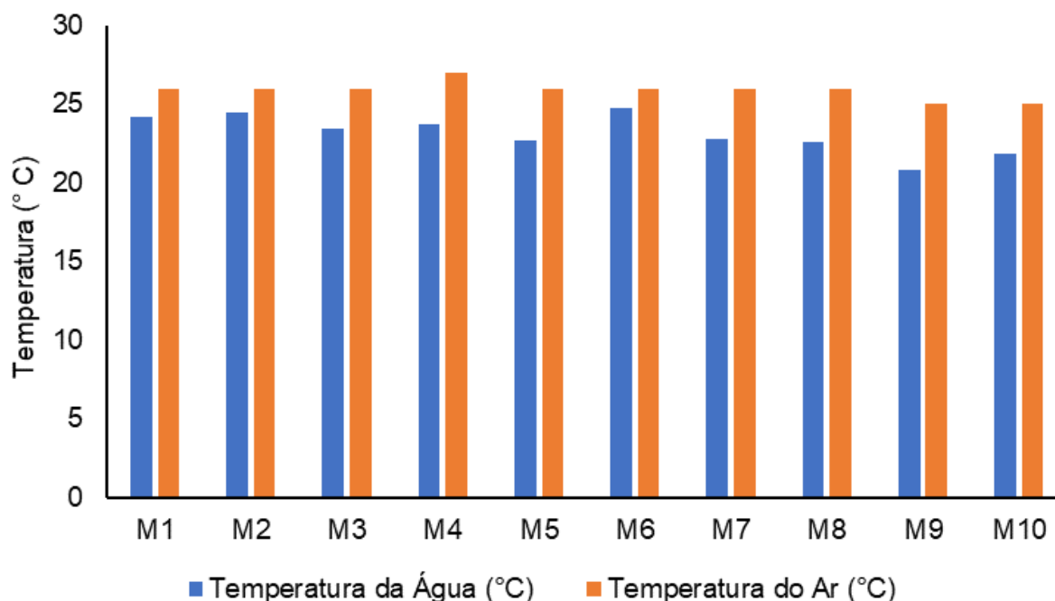
Figura V-2. Distribuição de temperatura do ar e da água na Sub-bacia do Sistema Lagunar de Maricá durante a campanha de junho de 2023.
