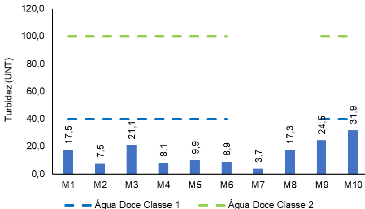
Figura V-7. Distribuição de turbidez na Sub-bacia do Sistema Lagunar de Maricá durante a campanha de junho de 2023.
