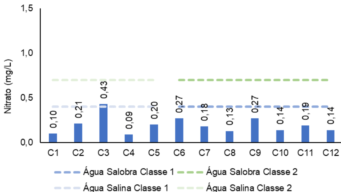
Figura V-45. Distribuição de nitrato na Sub-bacia do Sistema Lagunar Itaipu-Piratininga durante a campanha de junho de 2023.
