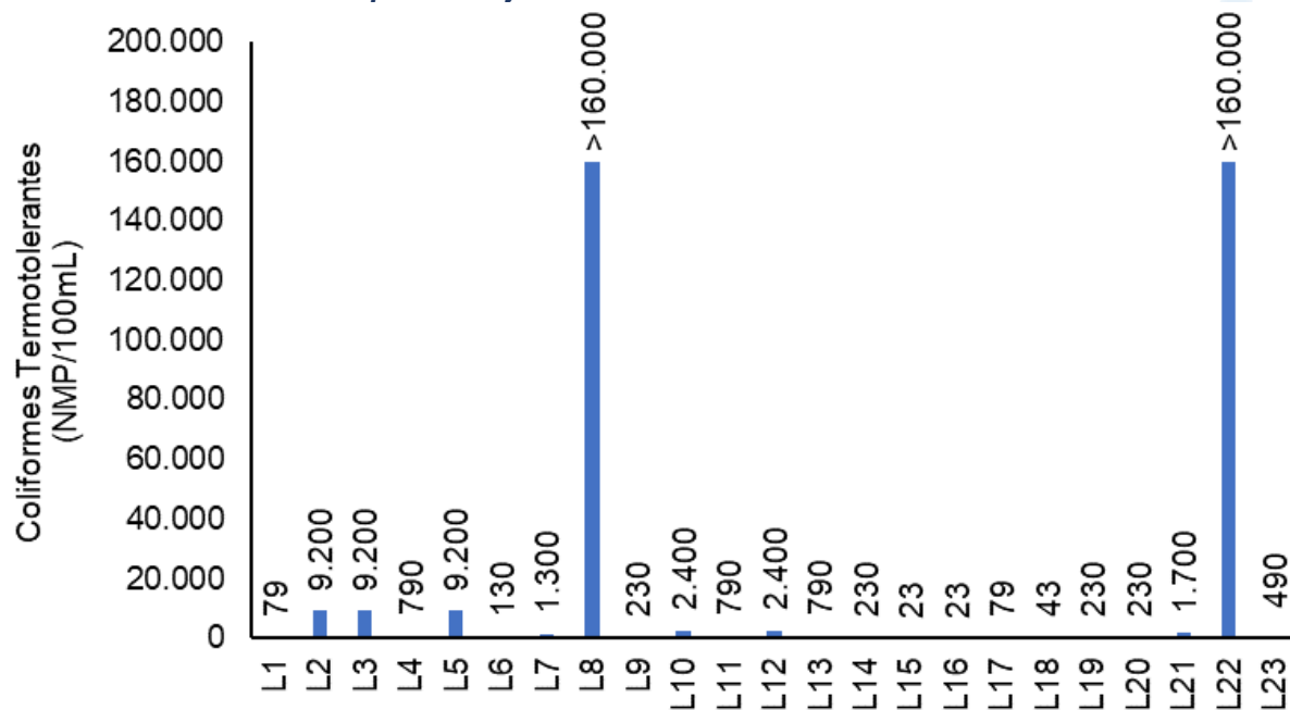
Figura V-60. Distribuição de coliformes termotolerantes na região Leste da Baía de Guanabara durante a campanha de junho de 2023.
