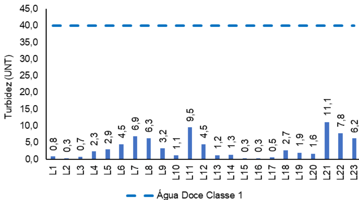
Figura V-55. Distribuição de turbidez na Sub-bacia Leste durante a campanha de junho de 2023.
