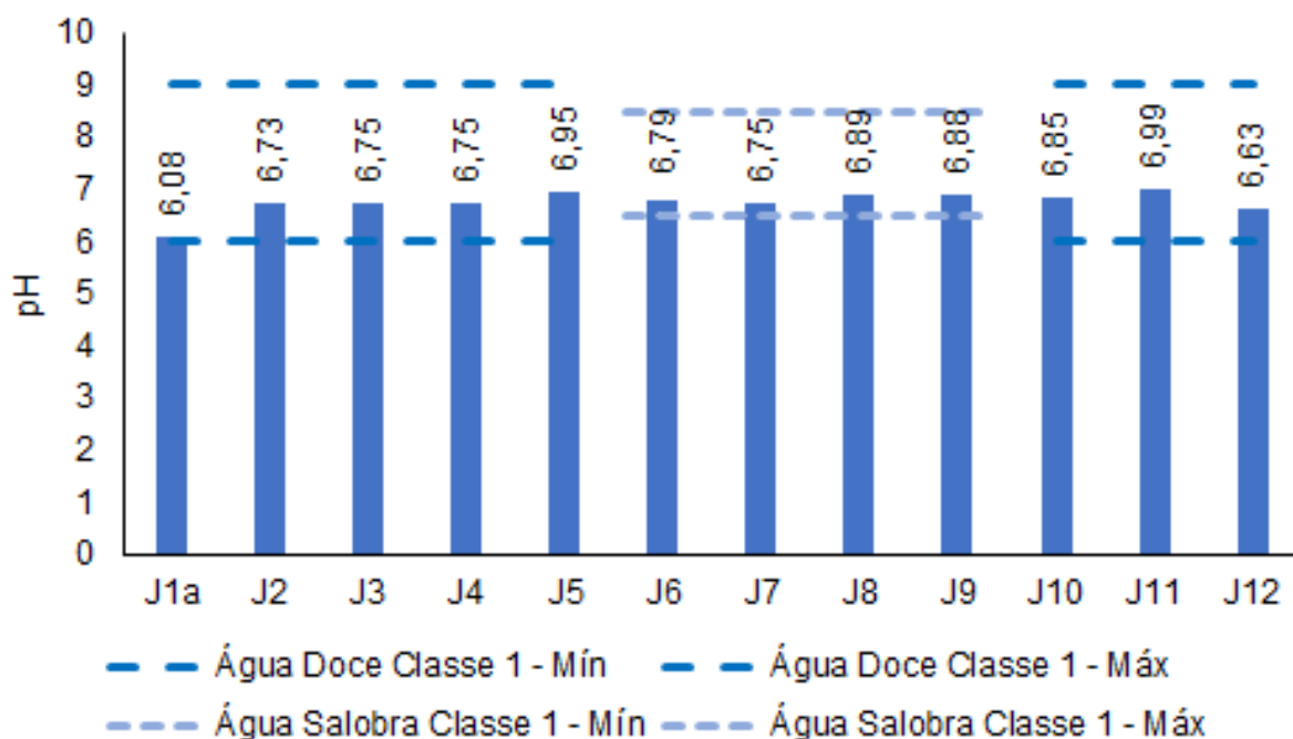
Figura V-18. Distribuição de pH na Sub-bacia do Sistema Lagunar de Jacarepaguá durante a campanha de junho de 2023.
