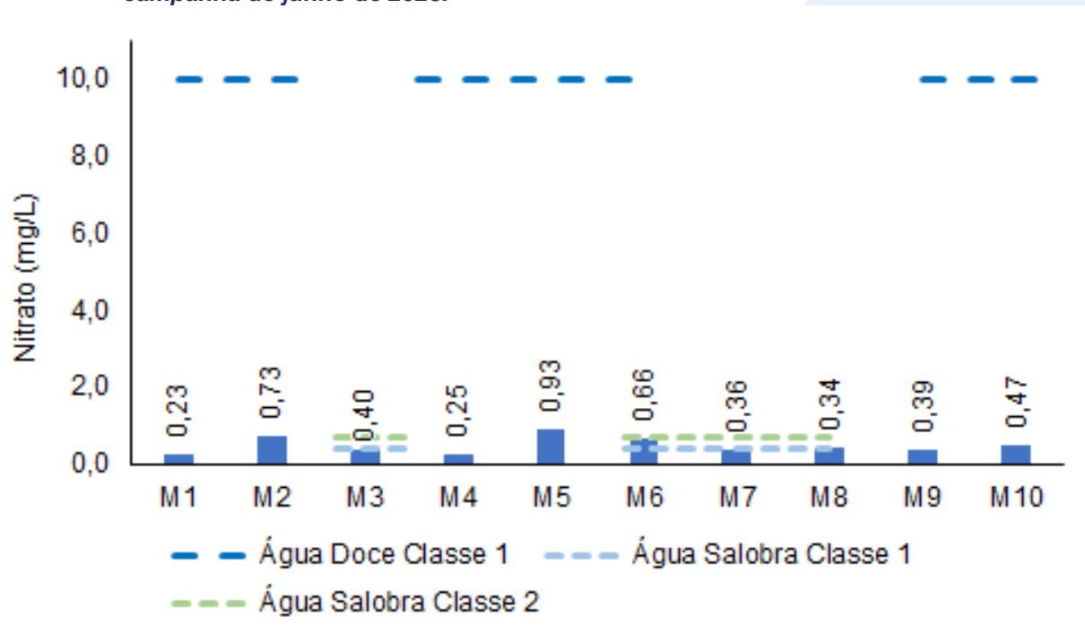
Figura V-9. Distribuição de nitrato na Sub-bacia do Sistema Lagunar de Maricá durante a campanha de junho de 2023.
