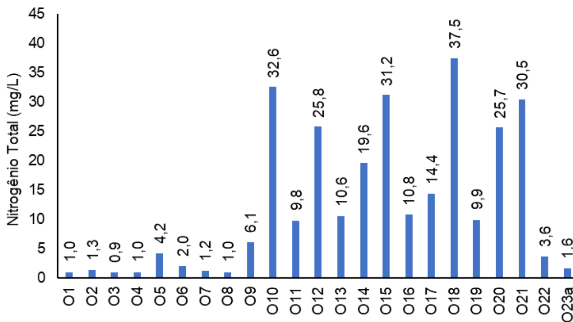
Figura V-70. Distribuição de nitrogênio total na Sub-bacia Oeste durante a campanha de junho de 2023.
