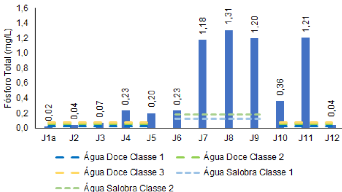
Figura V-20. Distribuição de fósforo total na Sub-bacia do Sistema Lagunar de Jacarepaguá durante a campanha de junho de 2023.
