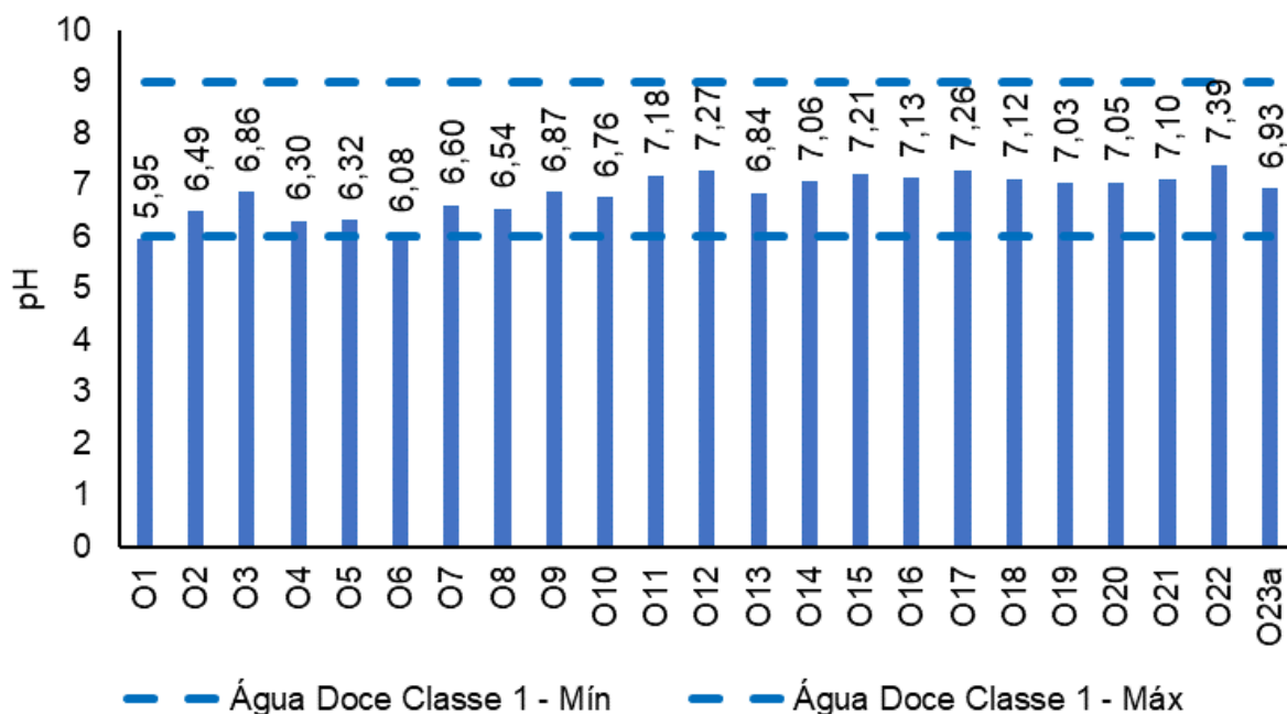
Figura V-66. Distribuição de pH na Sub-bacia Oeste durante a campanha de junho de 2023.
