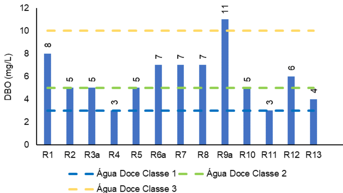
Figura V-28. Distribuição de DBO na Bacia da Lagoa Rodrigo de Freitas durante a campanha de junho de 2023.
