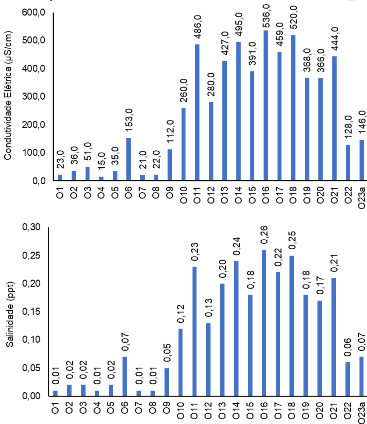
Figura V-61. Distribuição de condutividade e salinidade na Sub-bacia Oeste durante a campanha de junho de 2023.
