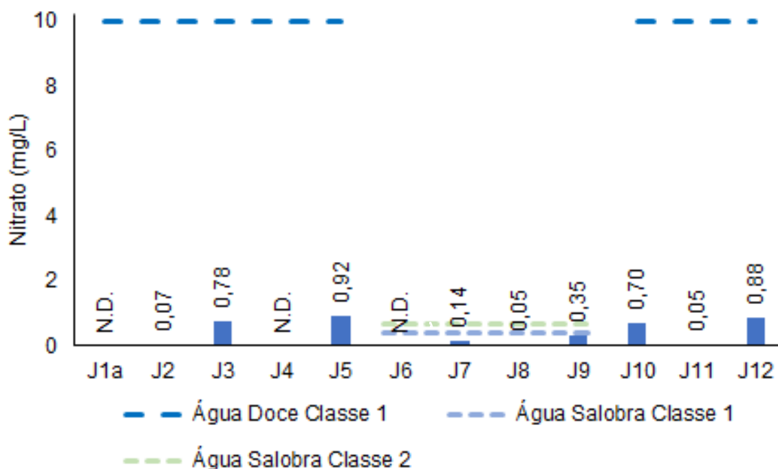
Figura V-21. Distribuição de nitrato na Sub-bacia do Sistema Lagunar de Jacarepaguá durante a campanha de junho de 2023.
