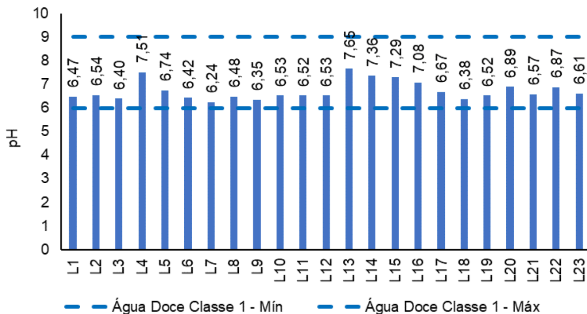
Figura V-54. Distribuição de pH na Sub-bacia Leste durante a campanha de junho de 2023.
