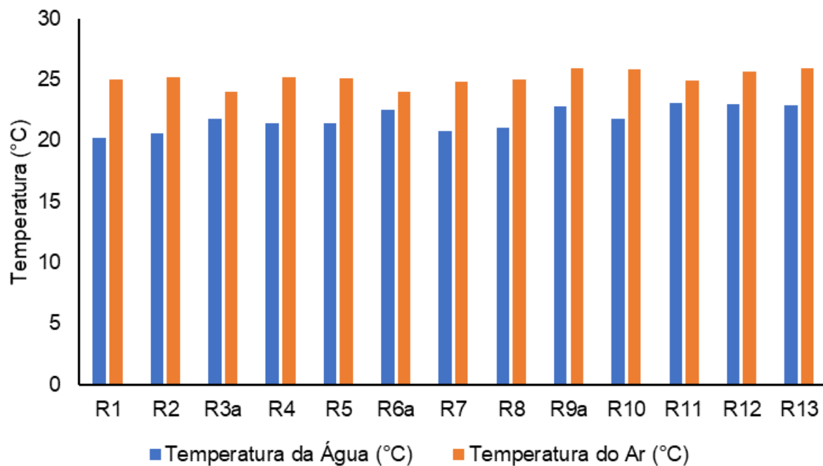
Figura V-26. Distribuição de temperatura do ar e da água na Bacia da Lagoa Rodrigo de Freitas durante a campanha de junho de 2023.
