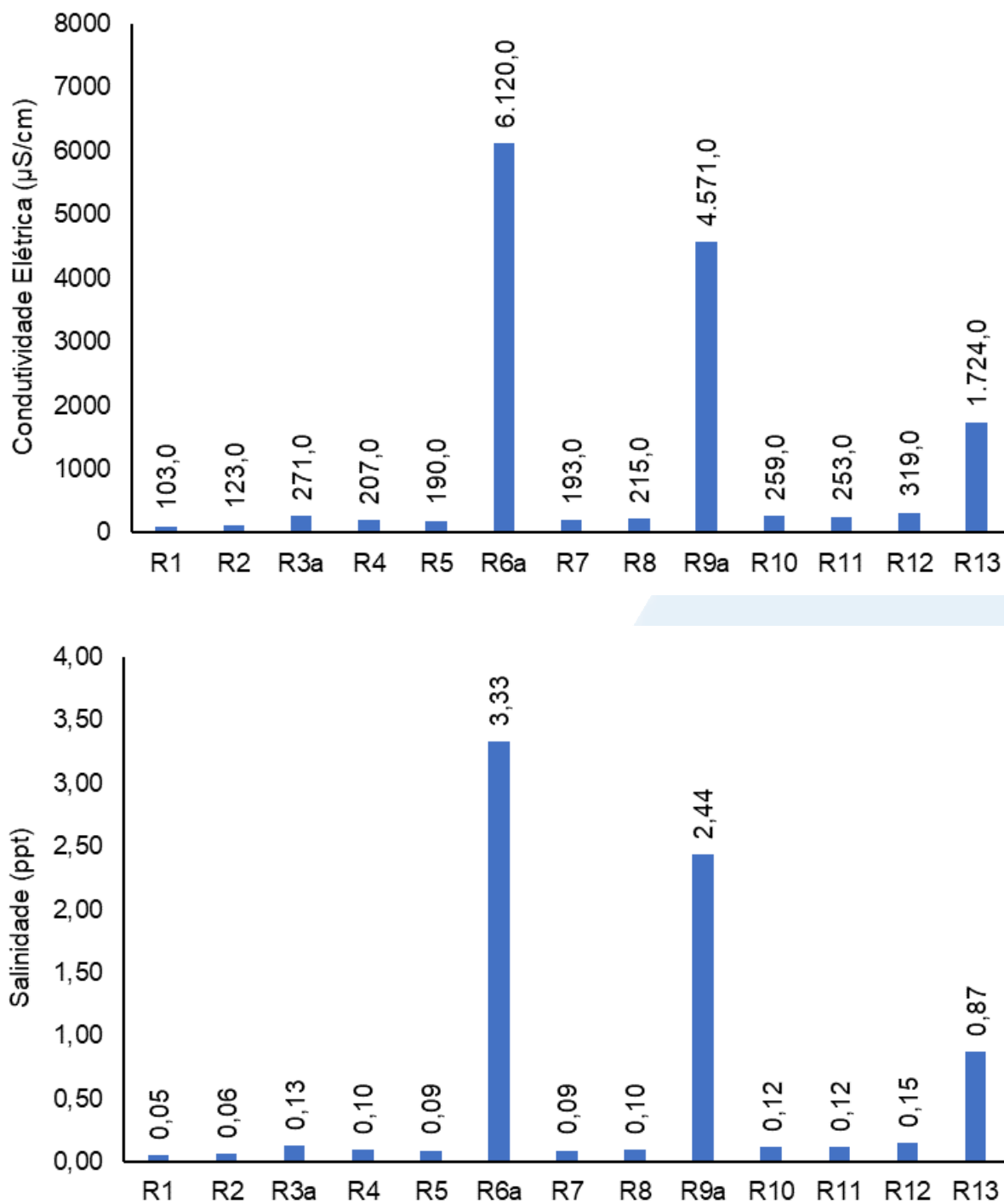
Figura V-25. Distribuição de condutividade e salinidade na Bacia da Lagoa Rodrigo de Freitas durante a campanha de junho de 2023.
