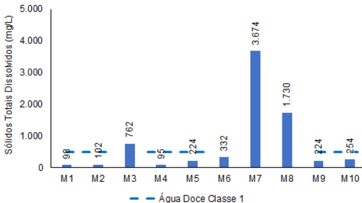
Figura V-11. Distribuição de STD na Sub-bacia do Sistema Lagunar de Maricá durante a campanha de junho de 2023.
