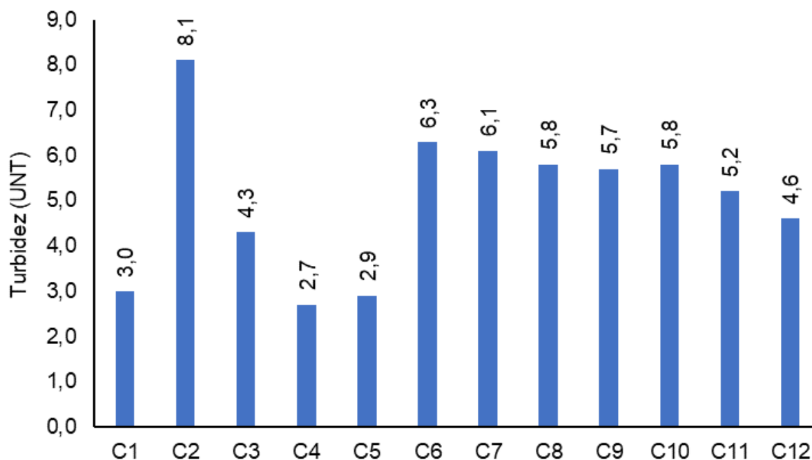
Figura V-43. Distribuição de turbidez na Sub-bacia do Sistema Lagunar Itaipu-Piratininga durante a campanha de junho de 2023.
