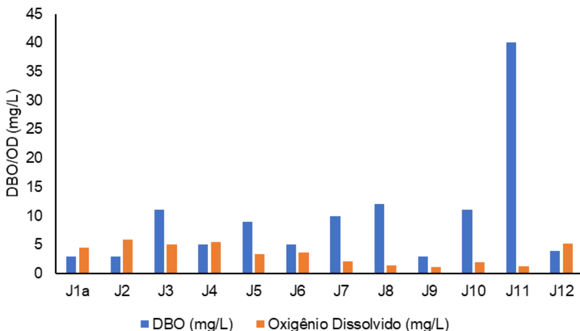
Figura V-17. Comparativo entre disponibilidade de OD e DBO na Sub-bacia do Sistema Lagunar de Jacarepaguá durante a campanha de junho de 2023.
