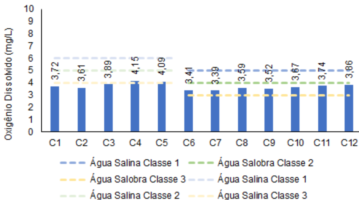
Figura V-39. Distribuição de oxigênio dissolvido na Sub-bacia do Sistema Lagunar Itaipu-Piratininga durante a campanha de junho de 2023.
