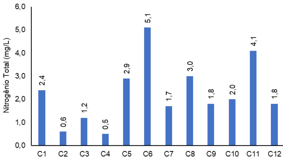
Figura V-46. Distribuição de nitrogênio total na Sub-bacia do Sistema Lagunar Itaipu-Piratininga durante a campanha de junho de 2023.
