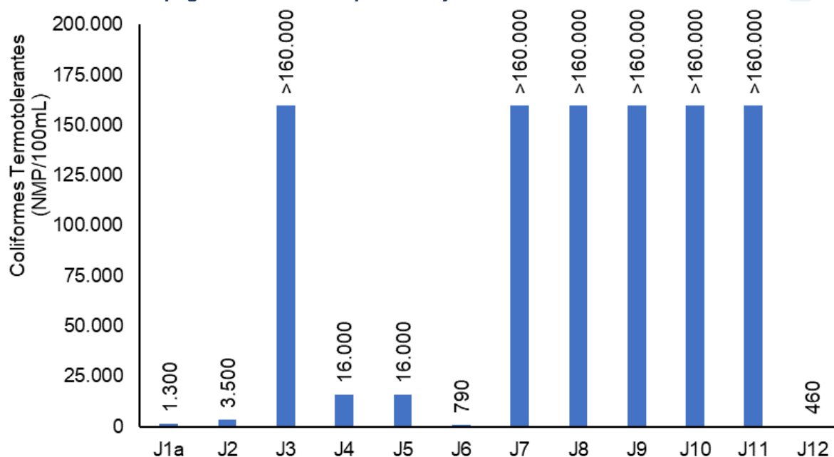
Figura V-24. Distribuição de coliformes termotolerantes na Sub-bacia do Sistema Lagunar de Jacarepaguá durante a campanha de junho de 2023.
