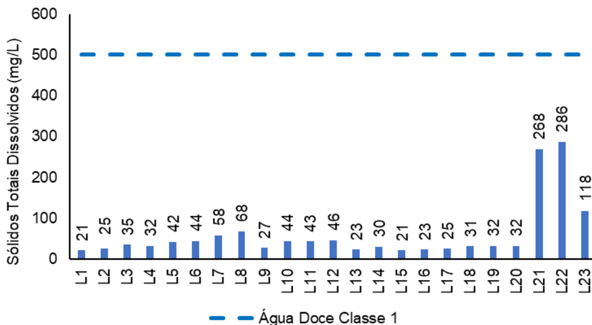
Figura V-59. Distribuição de STD na Sub-bacia Leste durante a campanha de junho de 2023.
