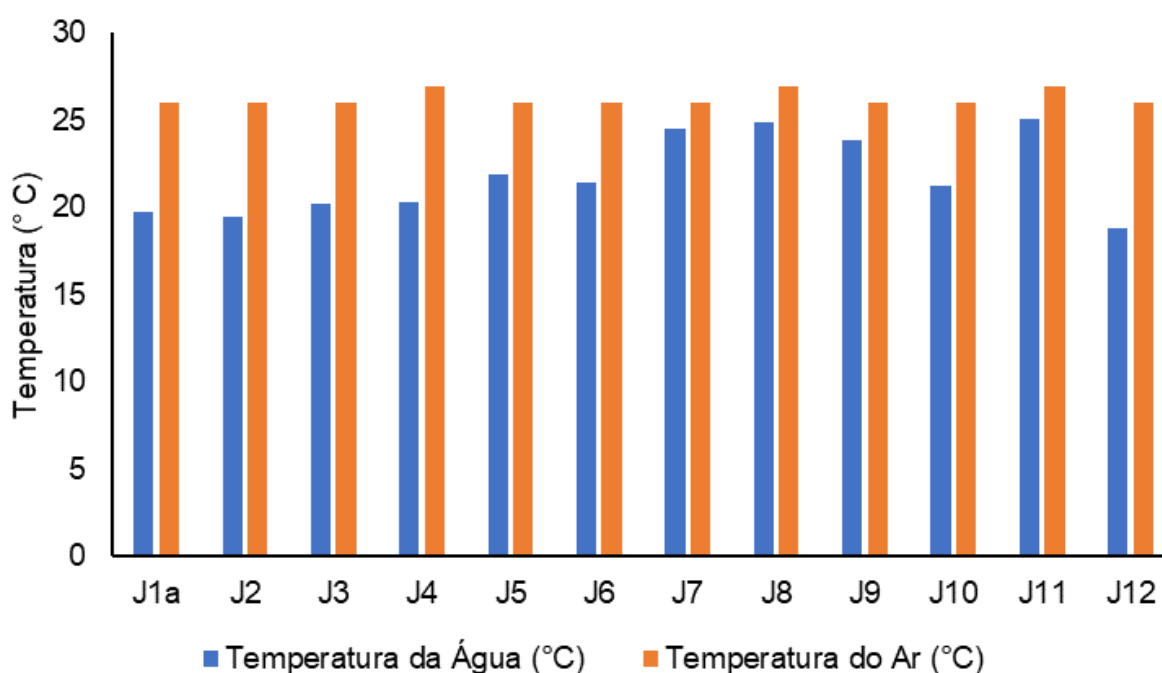
Figura V-14. Distribuição de temperatura do ar e da água na Sub-bacia do Sistema Lagunar de Jacarepaguá durante a campanha de junho de 2023.
