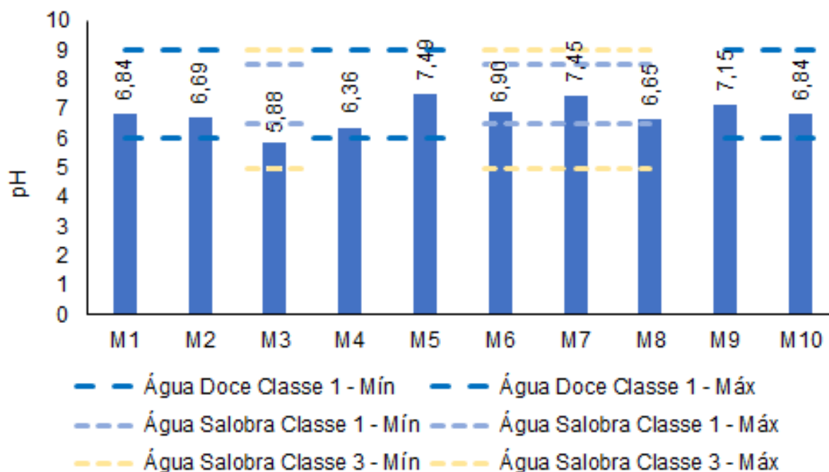
Figura V-6. Distribuição de pH na Sub-bacia do Sistema Lagunar de Maricá durante a campanha de junho de 2023.
