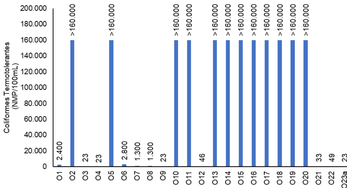
Figura V-72. Distribuição de coliformes termotolerantes na região Oeste durante a campanha de junho de 2023.
