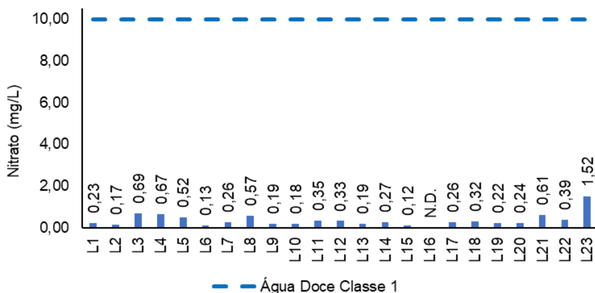
Figura V-57. Distribuição de nitrato na região Leste da Baía de Guanabara durante a campanha de junho de 2023.
