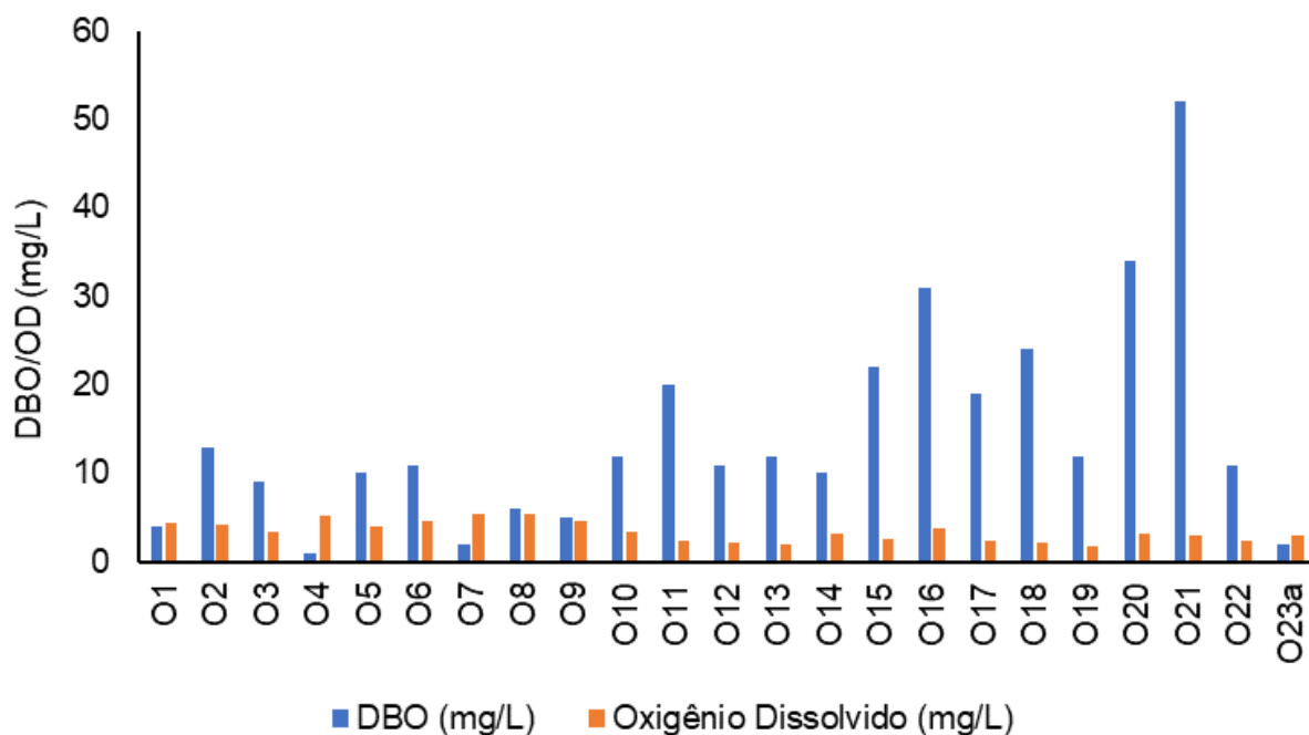
Figura V-65. Comparativo de OD e DBO na Sub-bacia Oeste durante a campanha de junho de 2023.
