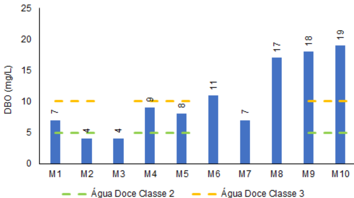
Figura V-4. Distribuição de DBO na Sub-bacia do Sistema Lagunar de Maricá durante a campanha de junho de 2023.
