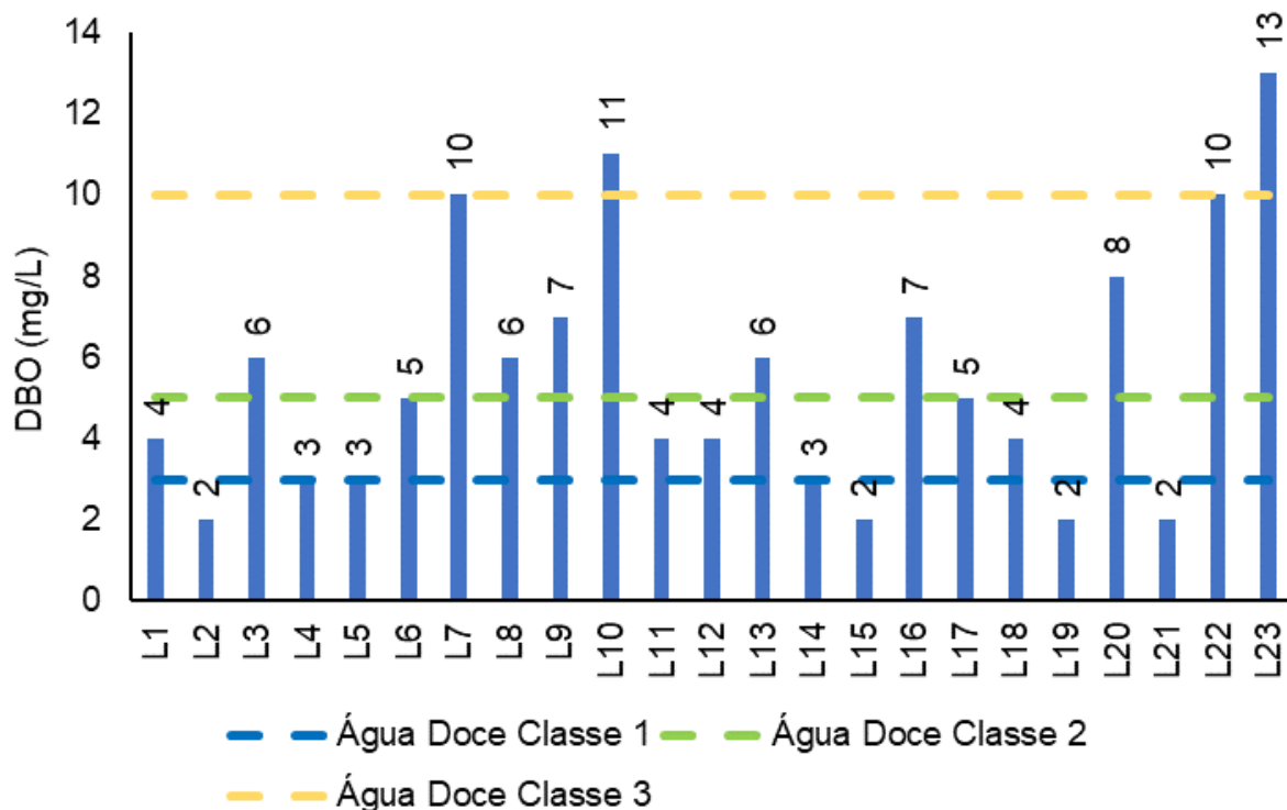
Figura V-52. Distribuição de DBO na Sub-bacia Leste durante a campanha de junho de 2023.
