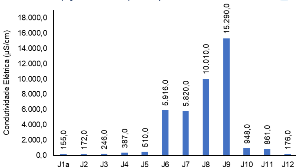
Figura V-13. Distribuição de condutividade e salinidade na Sub-bacia do Sistema Lagunar de Jacarepaguá durante a campanha de junho de 2023.
