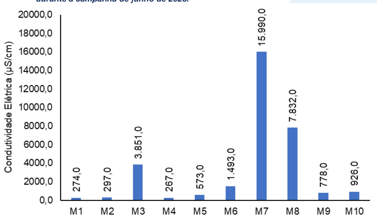
Figura V-1. Distribuição de condutividade e salinidade na Sub-bacia do Sistema Lagunar de Maricá durante a campanha de junho de 2023.
