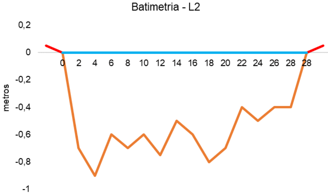
Figura V-79. Desenho esquemático da batimetria da estação L2 - Rio Macacu.
