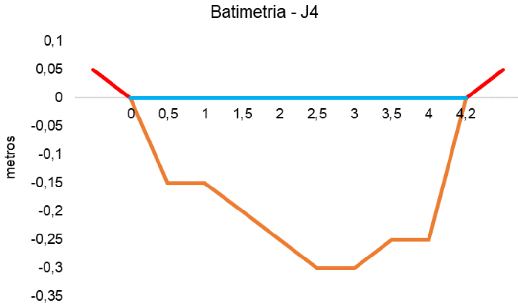
Figura V-74. Desenho esquemático da batimetria da estação J4 - Canal de Sernambetiba.
