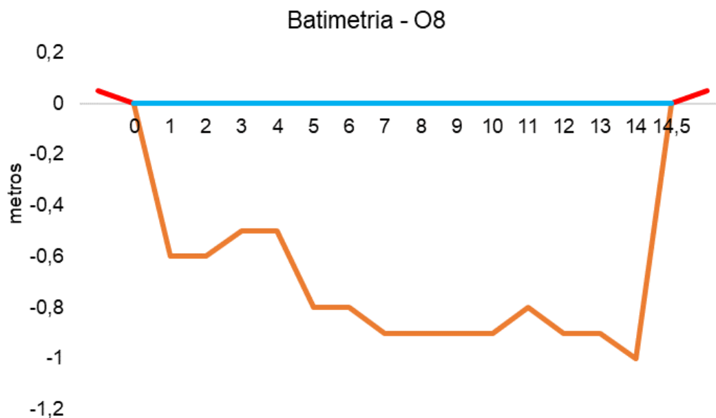
Figura V-100. Desenho esquemático da batimetria da estação O8 - Rio Tinguá.
