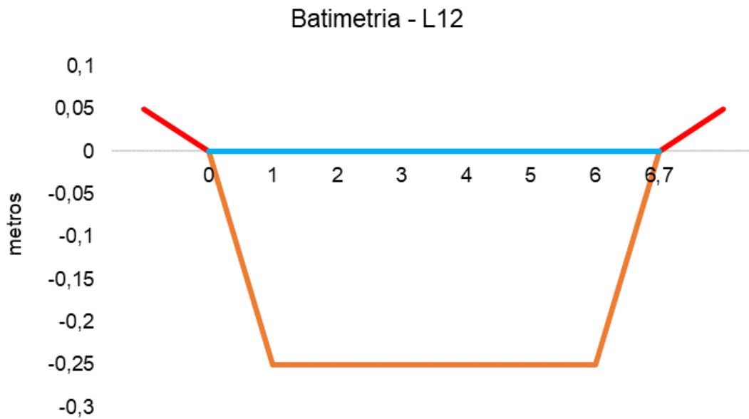
Figura V-86. Desenho esquemático da batimetria da estação L12 - Rio Rabelo.
