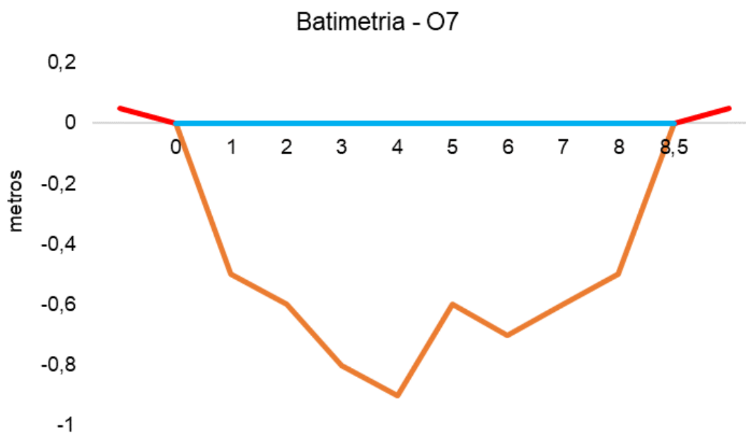
Figura V-99. Desenho esquemático da batimetria da estação O7 - Rio Tinguá.
