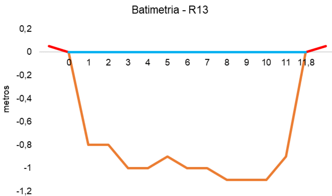
Figura V-77. Desenho esquemático da batimetria da estação R13 - Rio Rainha.
