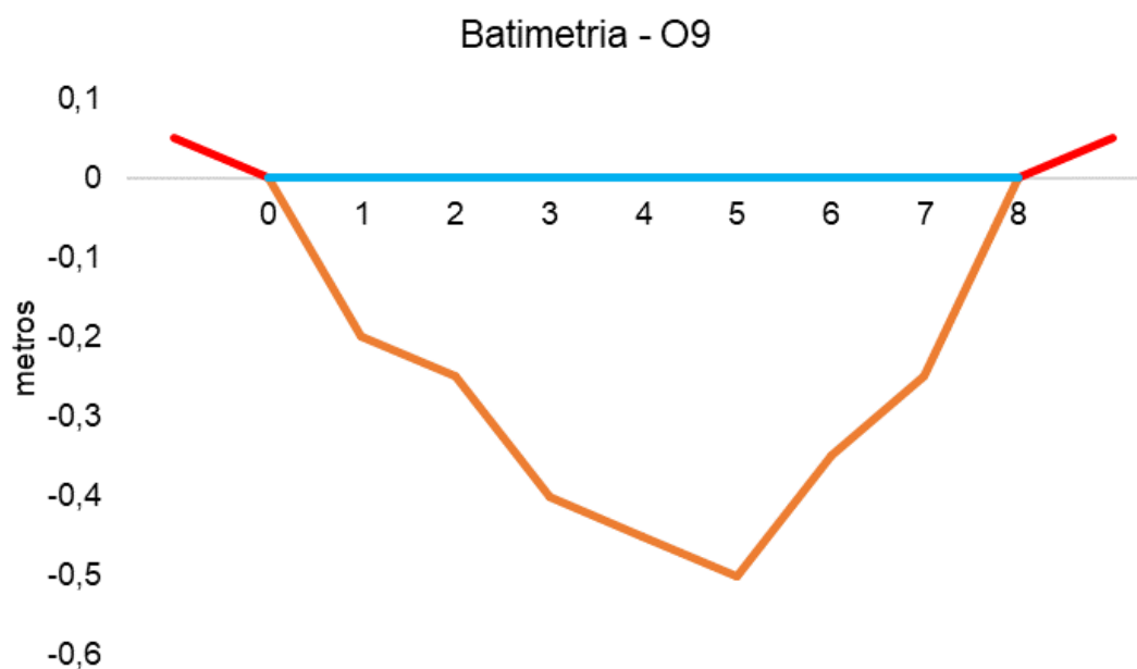
Figura V-101. Desenho esquemático da batimetria da estação O9 - Rio Iguaçu.
