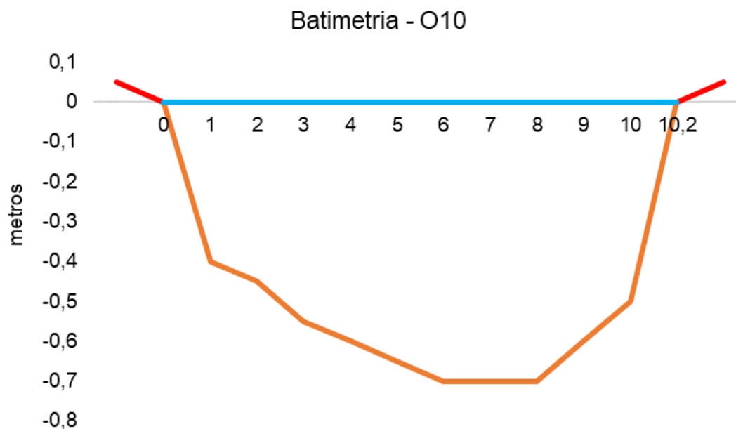
Figura V-102. Desenho esquemático da batimetria da estação O10 - Rio Iguaçu.
