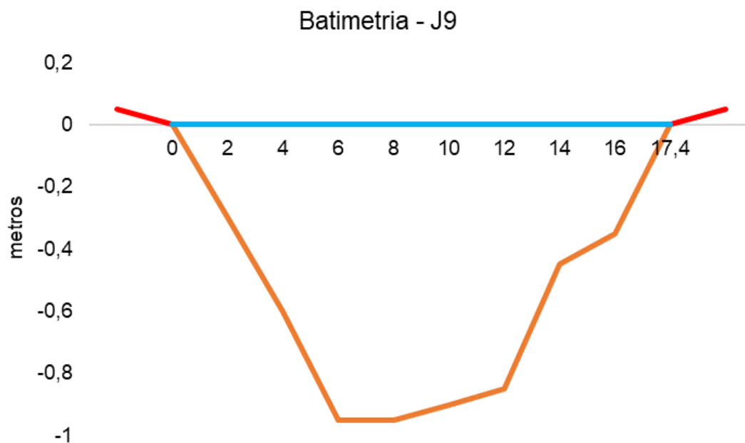
Figura V-76. Desenho esquemático da batimetria da estação J9 - Canal das Taxas.
