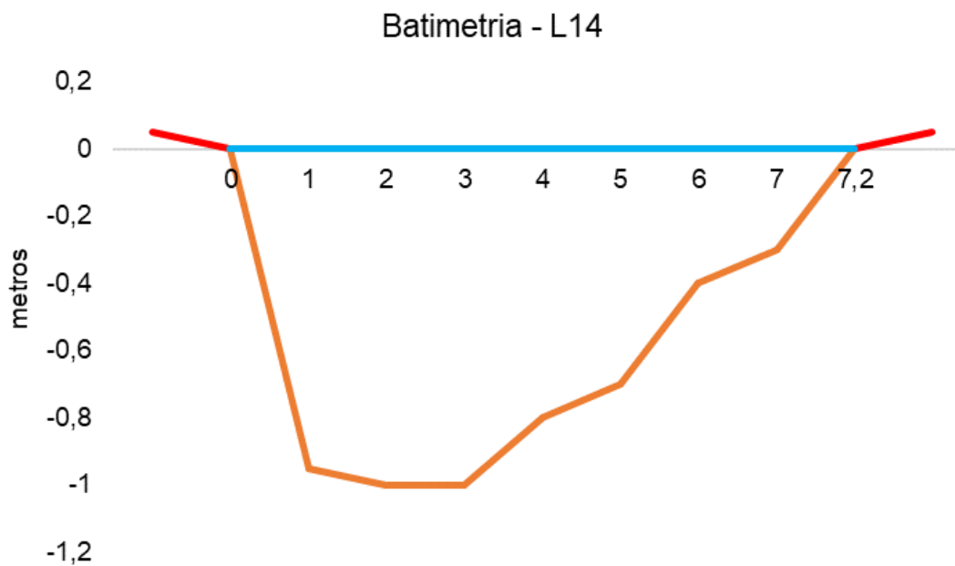
Figura V-88. Desenho esquemático da batimetria da estação L14 - Rio Duas Barras.
