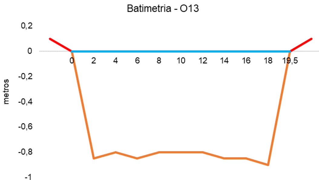
Figura V-105. Desenho esquemático da batimetria da estação O13 - Rio Botas.
