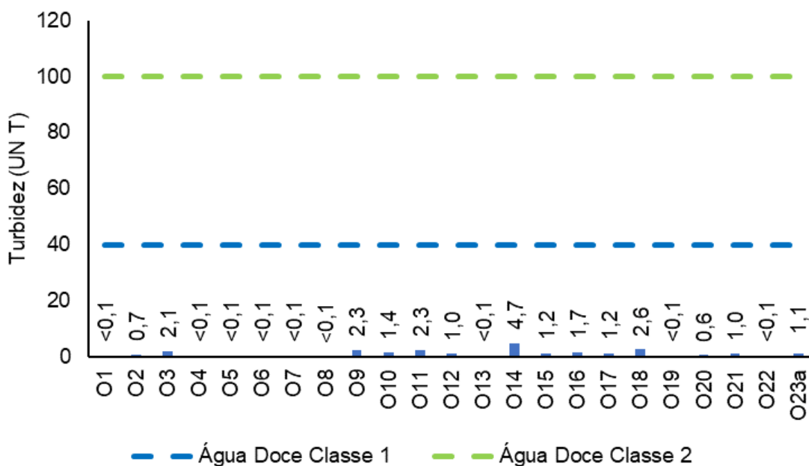
Figura V-67. Distribuição de turbidez na Sub-bacia Oeste durante a campanha de maio de 2023.
