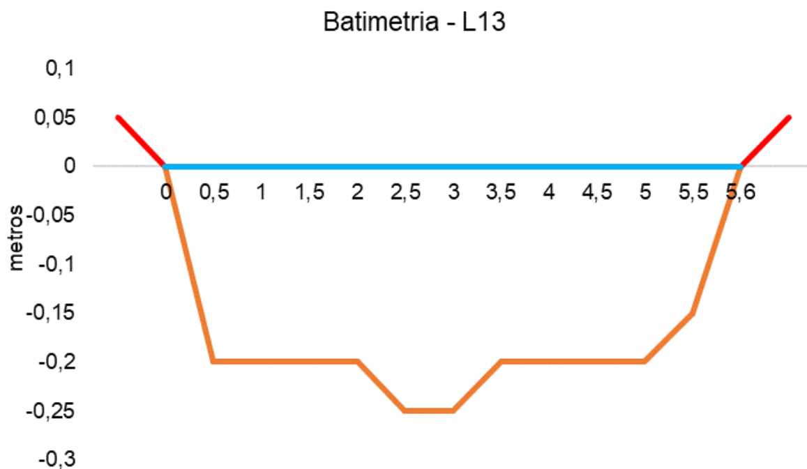
Figura V-87. Desenho esquemático da batimetria da estação L13 - Rio Itaperi.
