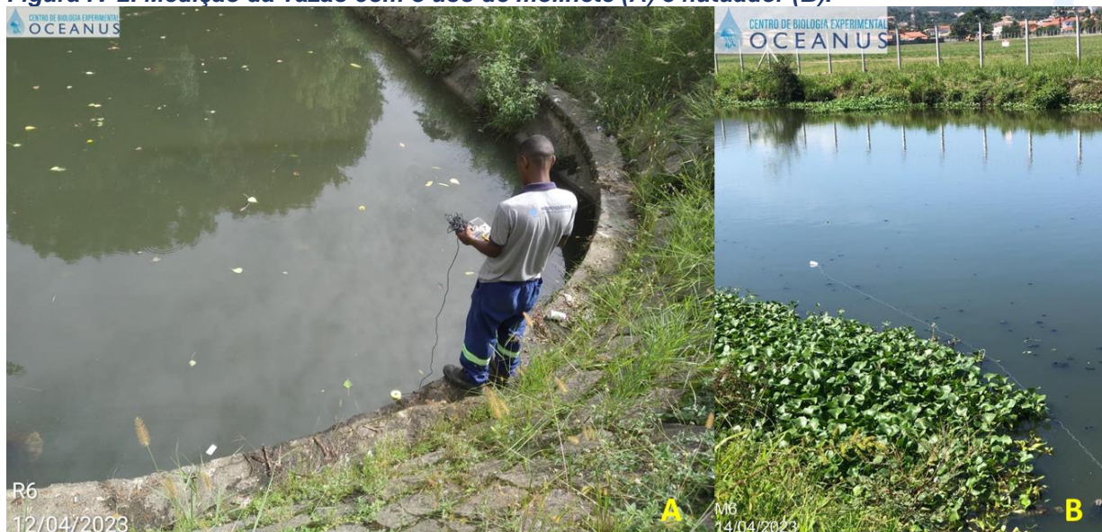
Figura IV-2. Medição da vazão com o uso de molinete (A) e flutuador (B).
