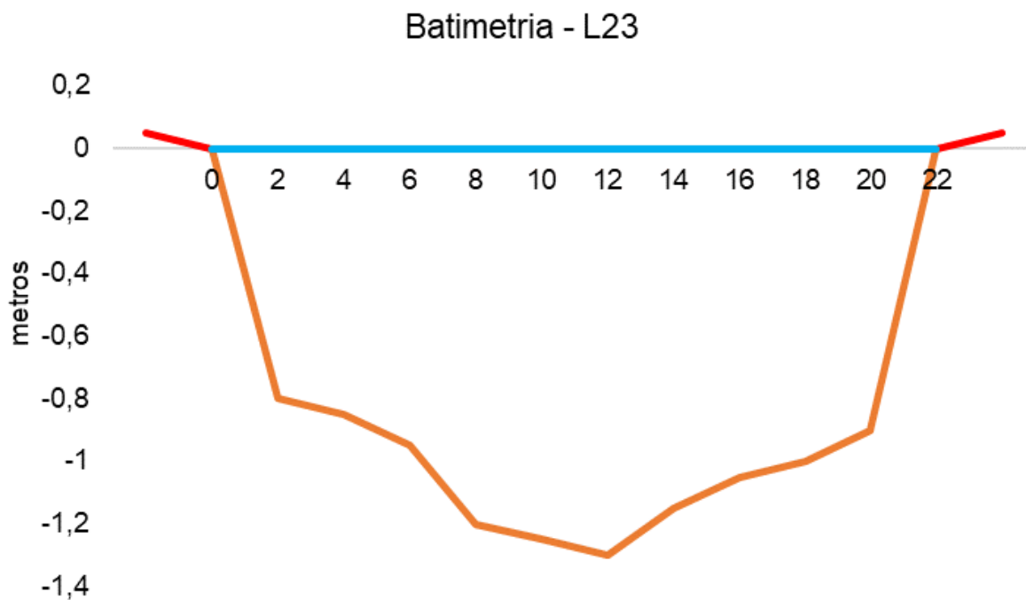
Figura V-95. Desenho esquemático da batimetria da estação L23 - Afluente do Rio Caceribu.
