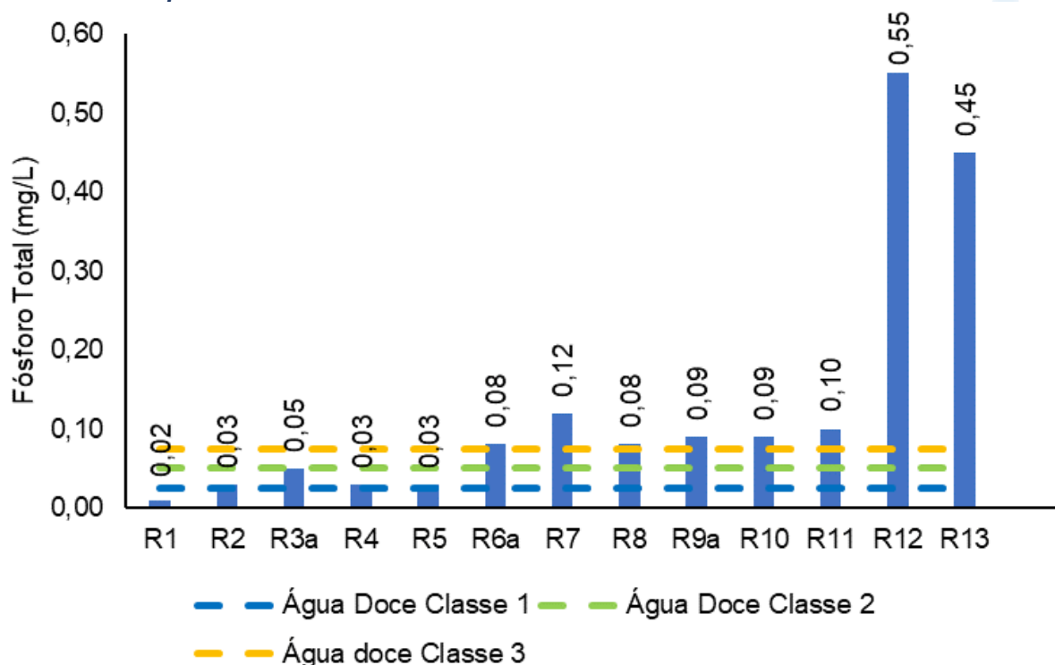
Figura V-32. Distribuição de fósforo total na Bacia da Lagoa Rodrigo de Freitas durante a campanha de abril de 2023.
