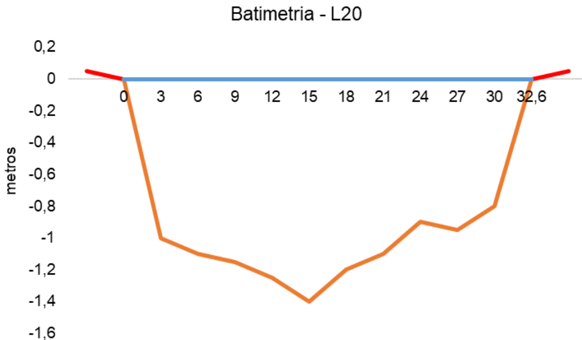
Figura V-93. Desenho esquemático da batimetria da estação L20 - Rio Guapiaçu.
