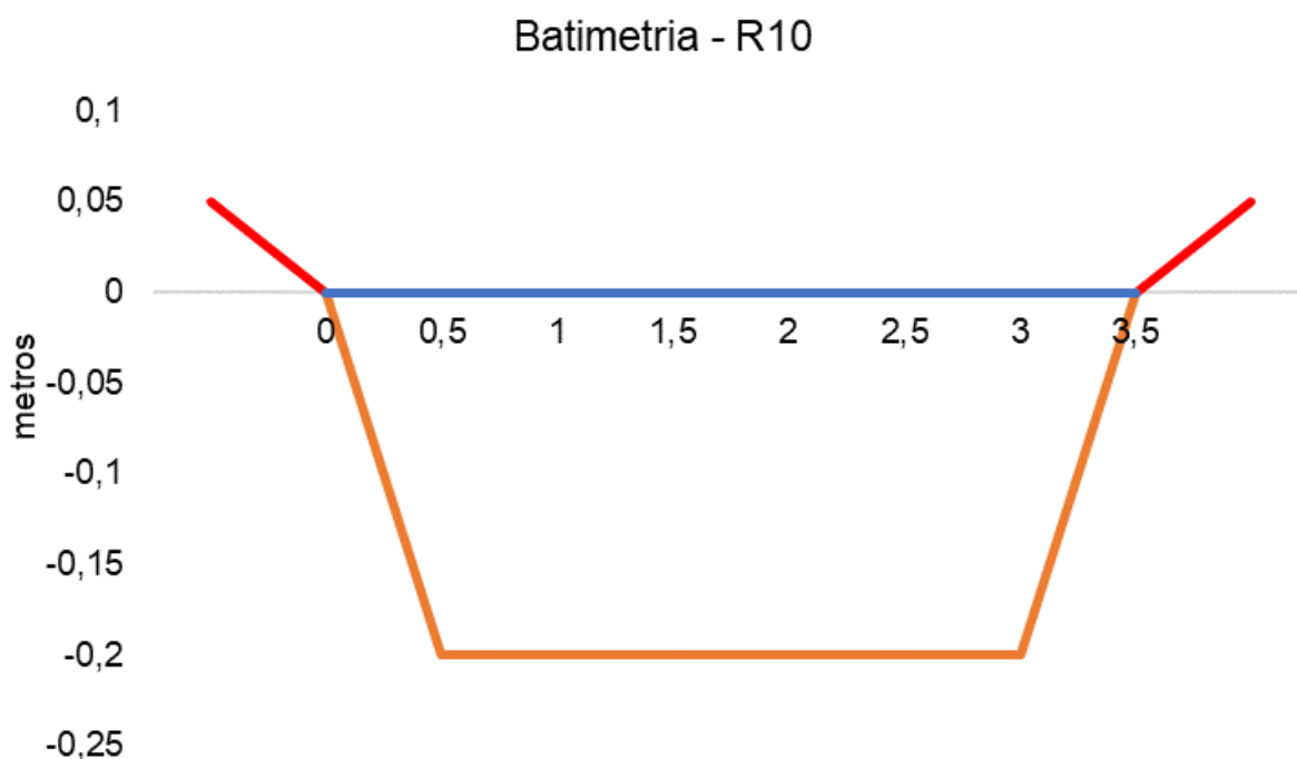
Figura V-76. Desenho esquemático da batimetria da estação R10 - Rio Rainha.
