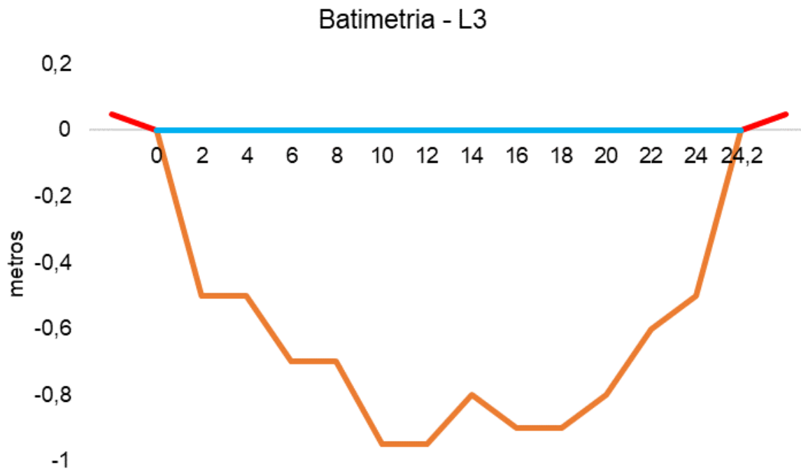
Figura V-80. Desenho esquemático da batimetria da estação L3 - Rio Macacu.
