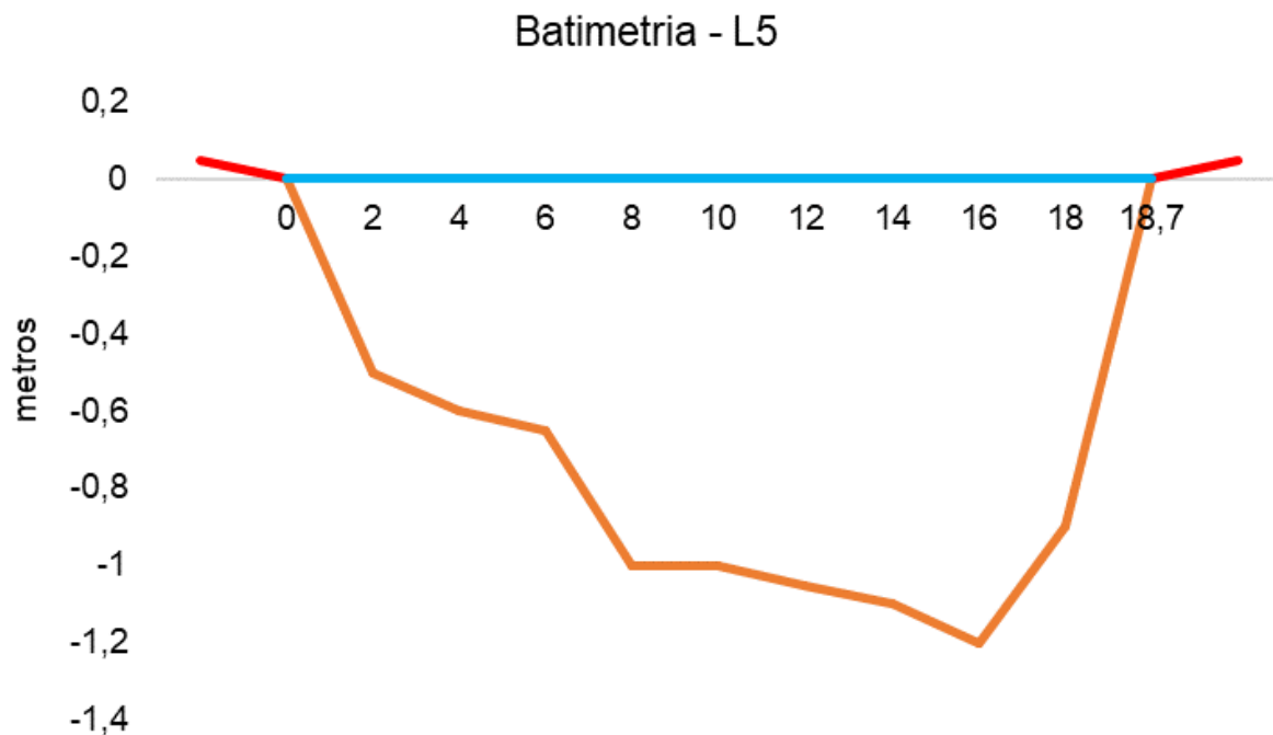
Figura V-82. Desenho esquemático da batimetria da estação L5 - Rio Macacu.
