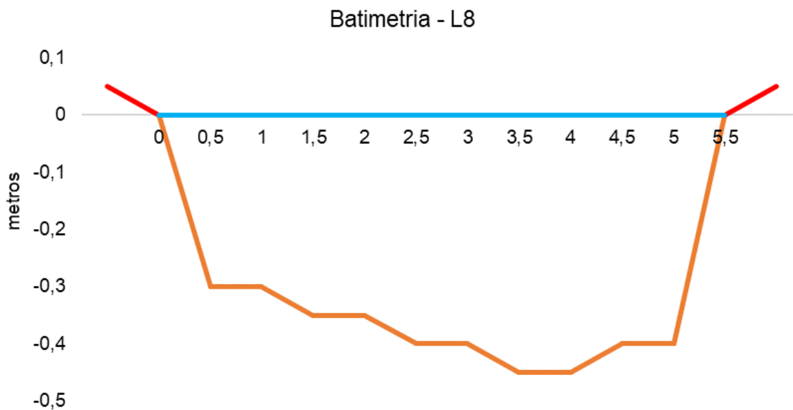
Figura V-84. Desenho esquemático da batimetria da estação L8 - Papucainha.
