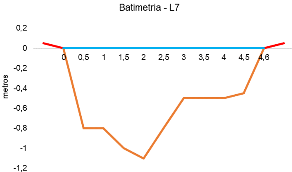
Figura V-83. Desenho esquemático da batimetria da estação L7 - Rio Cassiano.
