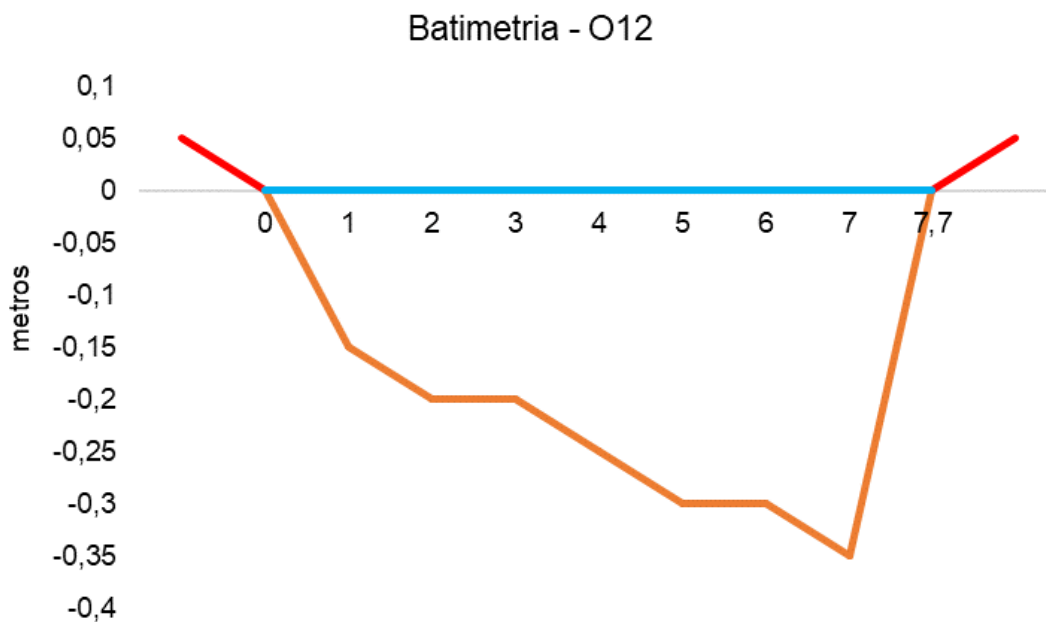
Figura V-105. Desenho esquemático da batimetria da estação O12 - Rio Botas.
