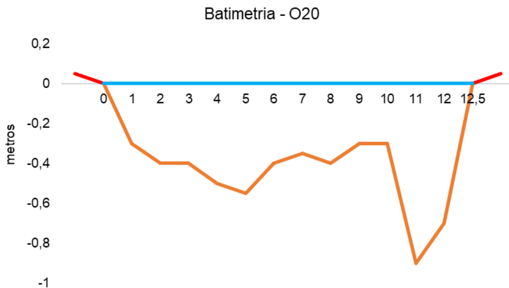
Figura V-111. Desenho esquemático da batimetria da estação O20 - Rio Acari.
