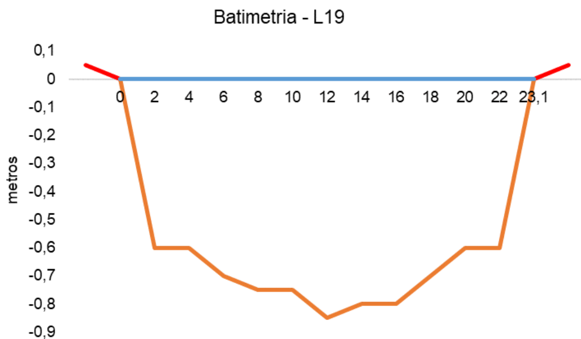
Figura V-92. Desenho esquemático da batimetria da estação L19 - Rio Guapiaçu.
