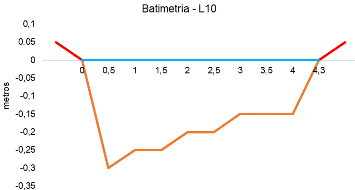
Figura V-85. Desenho esquemático da batimetria da estação L10 - Rio Rabelo.
