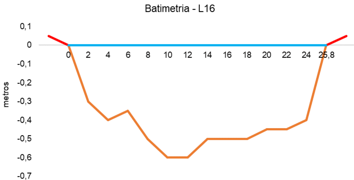
Figura V-90. Desenho esquemático da batimetria da estação L16 - Rio Guapiaçu.
