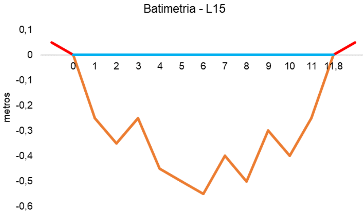
Figura V-89. Desenho esquemático da batimetria da estação L15 - Rio Guapiaçu.
