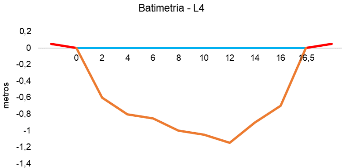
Figura V-81. Desenho esquemático da batimetria da estação L4 - Rio Macacu.
