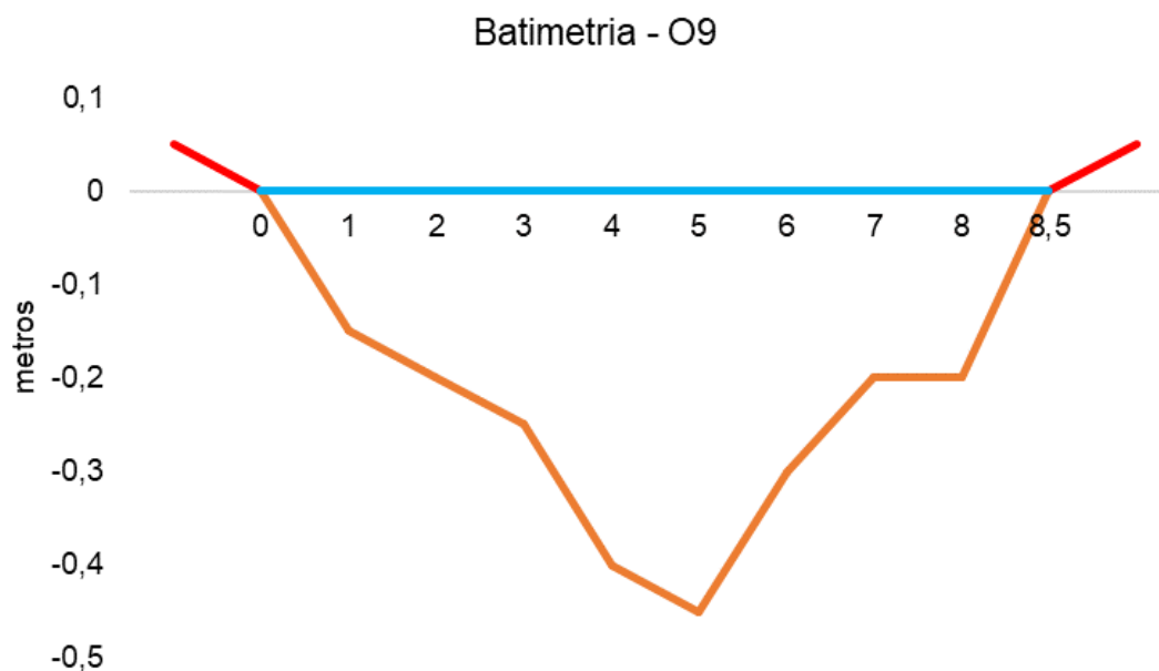
Figura V-102. Desenho esquemático da batimetria da estação O9 - Rio Iguçu.
