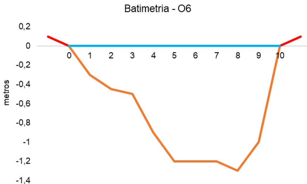
Figura V-99. Desenho esquemático da batimetria da estação O6 - Rio Sapucaia.
