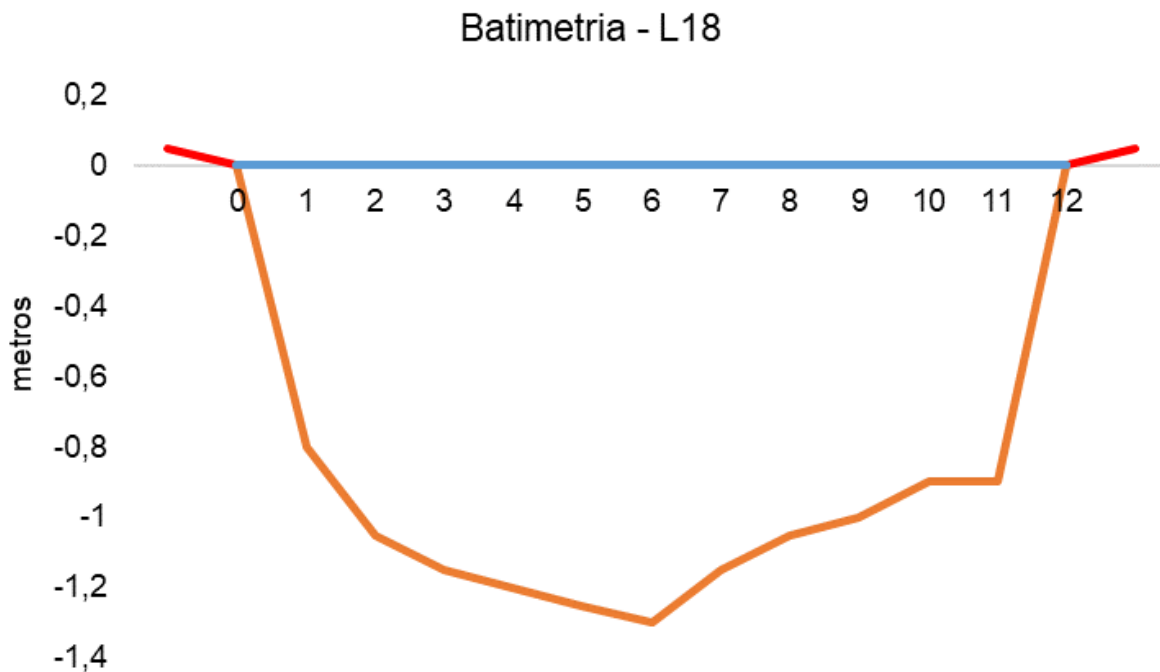
Figura V-91. Desenho esquemático da batimetria da estação L18 - Rio Guapiaçu.
