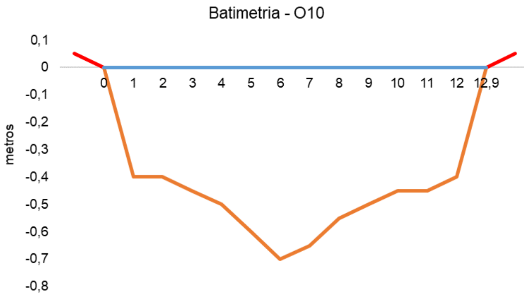
Figura V-103. Desenho esquemático da batimetria da estação O10 - Rio Iguaçu.
