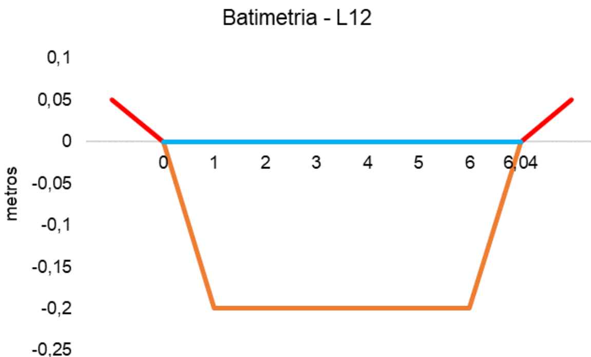
Figura V-86. Desenho esquemático da batimetria da estação L12 - Rio Rabelo.
