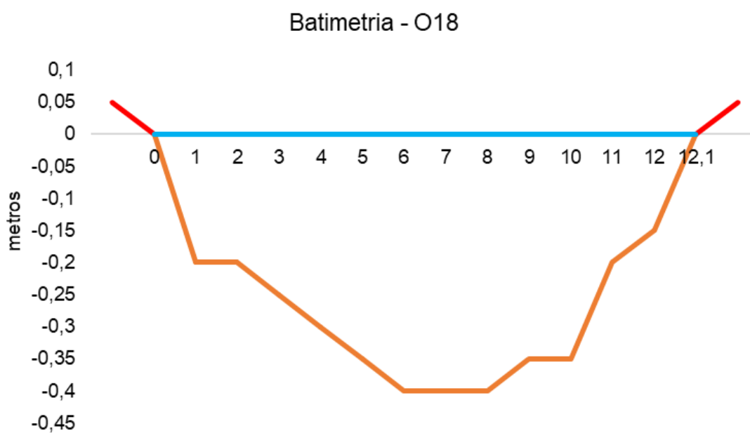
Figura V-110. Desenho esquemático da batimetria da estação O18 - Rio Acari.
